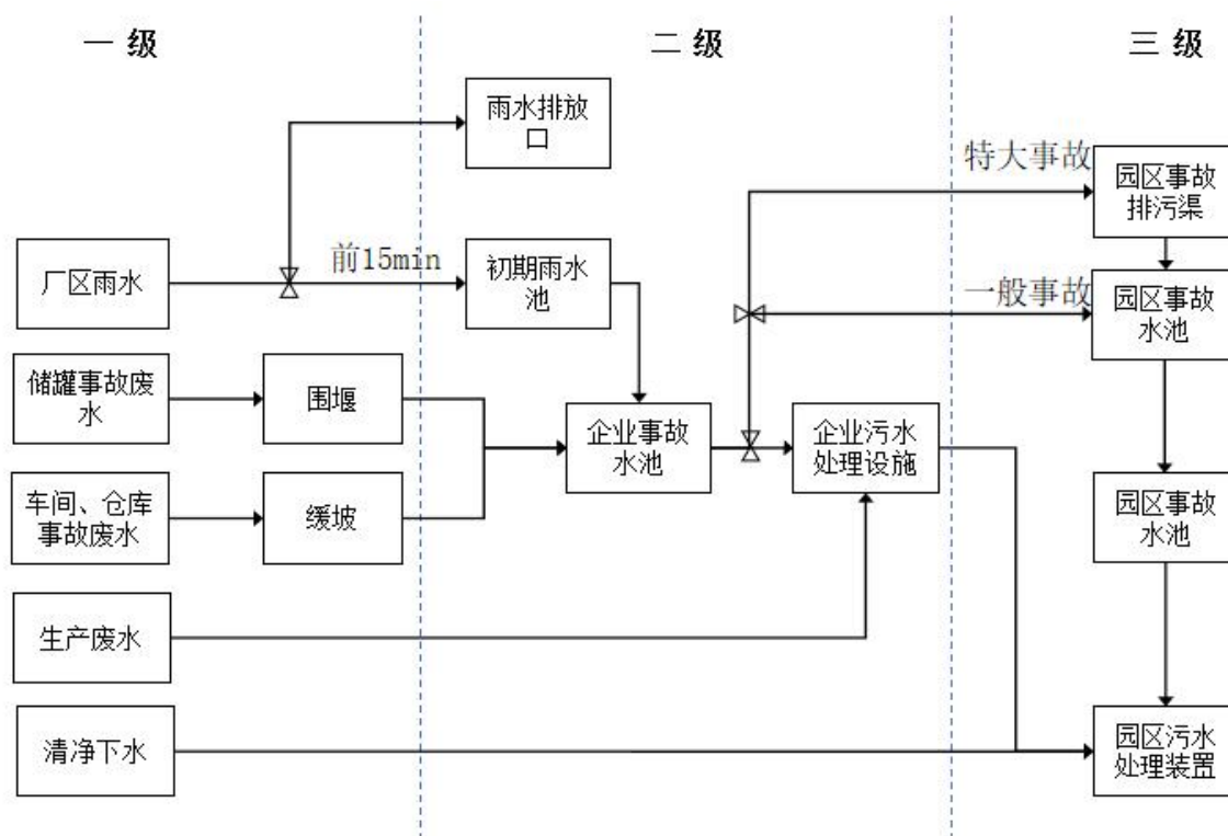
图 7.4-1 项目事故废水防控措施图
