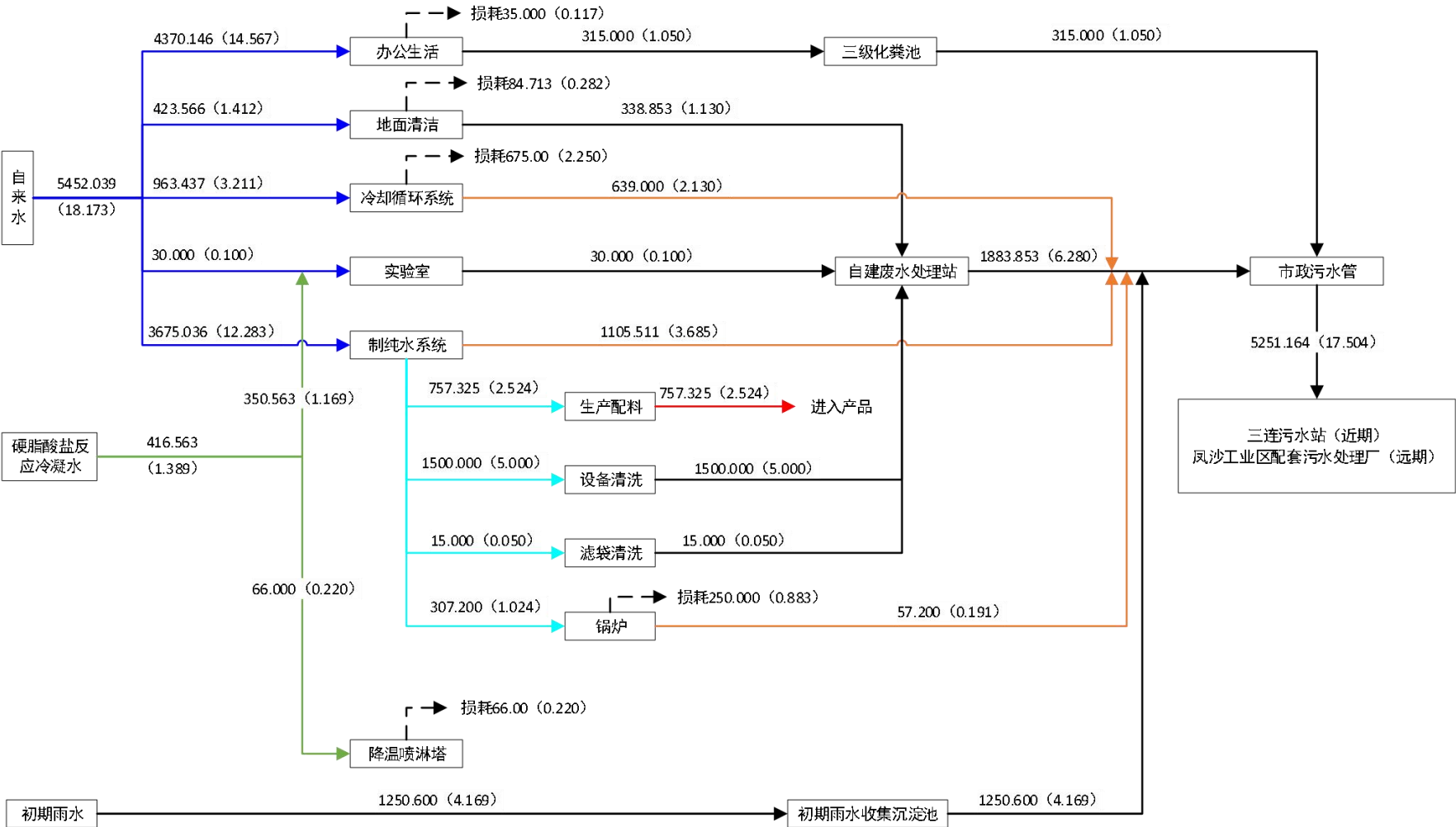
图 3.2-11 全厂水平衡图 单位: t/a (t/d)
