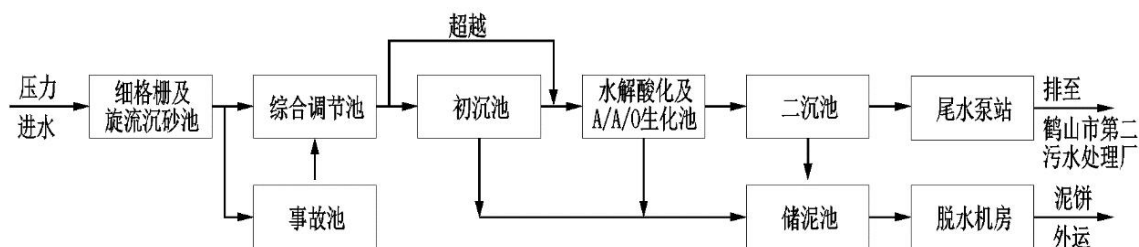
图 6.2-1 三连预处理站工艺流程图
