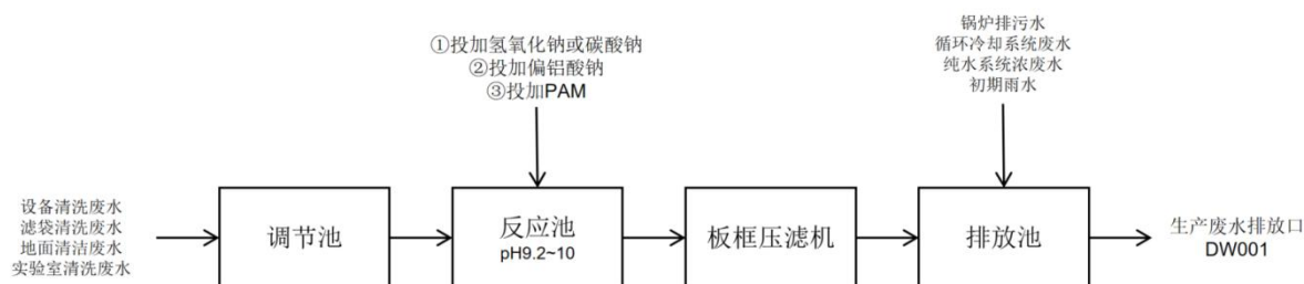
图 8.3-1 项目自建污水处理设施工艺流程图
