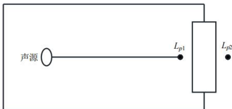
图 6.3-1 室内声源等效为室外声源图例
