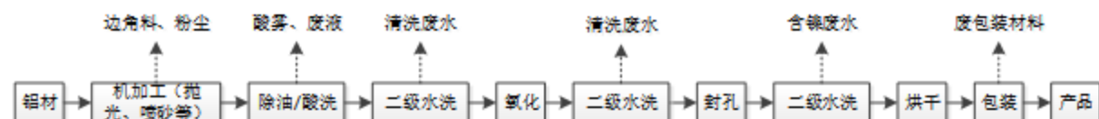
图 3.2-1 搬迁前项目铝制品生产工艺流程及产污环节图
