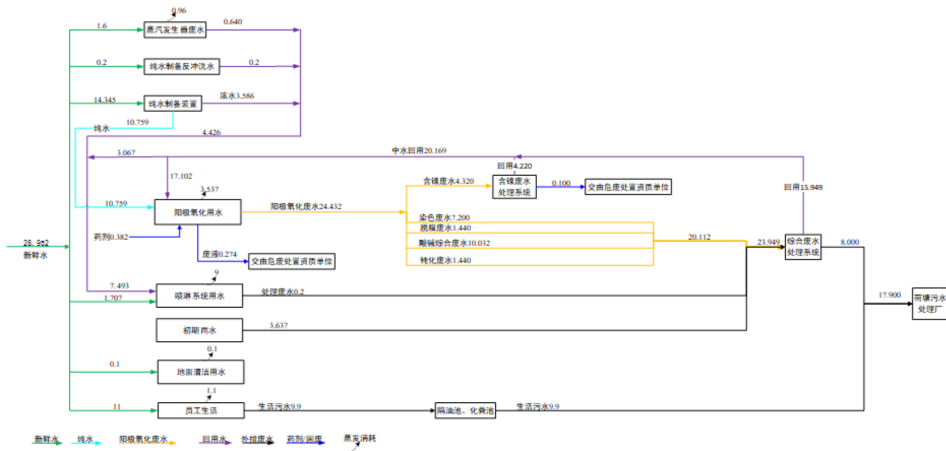
图 4.5-1 项目日水平衡图(单位: \text{m}^3/\text{d} )
