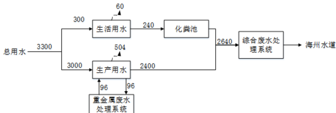
图 3.3-1 搬迁前项目厂区用水平衡图 单位 m³/a
