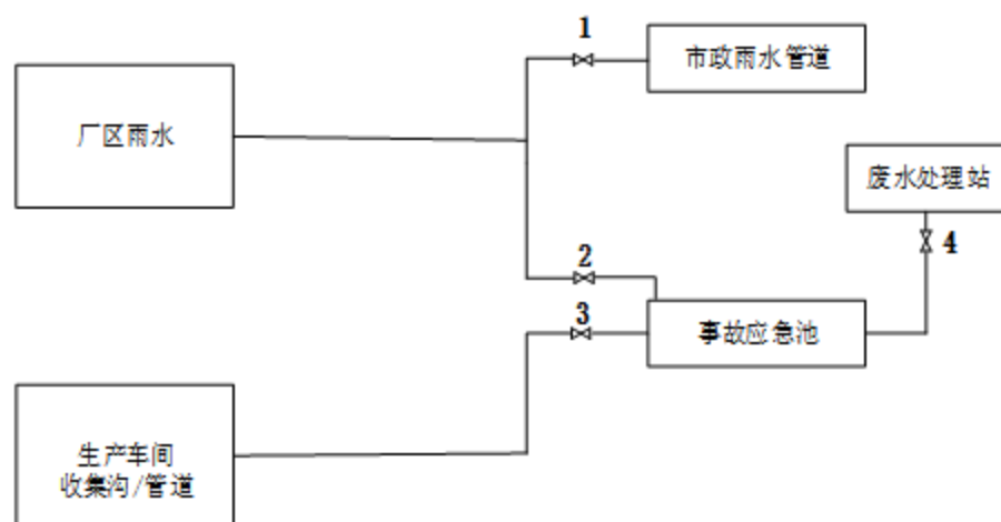
图 6.9-4 事故废水围堵示意图
