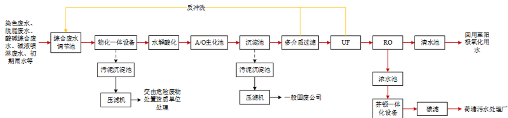
图 7.1-2 综合废水处理工艺图
