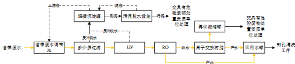
图 7.1-1 含镍废水处理工艺图
