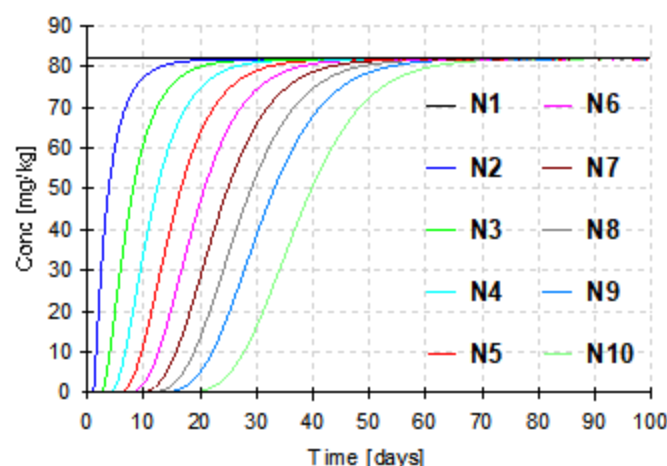
图 6.7-1 镍在不同时间的浓度分布图(N1~N9 为深度 0.0m、0.3m、0.6m、0.9m、1.2m、1.5m、1.8m、2.1m、2.4m、3m)
