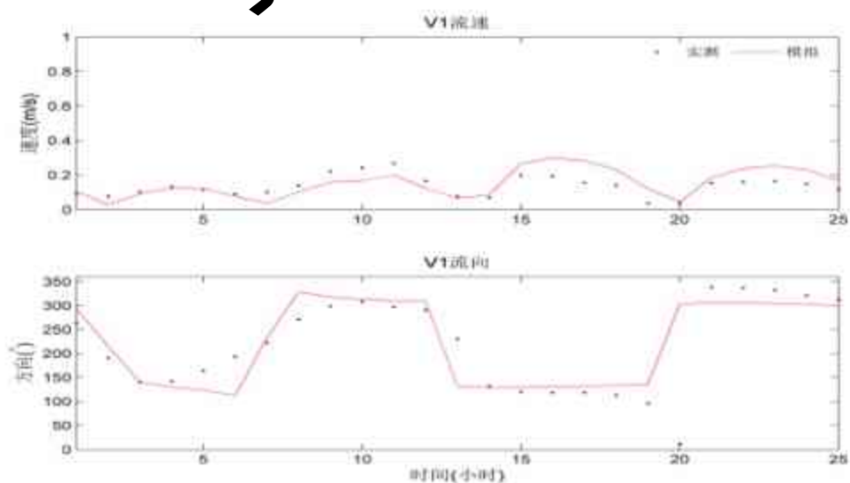
图 6.1.2-3a 2024 年 12 月表层流速流向验证图 (·表示实测值, —表示模拟值)
