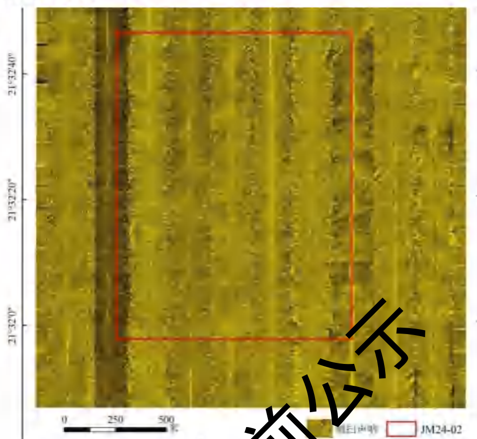
图 5.2.2-1 项目海域侧扫声呐图
