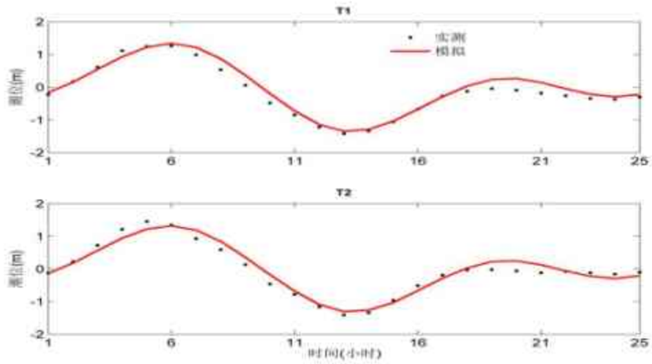
图 6.1.2-2 2024 年 12 月测站潮位验证曲线
