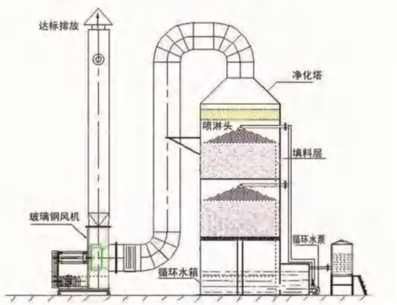
图 6.2-1b 废气喷淋处理装置示意图
