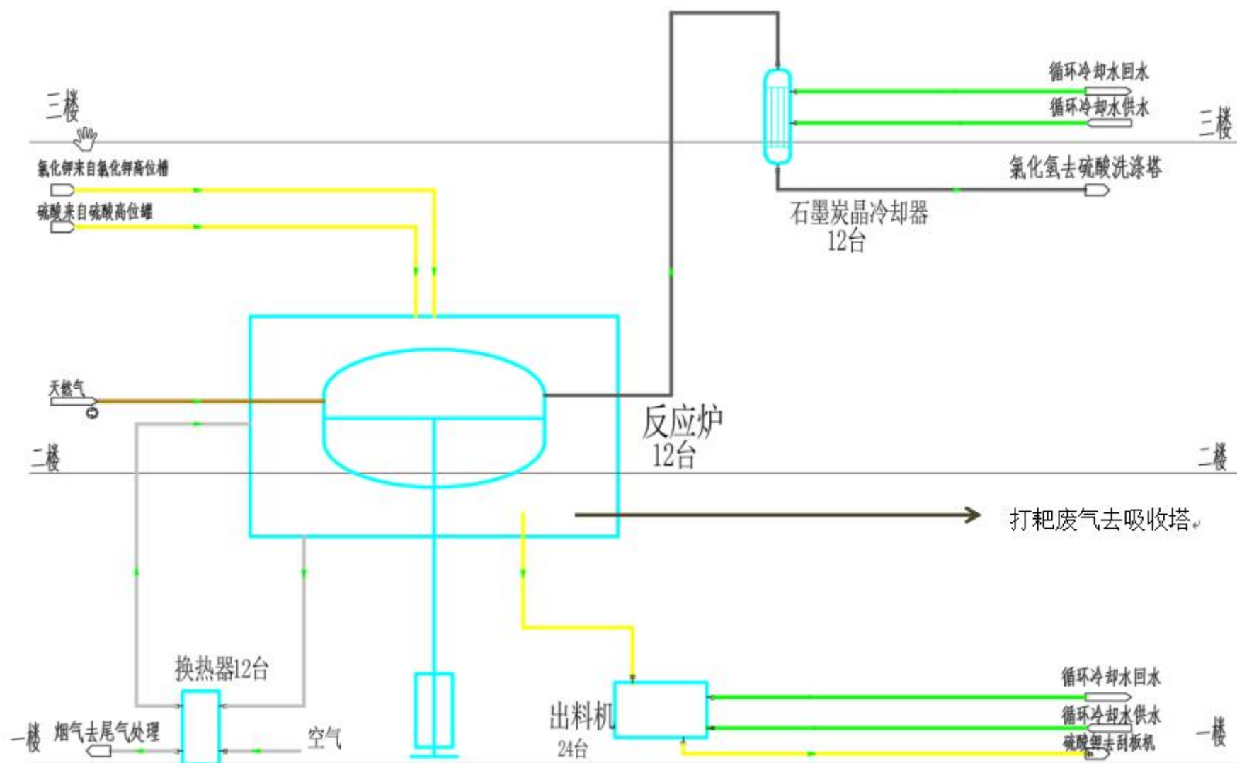
图 3.3-2 (3) 反应炉设备连接图
