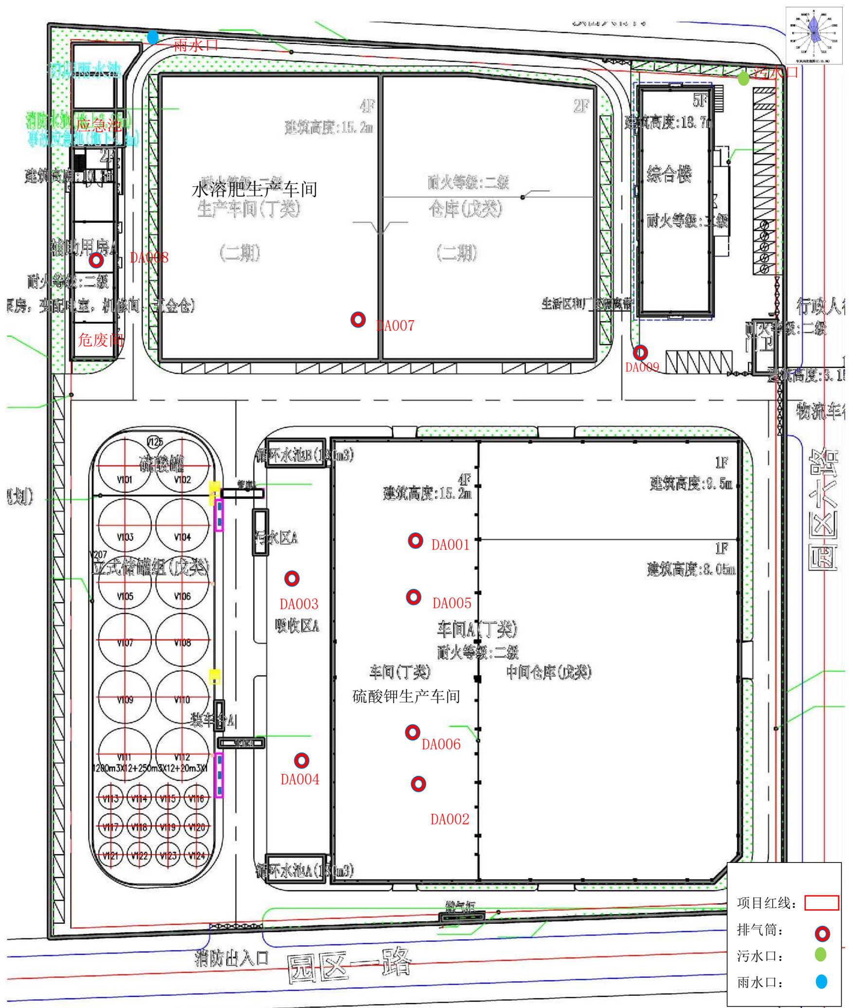
图 3.1-4 项目总平面图
