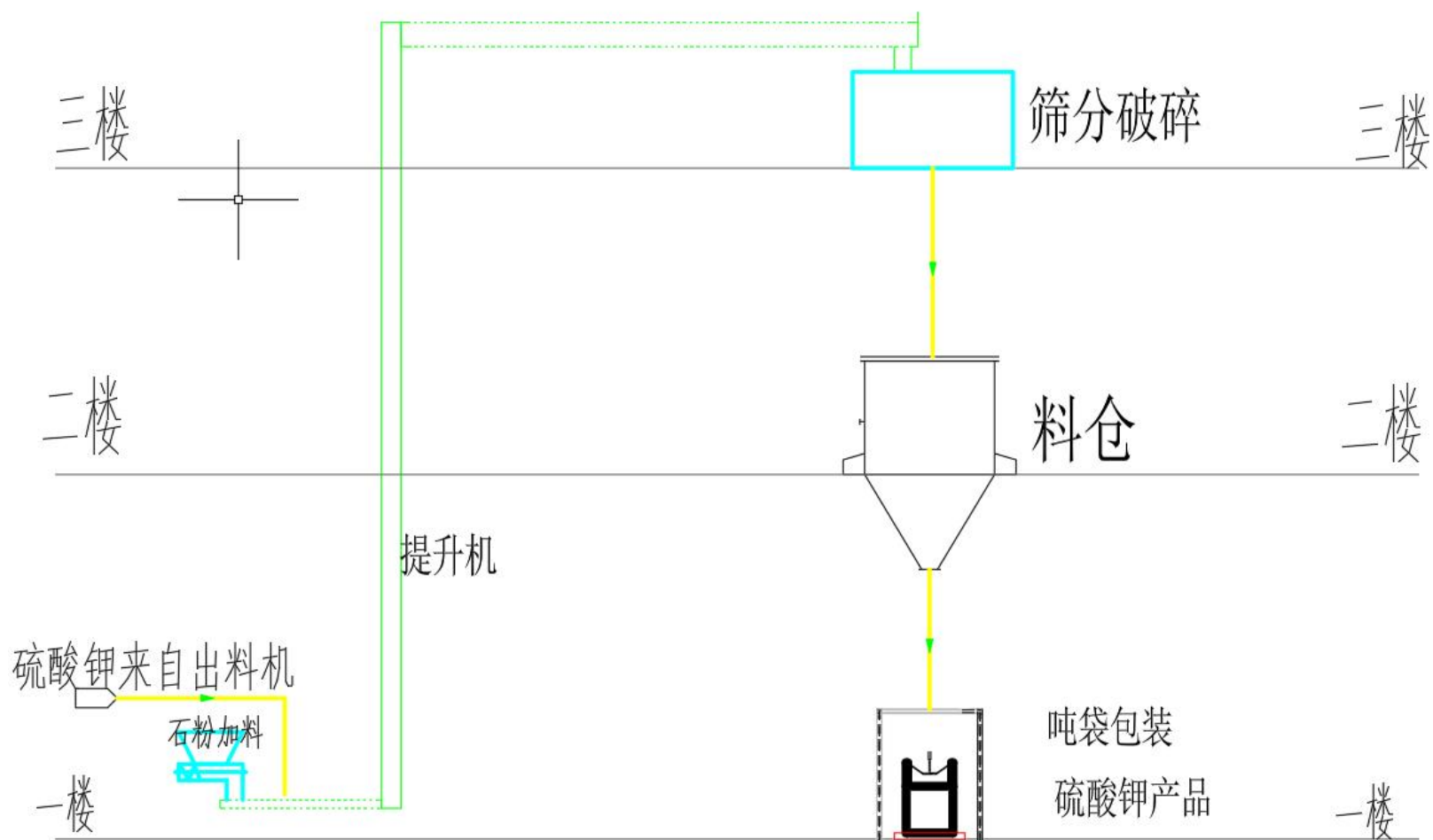
图 3.3-2 (4) 筛分粉碎包装设备连接图
