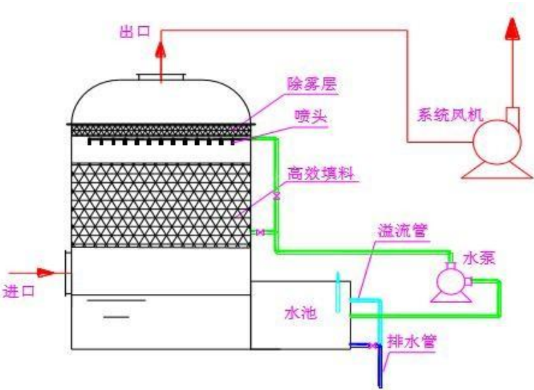
图 6.3-1 喷淋塔示意图
