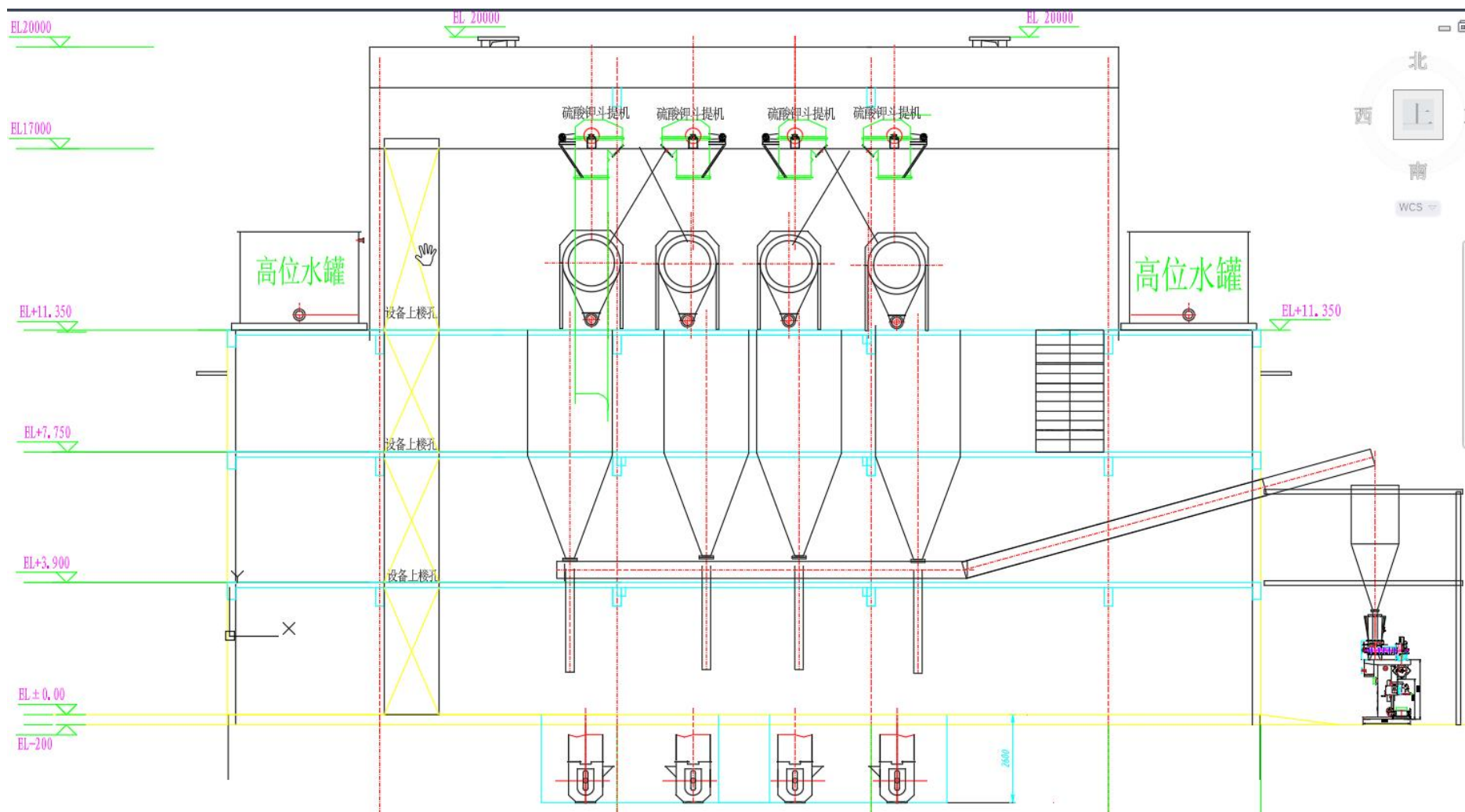
图 3.1-5 (3) 项目成品包装设备布置图 (立面图)
