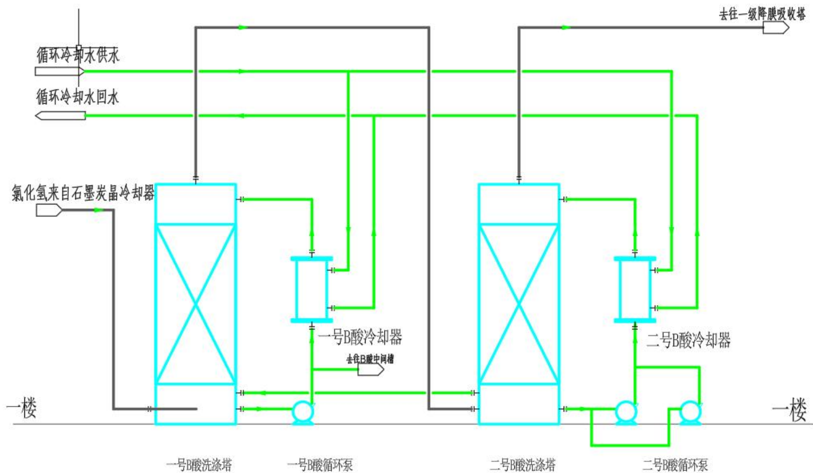
图 3.3-2 (5) 硫酸洗涤设备连接图
