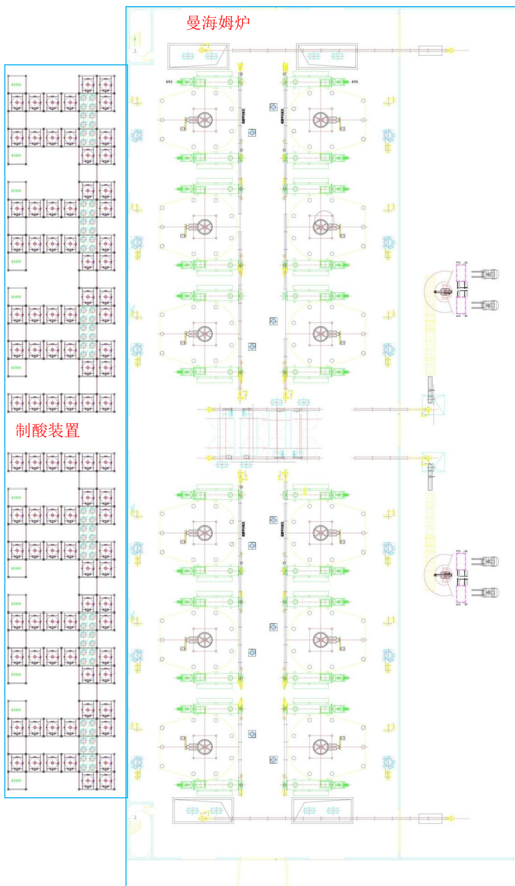
图 3.1-5 项目硫酸钾生产车间设备布置图
