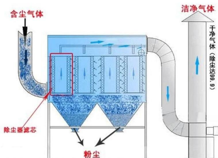
图 6.3-2 袋式除尘器结构图
