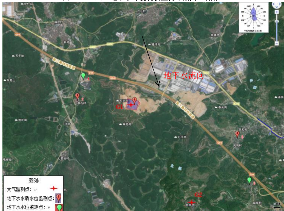
图 4.2-14 (2) 地下水环境现状监测布点图
