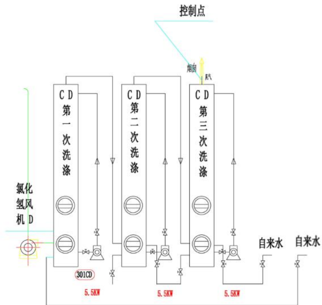
图 3.3-2 (7) 尾气吸收设备连接图
