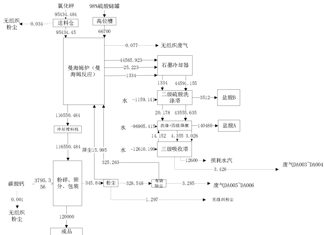
图 3.3-6 硫酸钾生产物料平衡图 (t/a)
