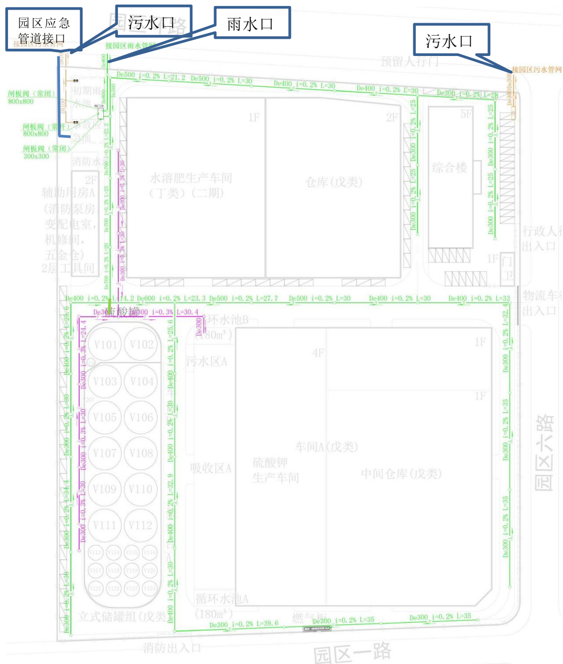
排水管网方案图
