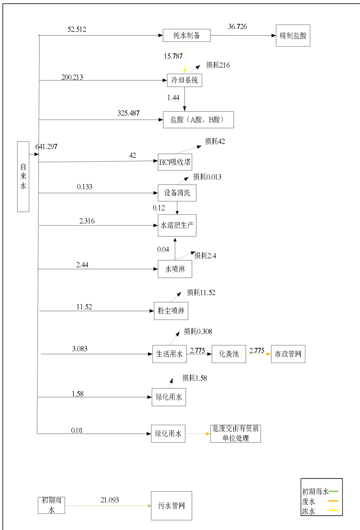
图 3.3-7 项目用水和排水平衡图 单位: t/d
