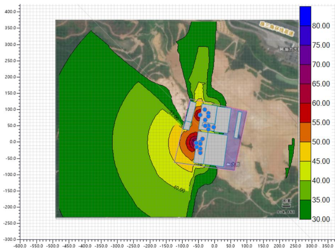
图 5.2.3-1 项目噪声等值线图
