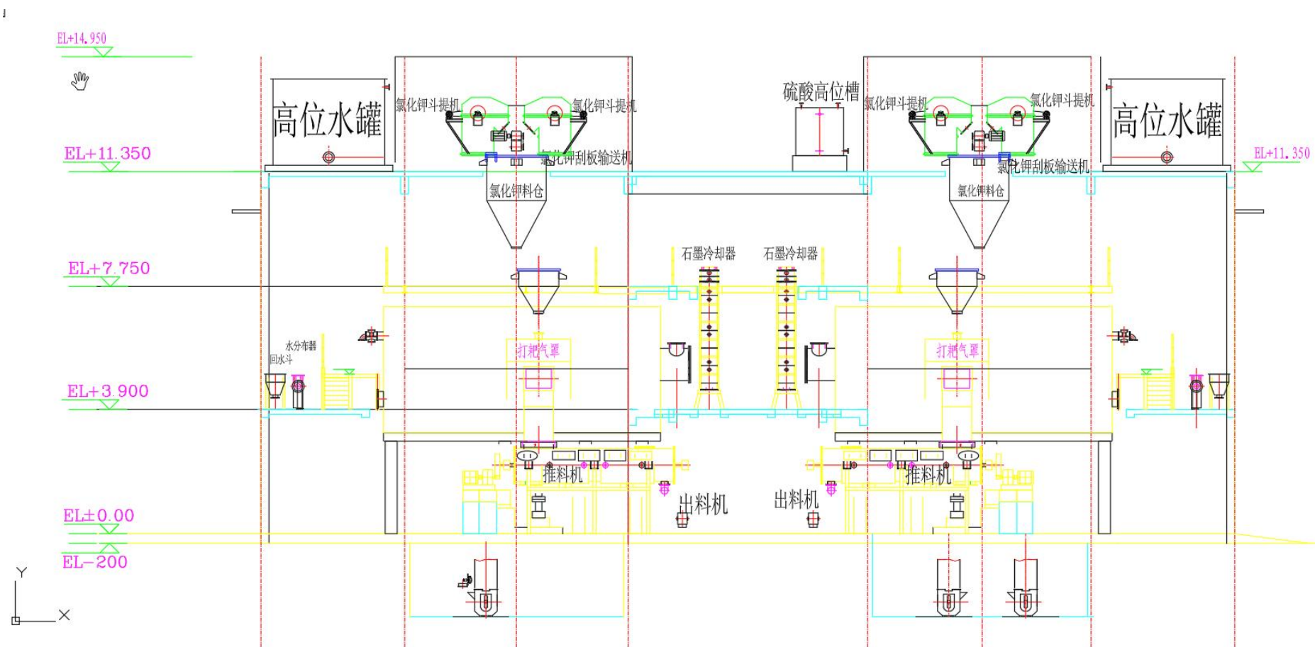
图 3.1-5 (2) 项目硫酸钾生产车间设备布置图 (立面图)
