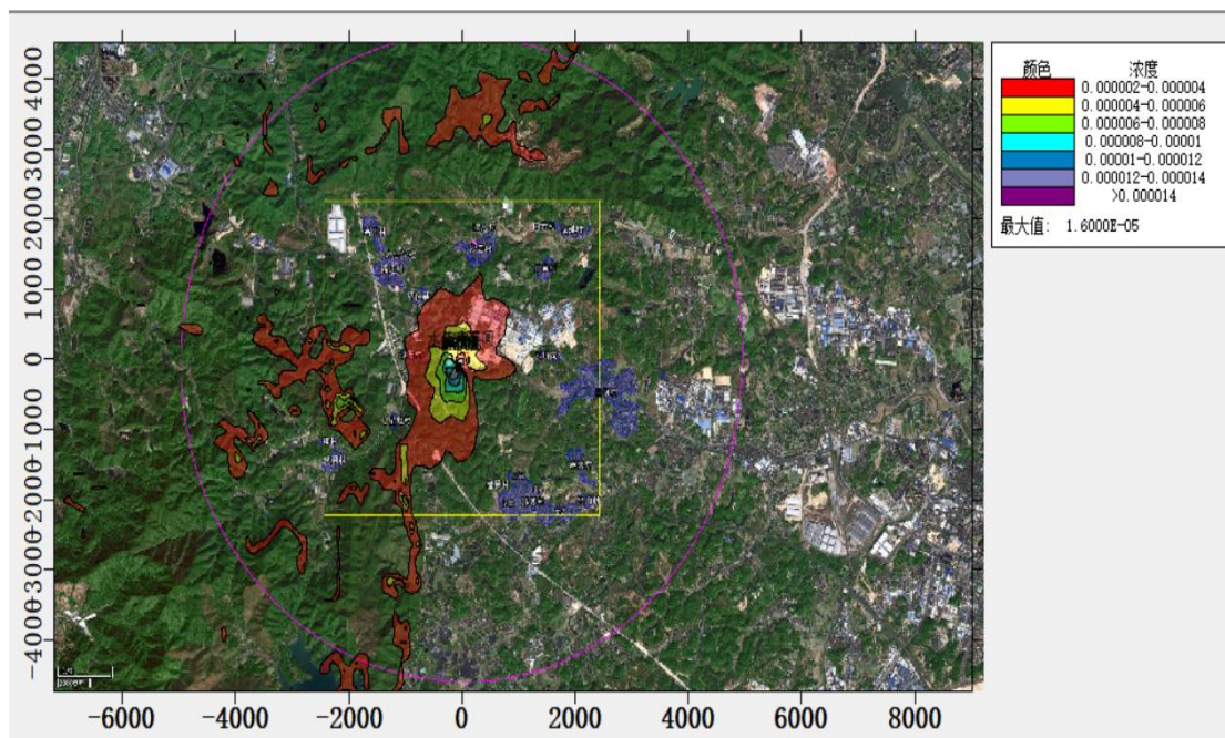
图 5.2.1-8 SO 2 日平均浓度等值线图
