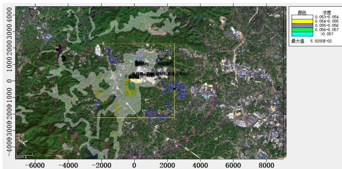
图 5.2.1-29 NO x 叠加后日均浓度等值线图
