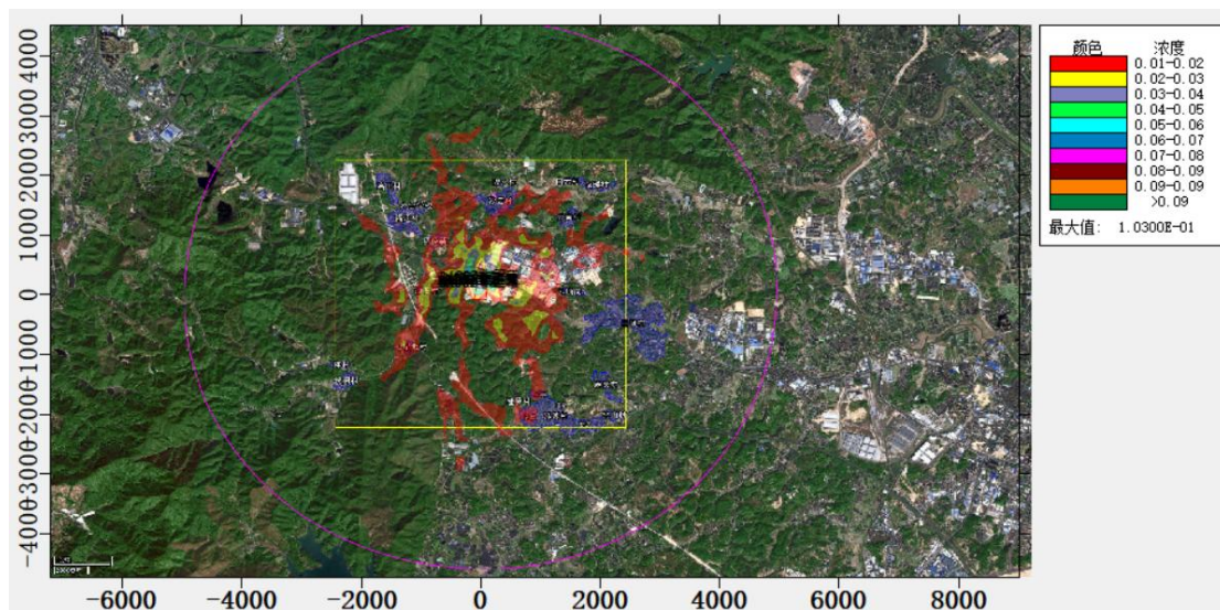
图 5.2.1-42 氯化氢 1 小时浓度等值线图（非正常排放）
