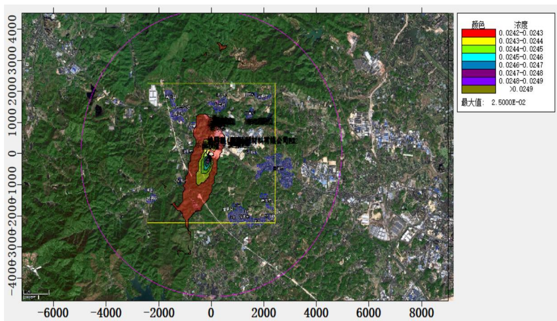
图 5.2.1-27 NO 2 叠加后年平均浓度等值线图
