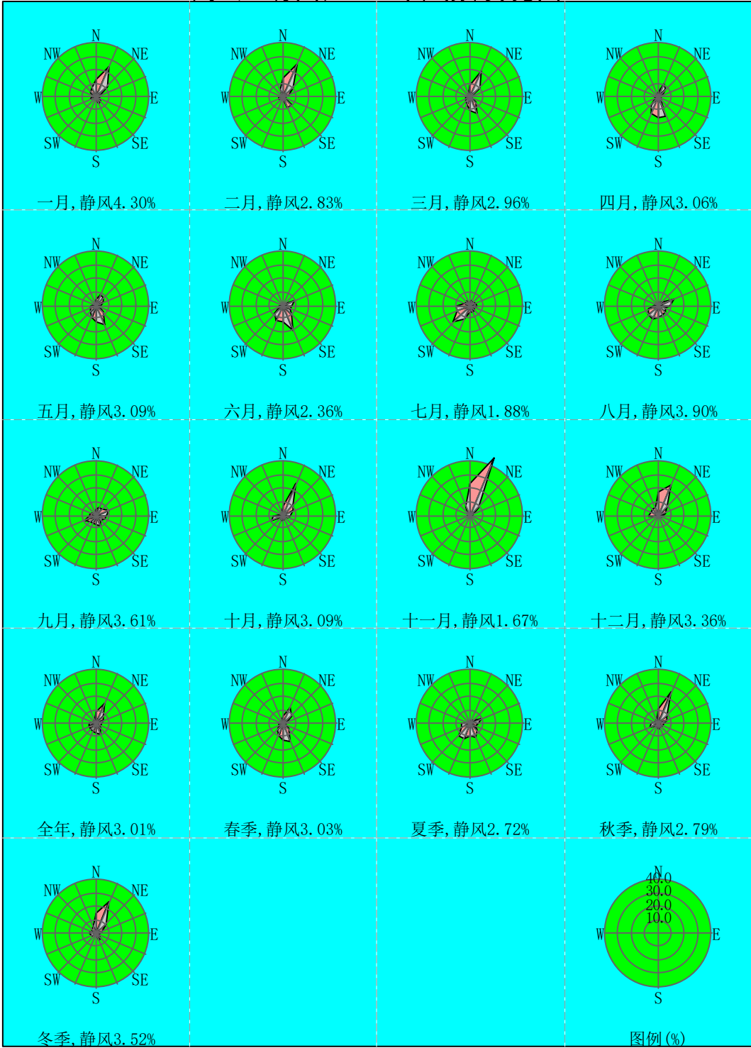
图 5.2.1-6 2025 年鹤山不同季节风速频率玫瑰图
