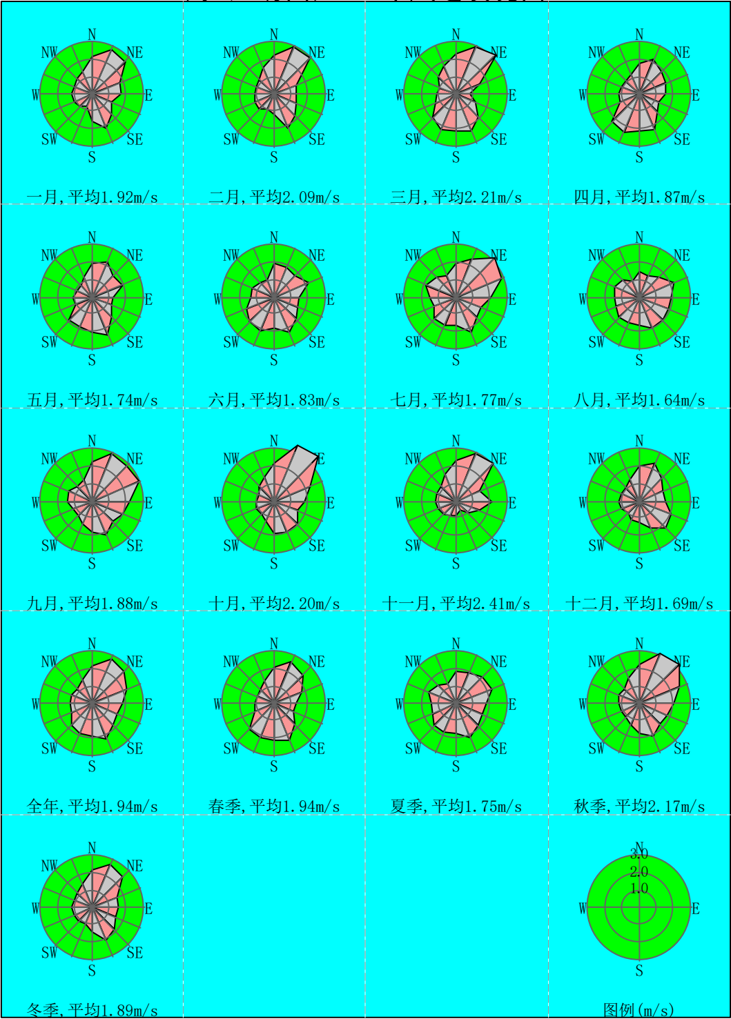
图 5.2.1-5 2025 年鹤山不同季节风速玫瑰图
