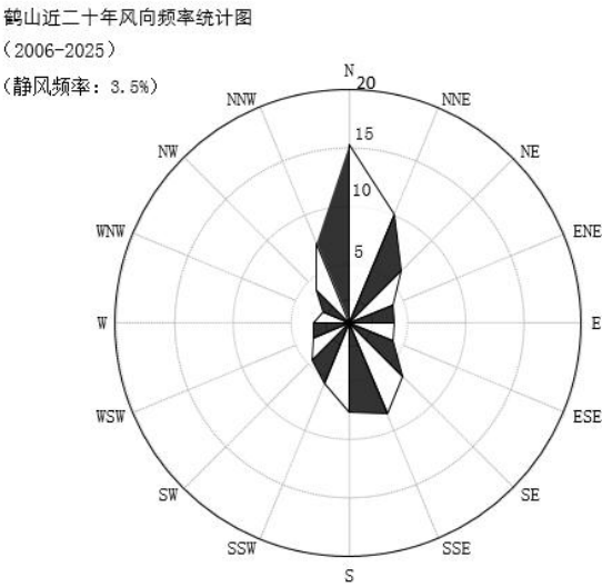
图 5.2.1-1 鹤山气象站累年各风向玫瑰图（统计年限：2006~2025 年）
