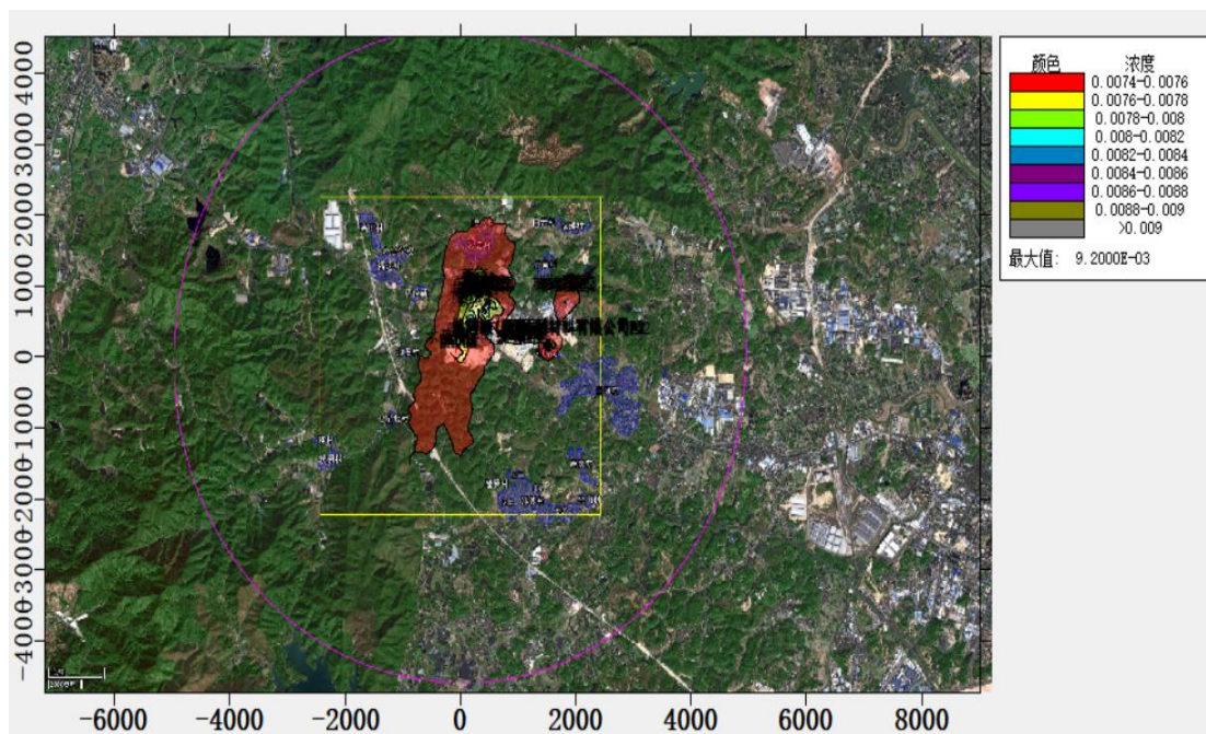
图 5.2.1-25 SO 2 叠加后年平均浓度等值线图
