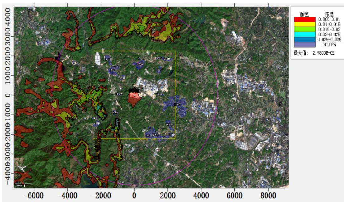
图 5.2.1-10 NO x 1 小时浓度等值线图
