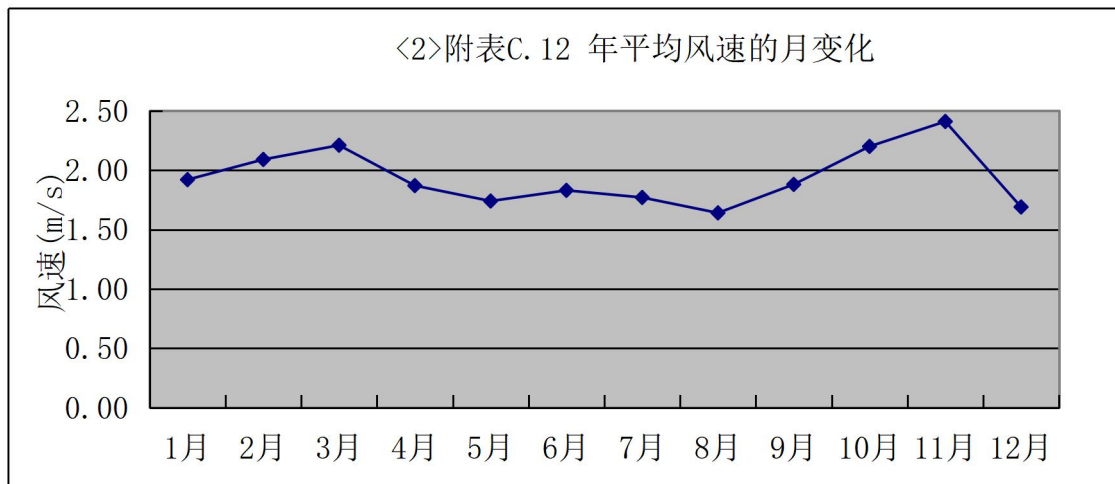
图 5.2.1-2 2025 年鹤山平均风速的月变化曲线
