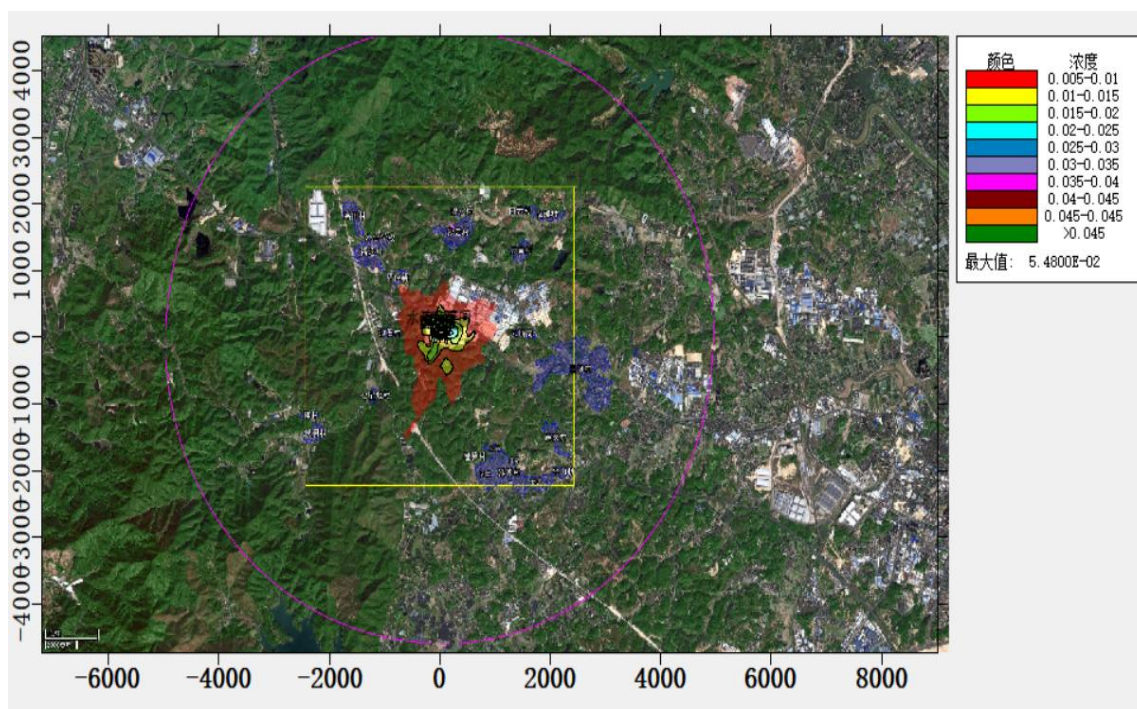
图 5.2.1-13 TSP 日平均浓度等值线图
