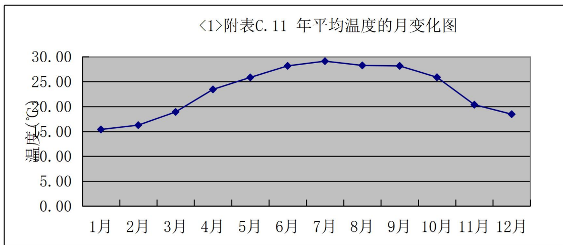
图 5.2.1-3 2025 年鹤山平均温度的月变化曲线
