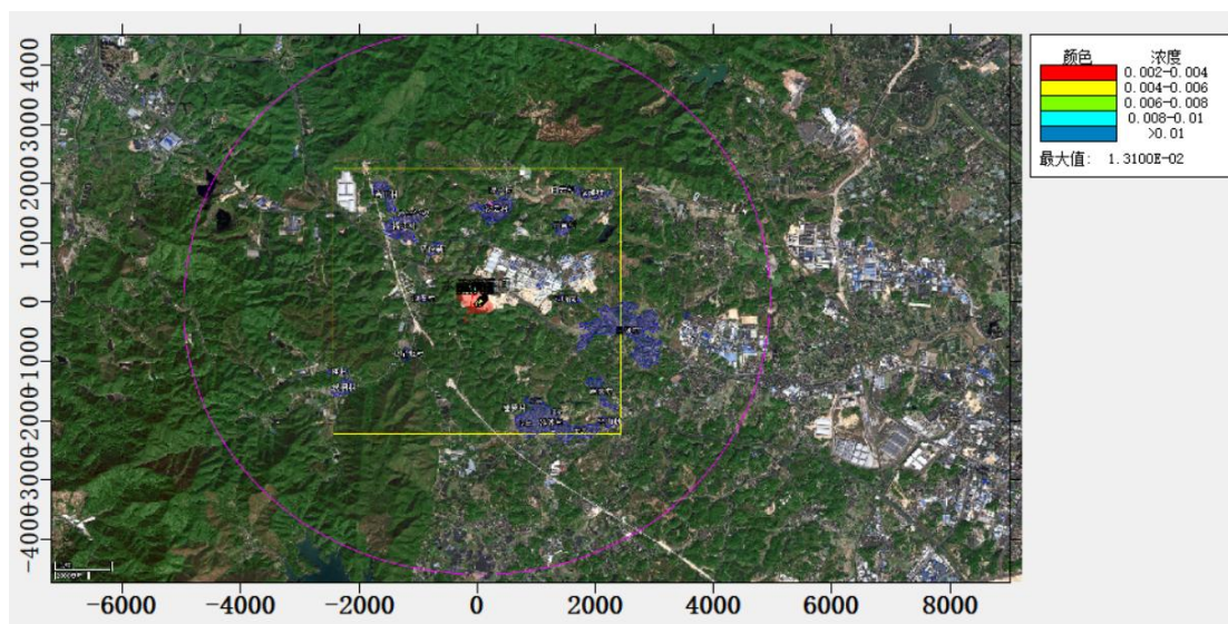
图 5.2.1-19 氨 1 小时浓度等值线图
