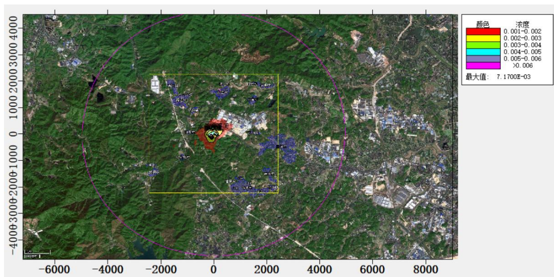
图 5.2.1-23 硫酸雾日平均浓度等值线图
