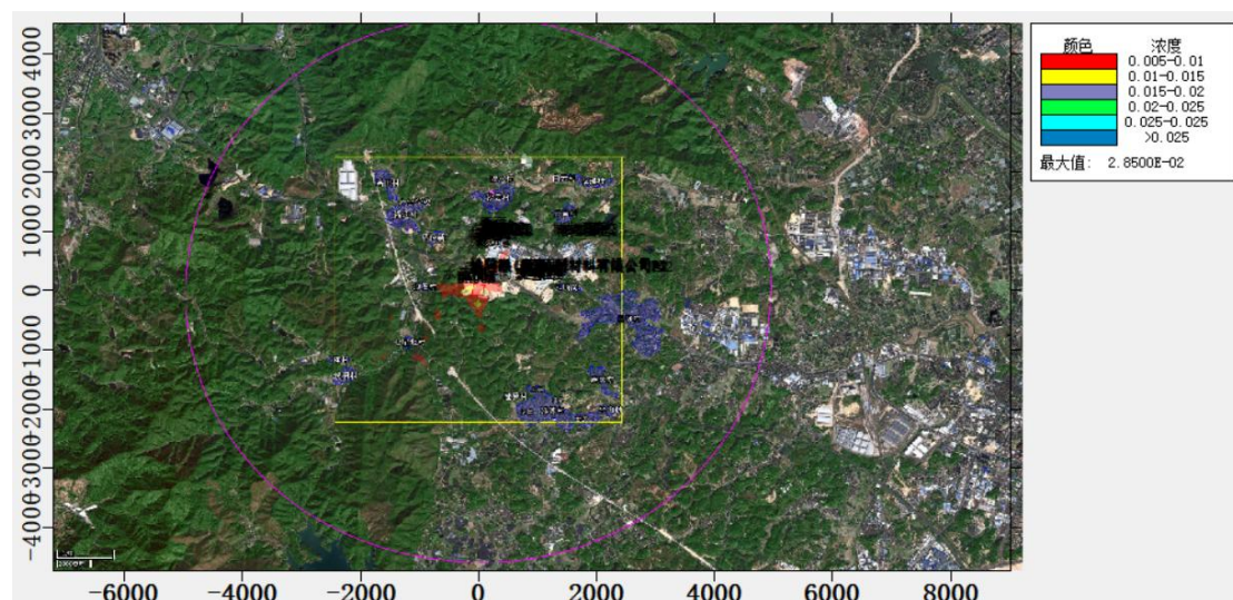
图 5.2.1-36 氯化氢叠加后 1 小时浓度等值线图
