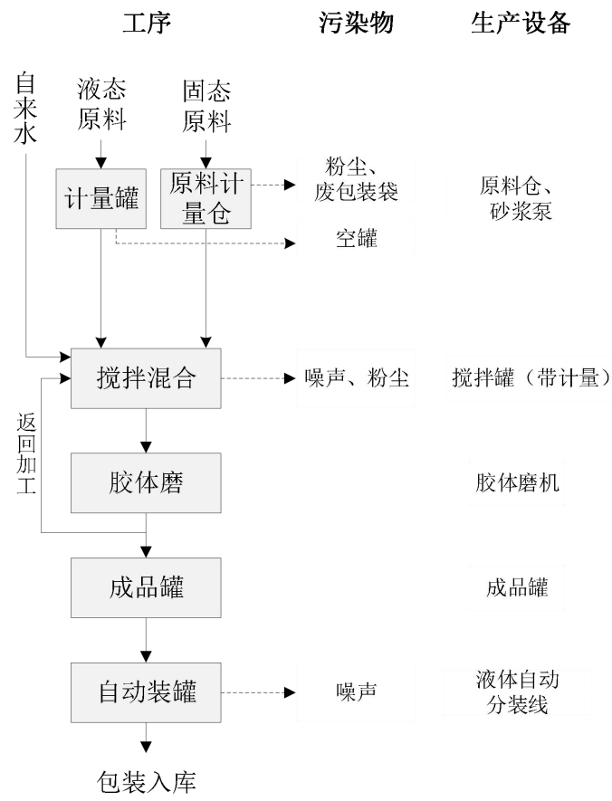
图 3.3-5 水溶肥（液态）生产工艺流程及产污分析图
