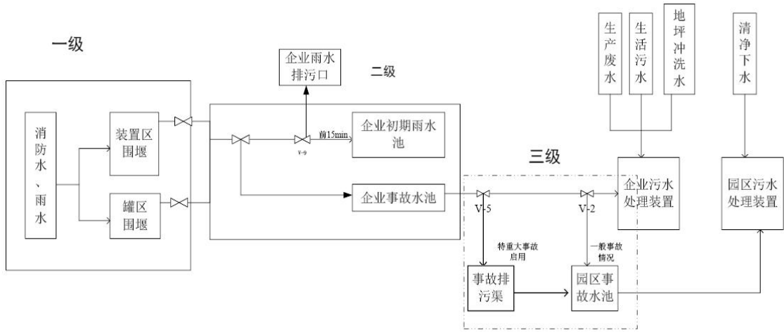
图 5.2.8-5 园区事故状态下废水收集示意图
