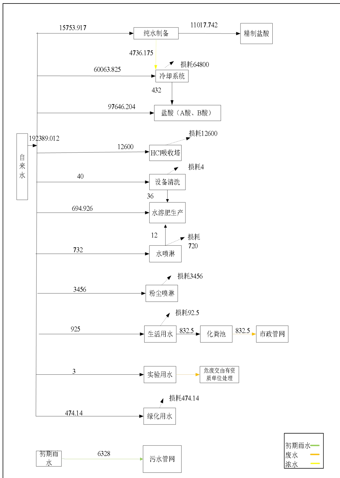
图 3.3-6 项目用水和排水平衡图 单位: t/a
