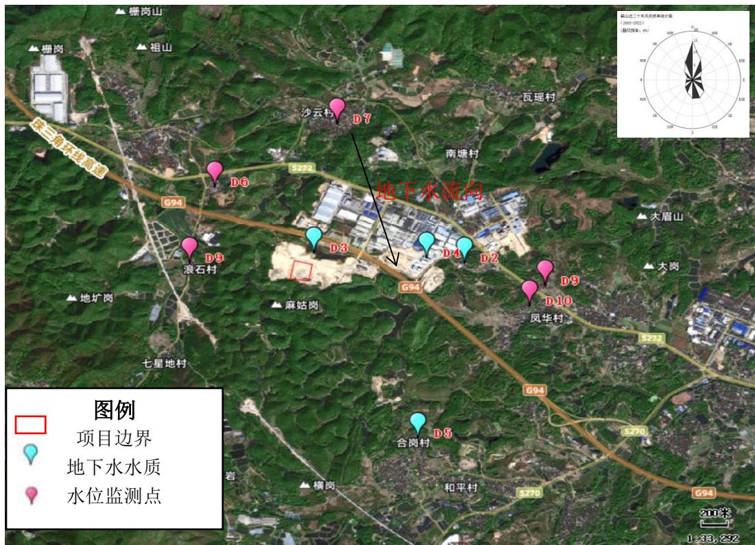
图 4.2-14 (1) 地下水环境现状监测布点图 (引用)
