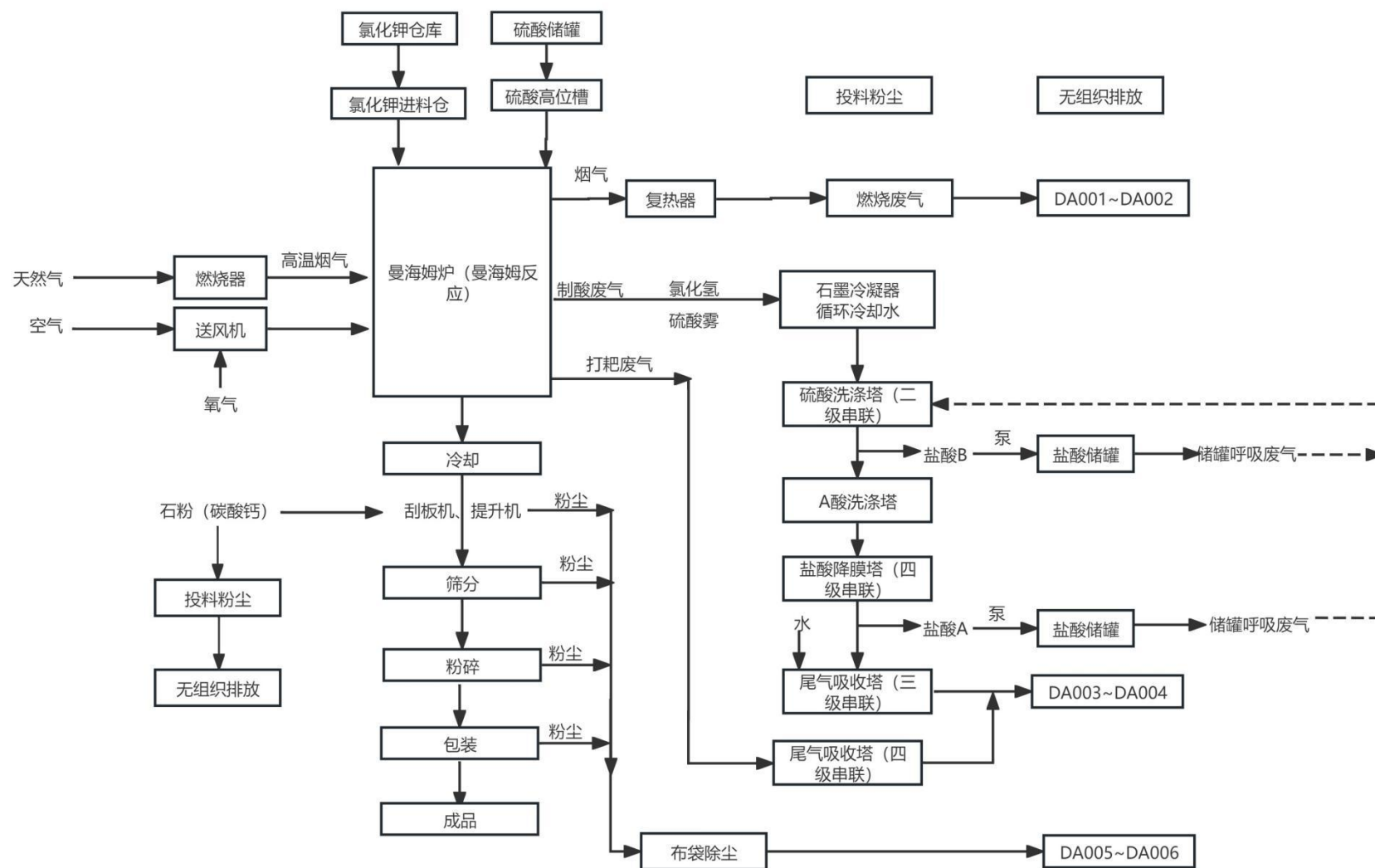
图3.3-1 硫酸钾生产工艺流程图
