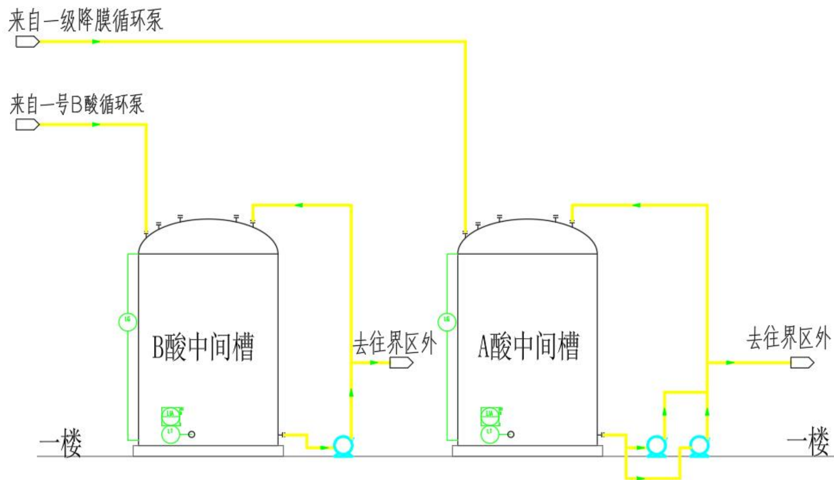
图 3.3-2 (8) 盐酸储存设备连接图
