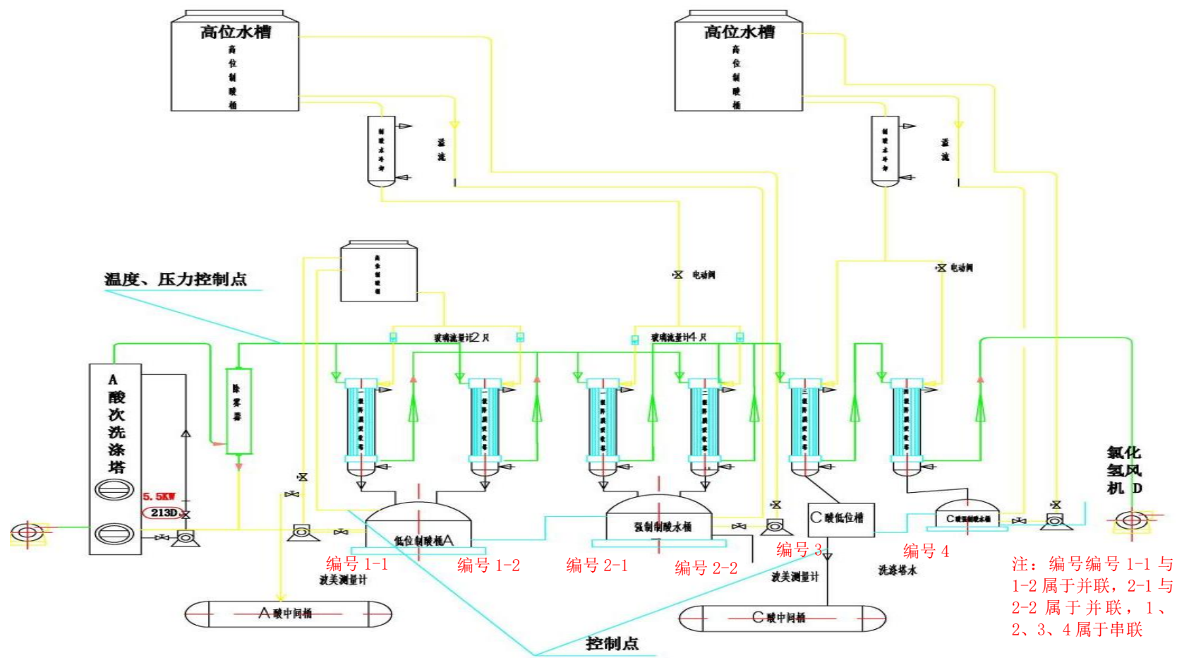
图 3.3-2 (6) 降膜吸收塔设备连接图
