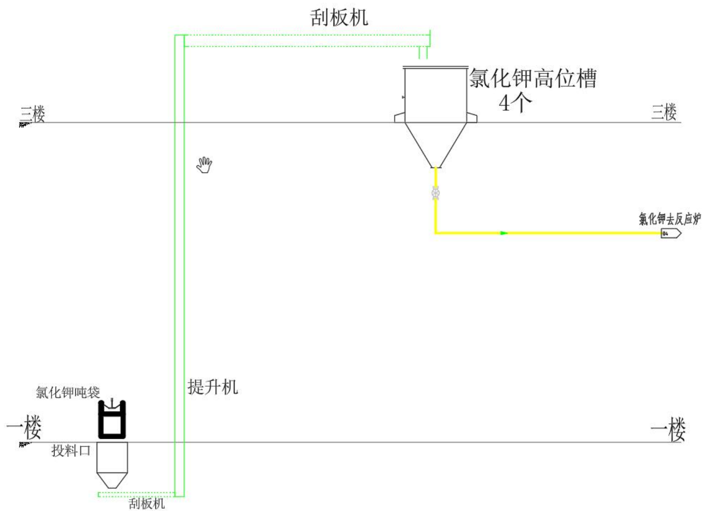
图 3.3-2 (2) 氯化钾上料设备连接图
