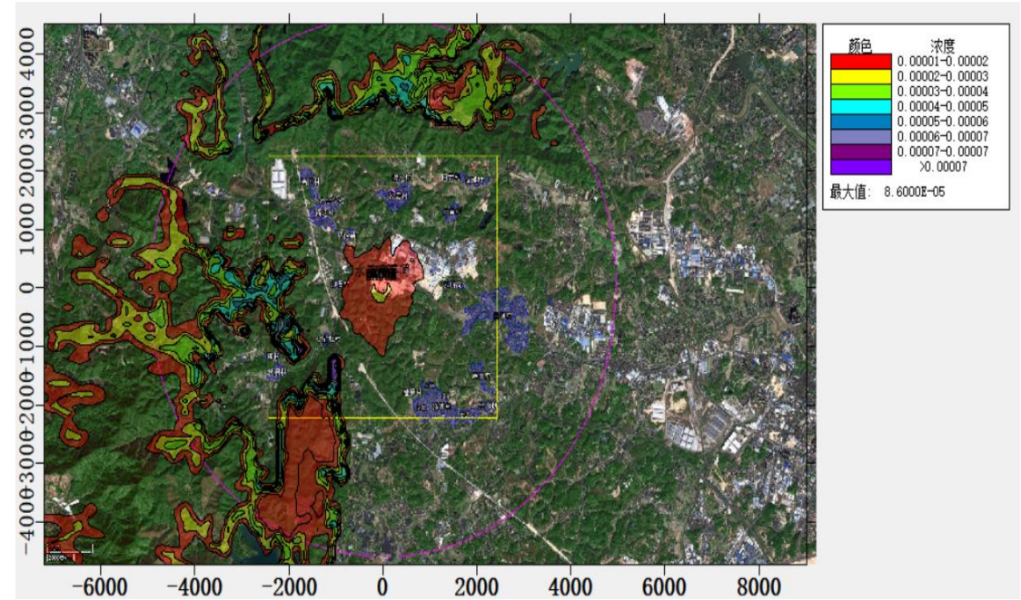
图 5.2.1-7 SO 2 1 小时浓度等值线图
