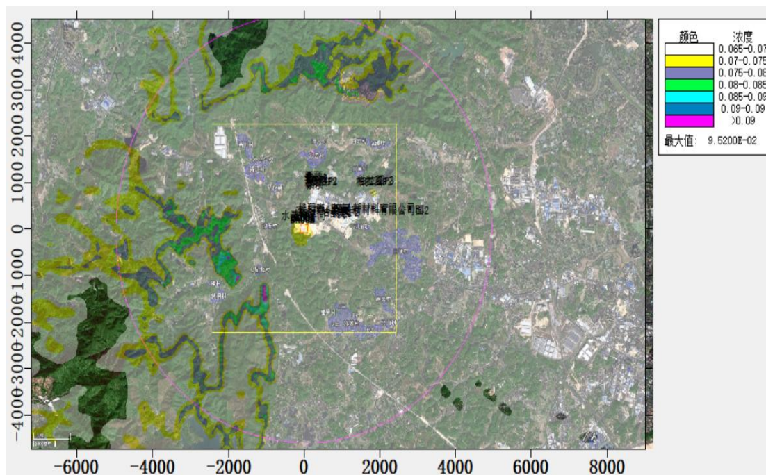
图 5.2.1-28 NO x 叠加后 1 小时浓度等值线图
