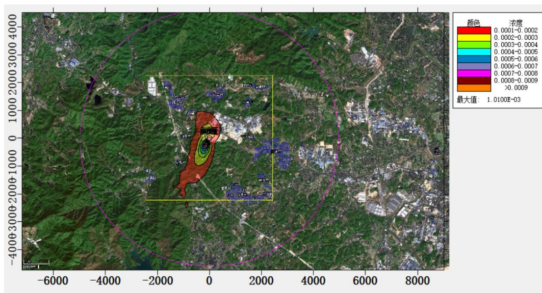
图 5.2.1-12 NO x 年平均浓度等值线图
