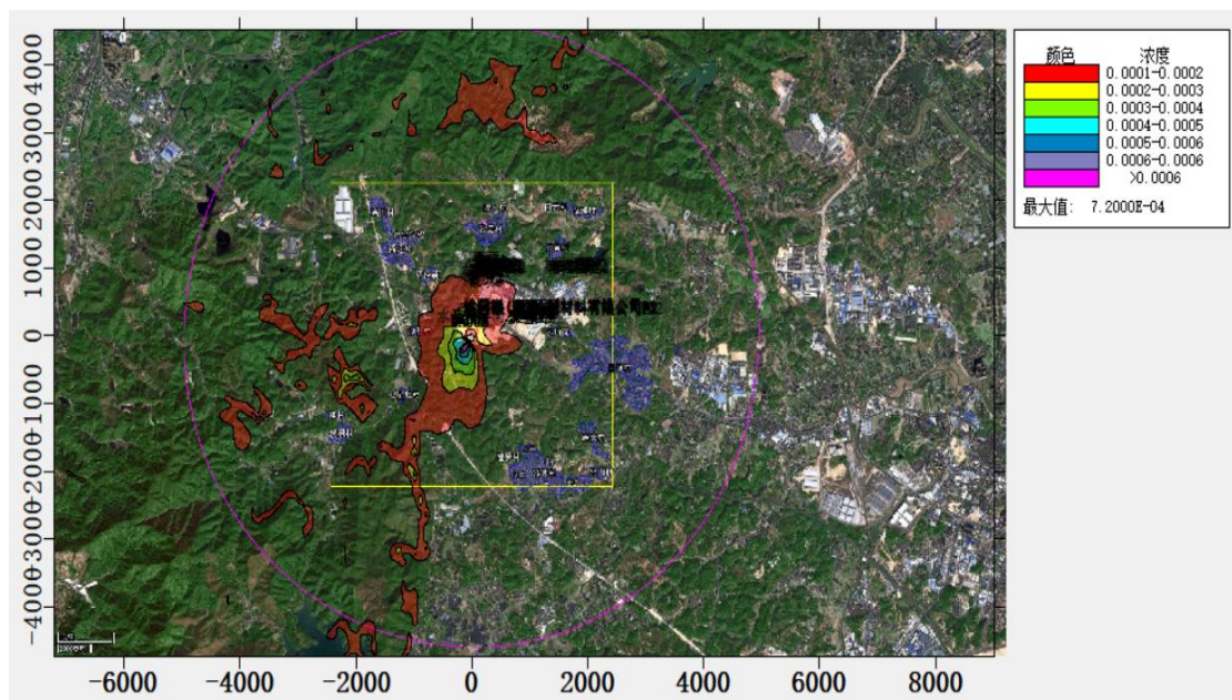
图 5.2.1-17 PM 2.5 日平均浓度等值线图
