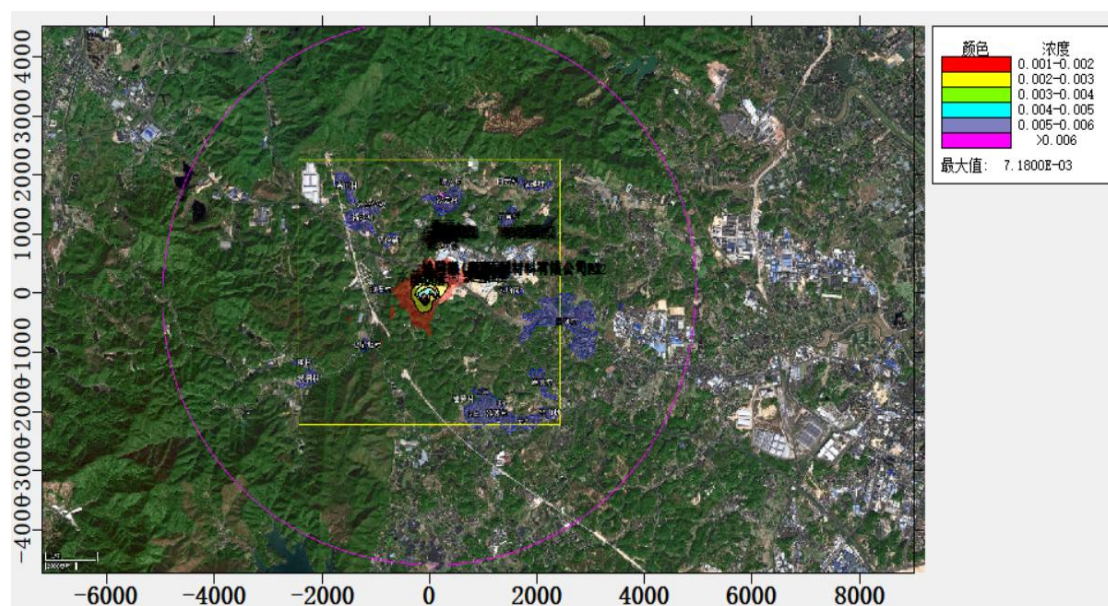
图 5.2.1-39 硫酸雾叠加后日均浓度等值线图
