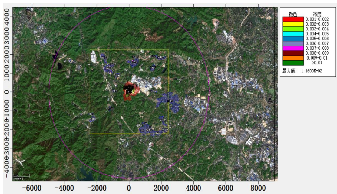
图 5.2.1-14 TSP 年平均浓度等值线图
