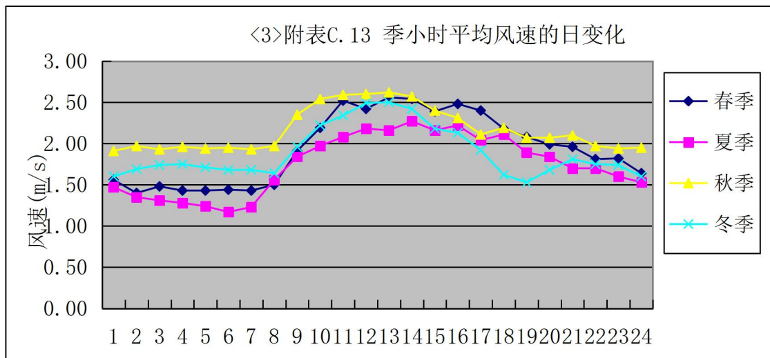
图 5.2.1-4 2025 年鹤山季小时平均风速的日变化
