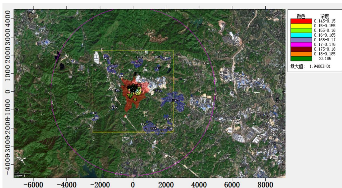
图 5.2.1-34 TSP 叠加后日平均浓度等值线图
