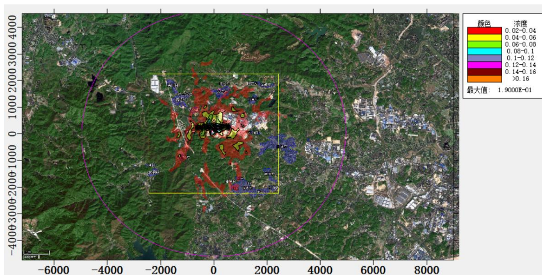
图 5.2.1-43 硫酸雾 1 小时浓度等值线图（非正常排放）
