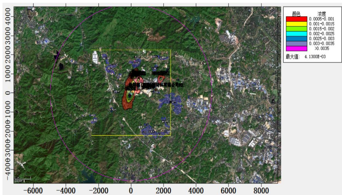
图 5.2.1-16 PM 10 年平均浓度等值线图
