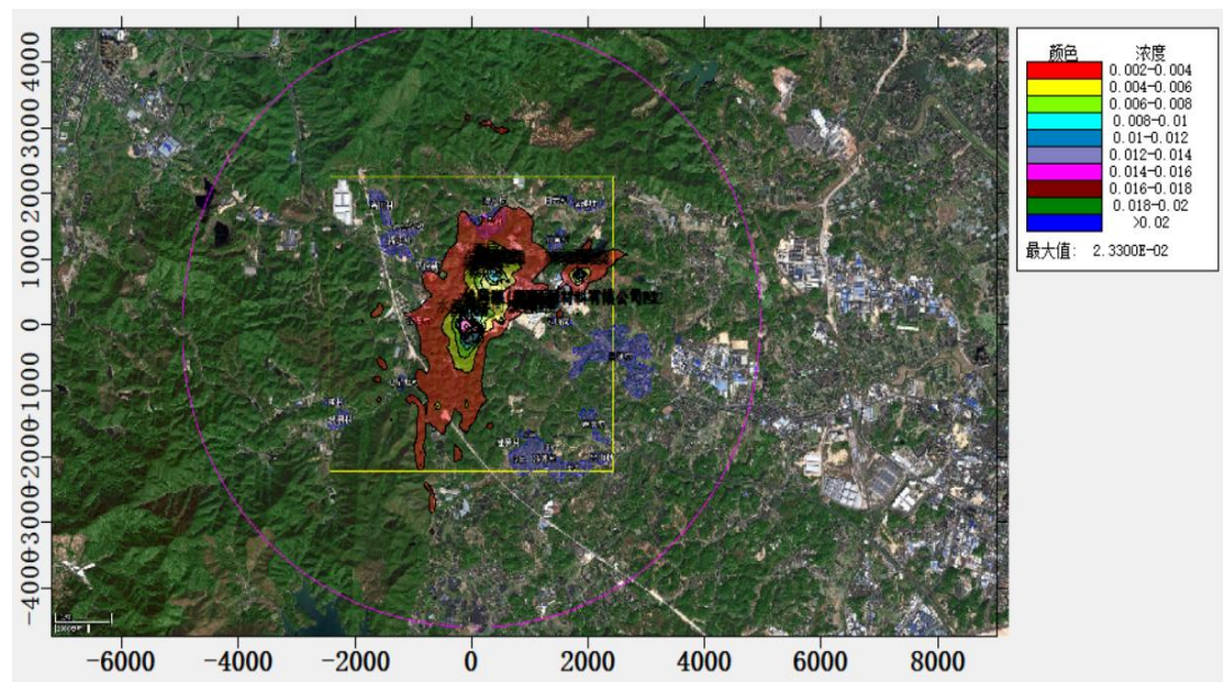
图 5.2.1-15 PM 10 日平均浓度等值线图
