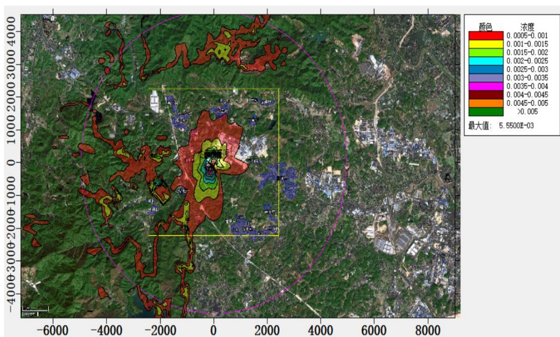
图 5.2.1-11 NO x 日平均浓度等值线图
