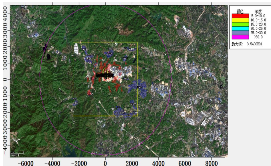
图 5.2.1-40 TSP 1 小时浓度等值线图（非正常排放）
