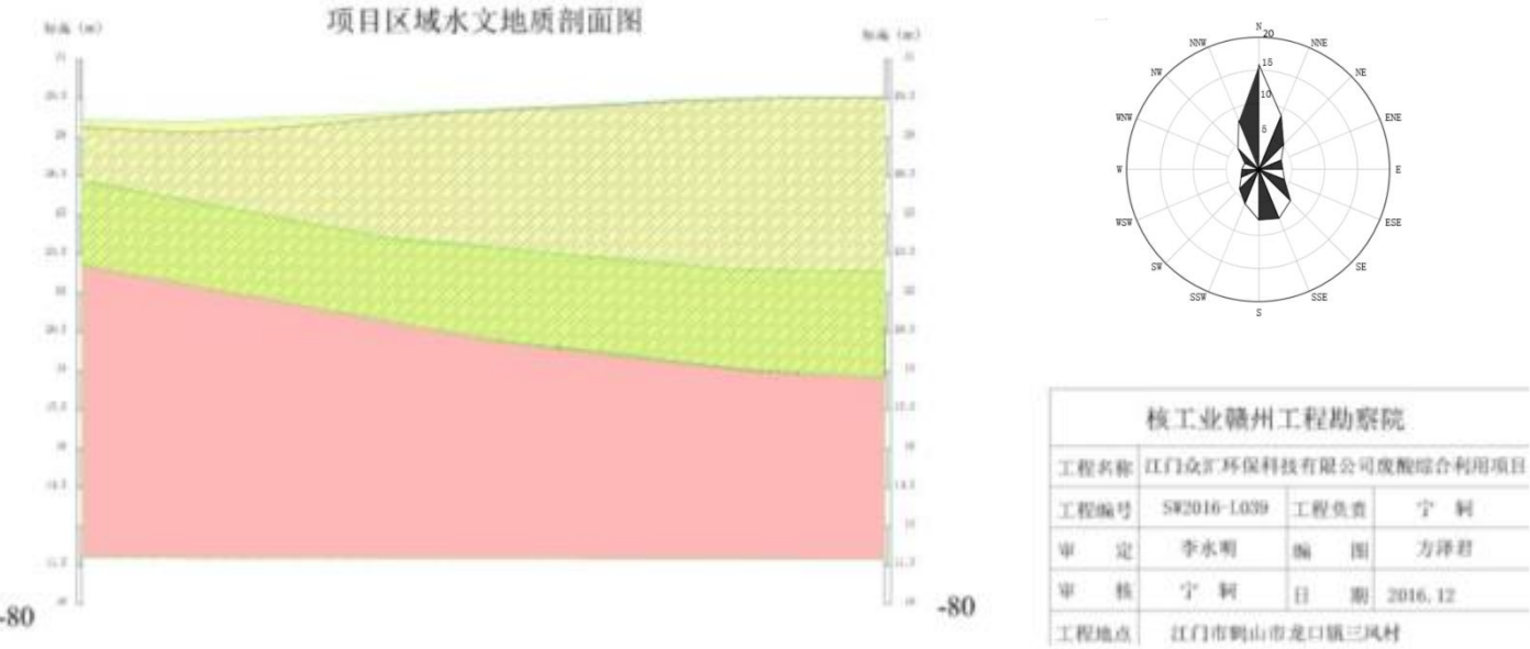
图 4.2-3 区域水文地质图
