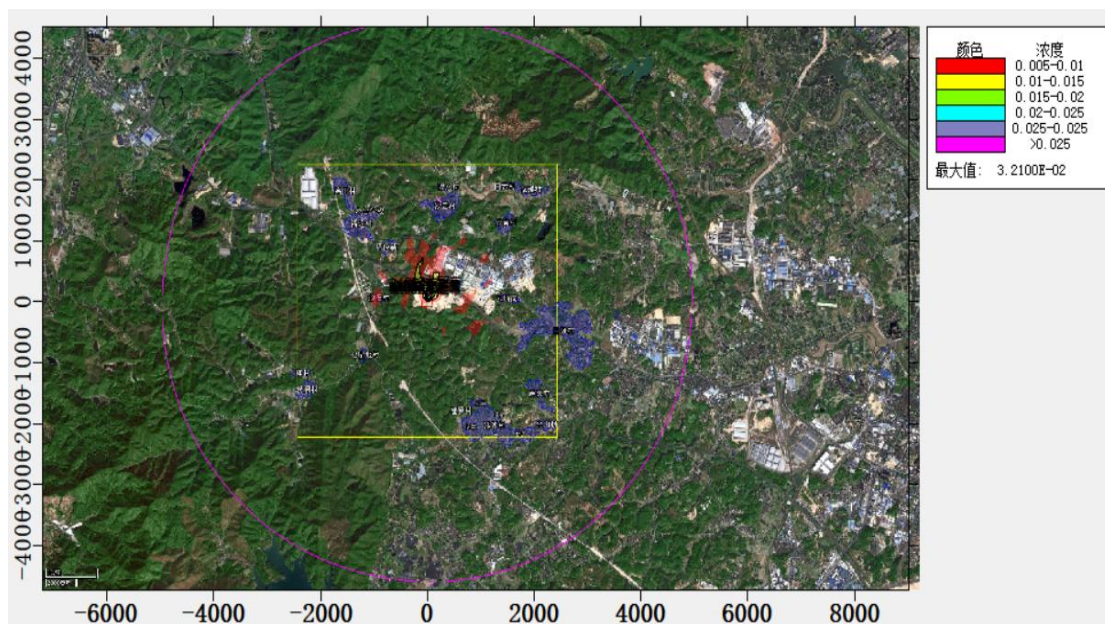
图 5.2.1-41 氨 1 小时浓度等值线图（非正常排放）
