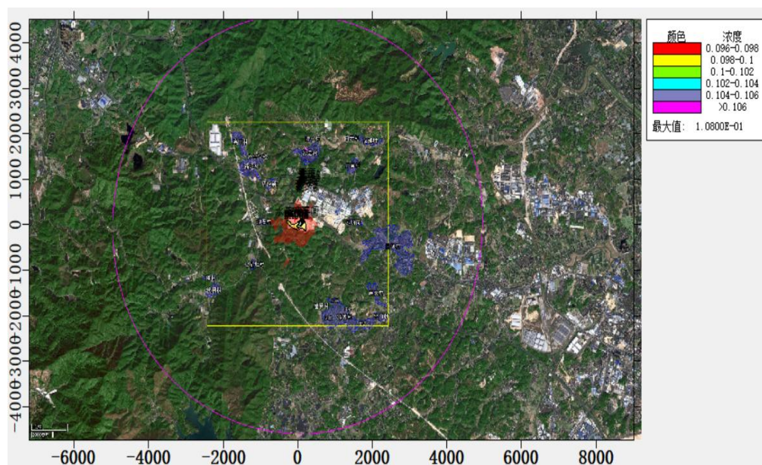
图 5.2.1-35 氨叠加后 1 小时浓度等值线图
