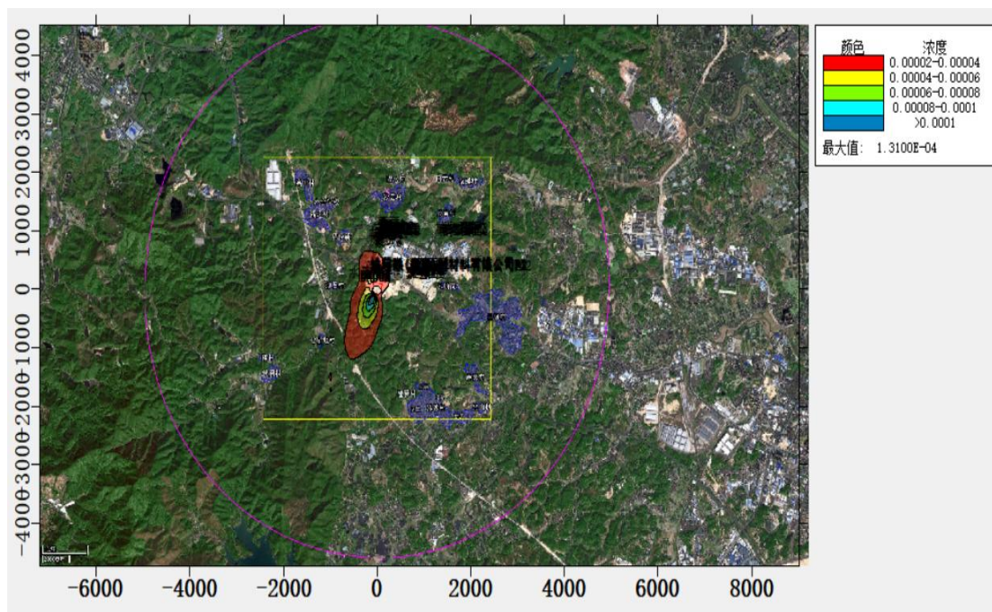
图 5.2.1-18 PM 2.5 年平均浓度等值线图
