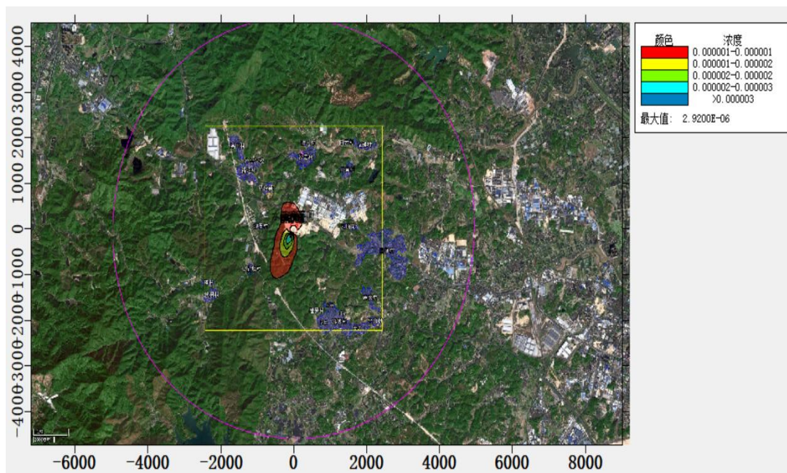
图 5.2.1-9 SO 2 年平均浓度等值线图
