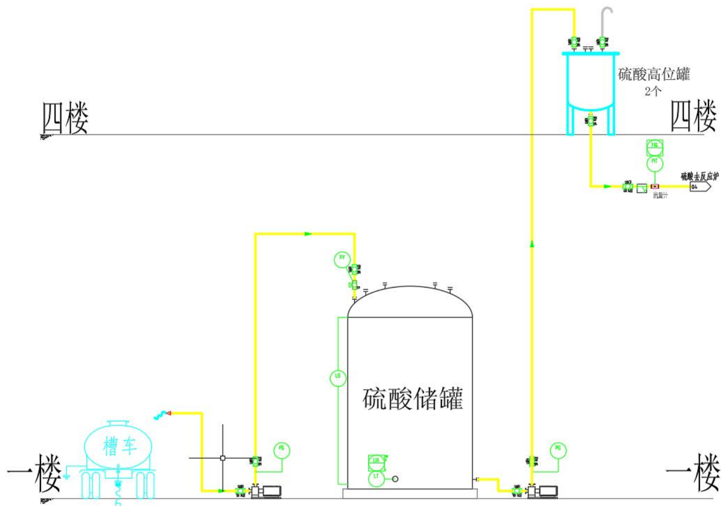
图 3.3-2 (1) 硫酸储罐与管道设备连接图
