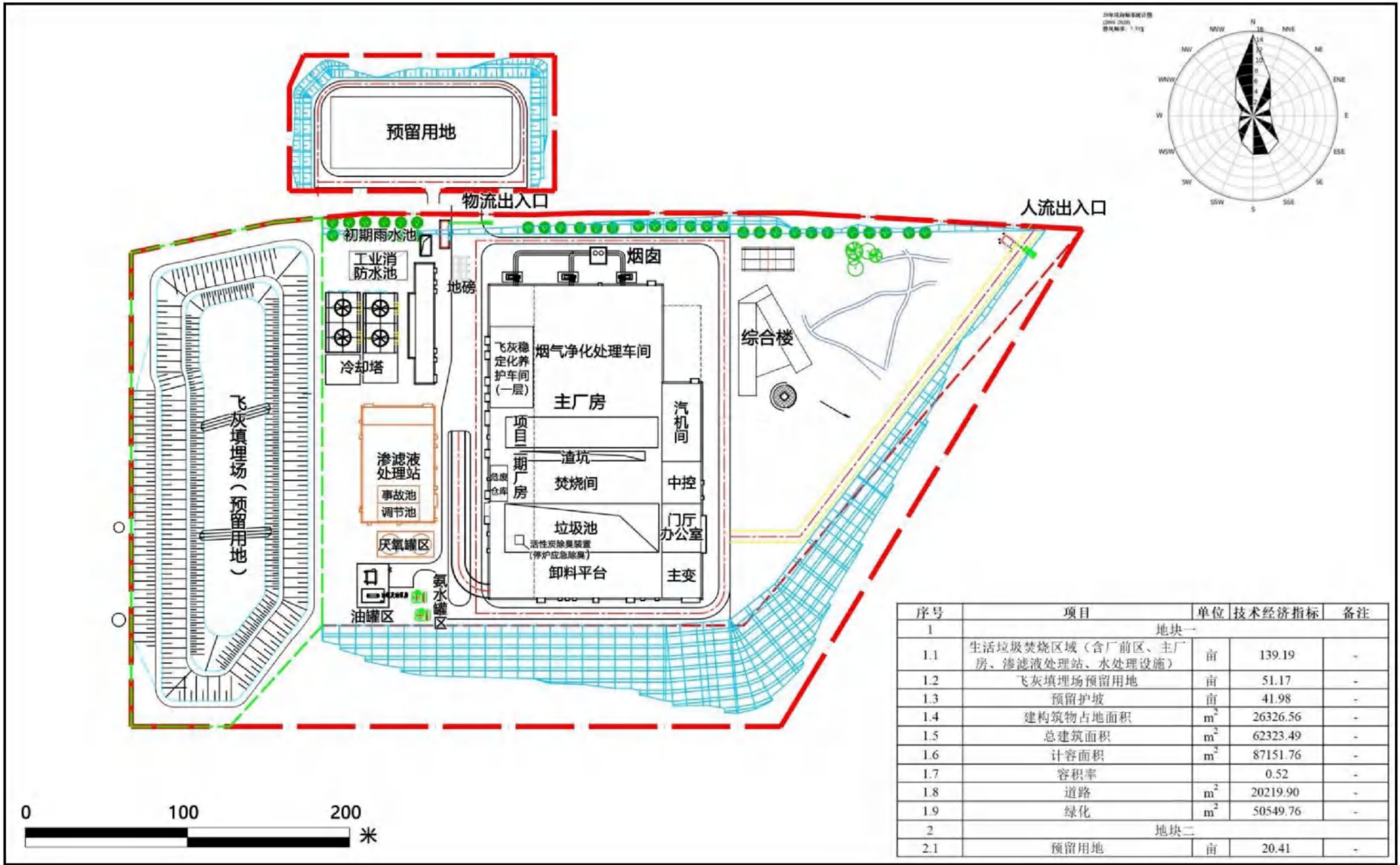
图 3.2-1 原项目环评总平面布置图
