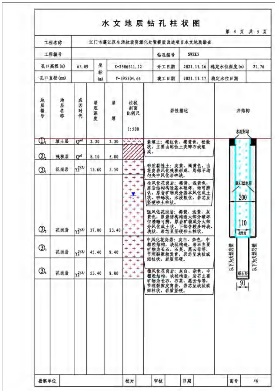
图 5.4-10 SWZK5 水文地质钻孔柱状图
