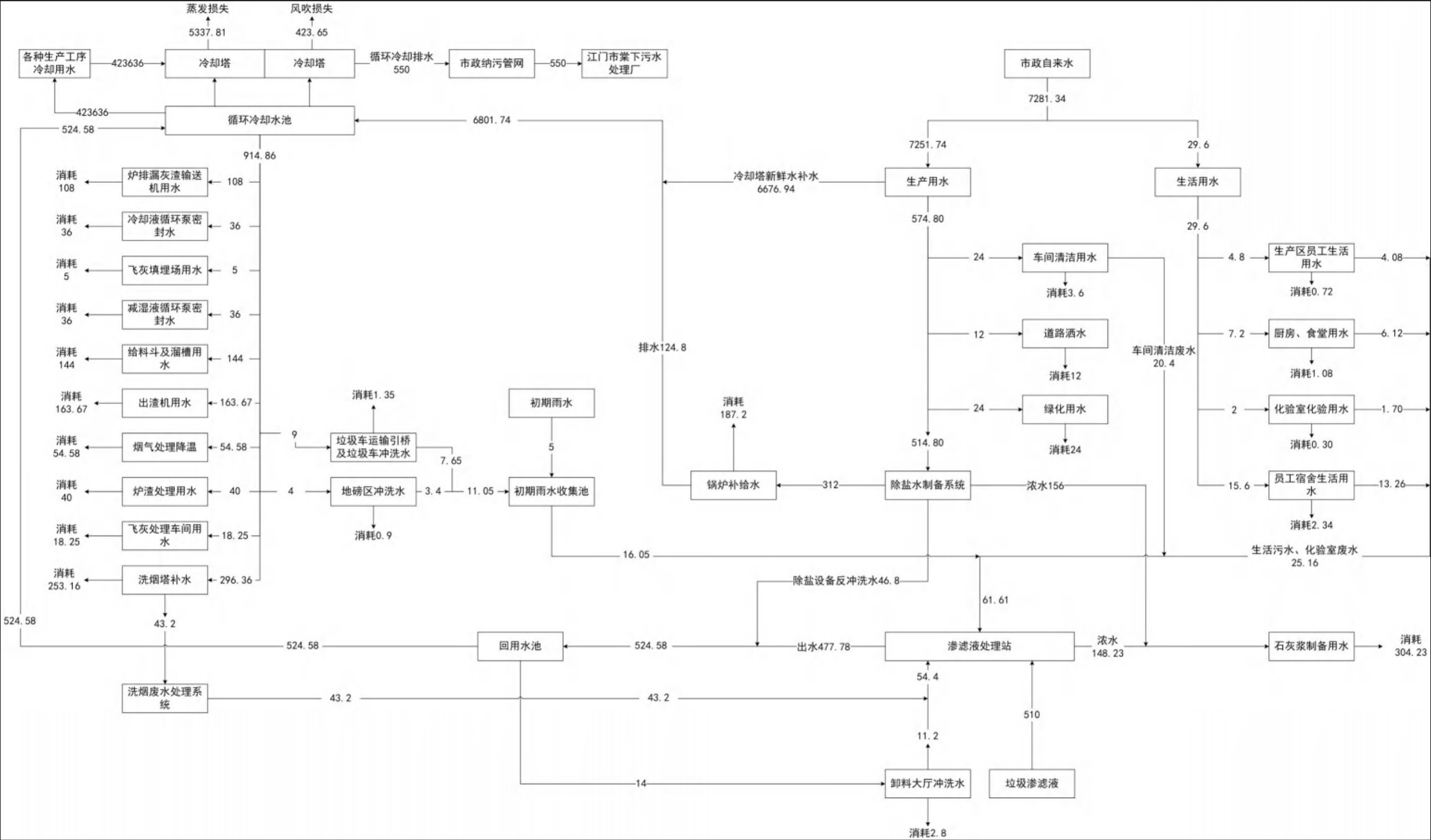
图 4.2-9 项目水平衡图（年平均）（单位 t/d）
