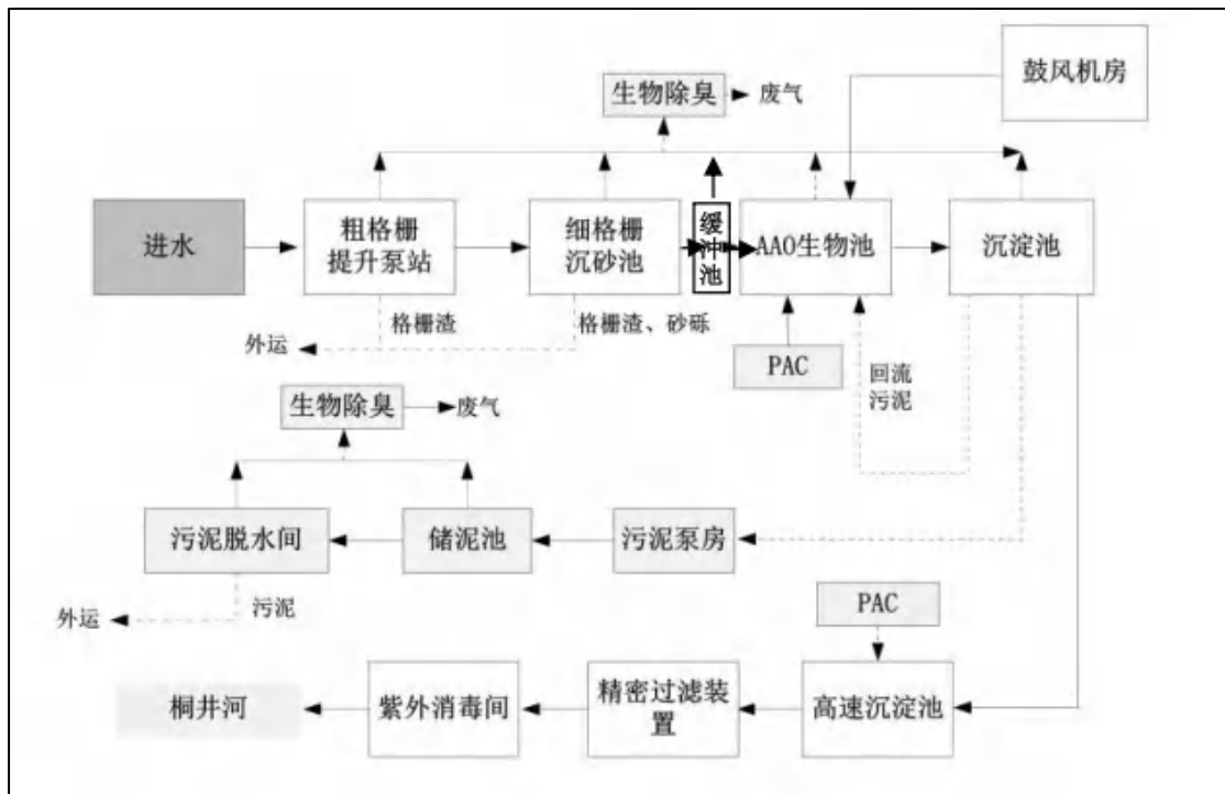
图 7.2-4 江门市棠下污水处理厂二期及扩建工程污水处理工艺流程图
