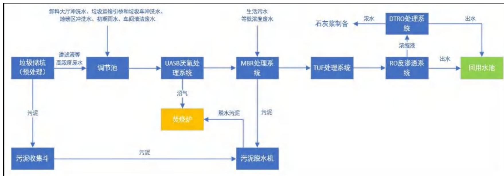
图 7.2-1 渗滤液处理系统工艺流程图
