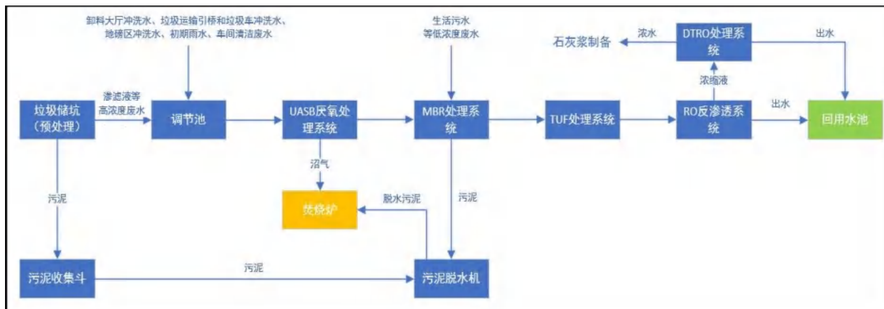
图 3.6-2 渗滤液处理系统工艺流程图
