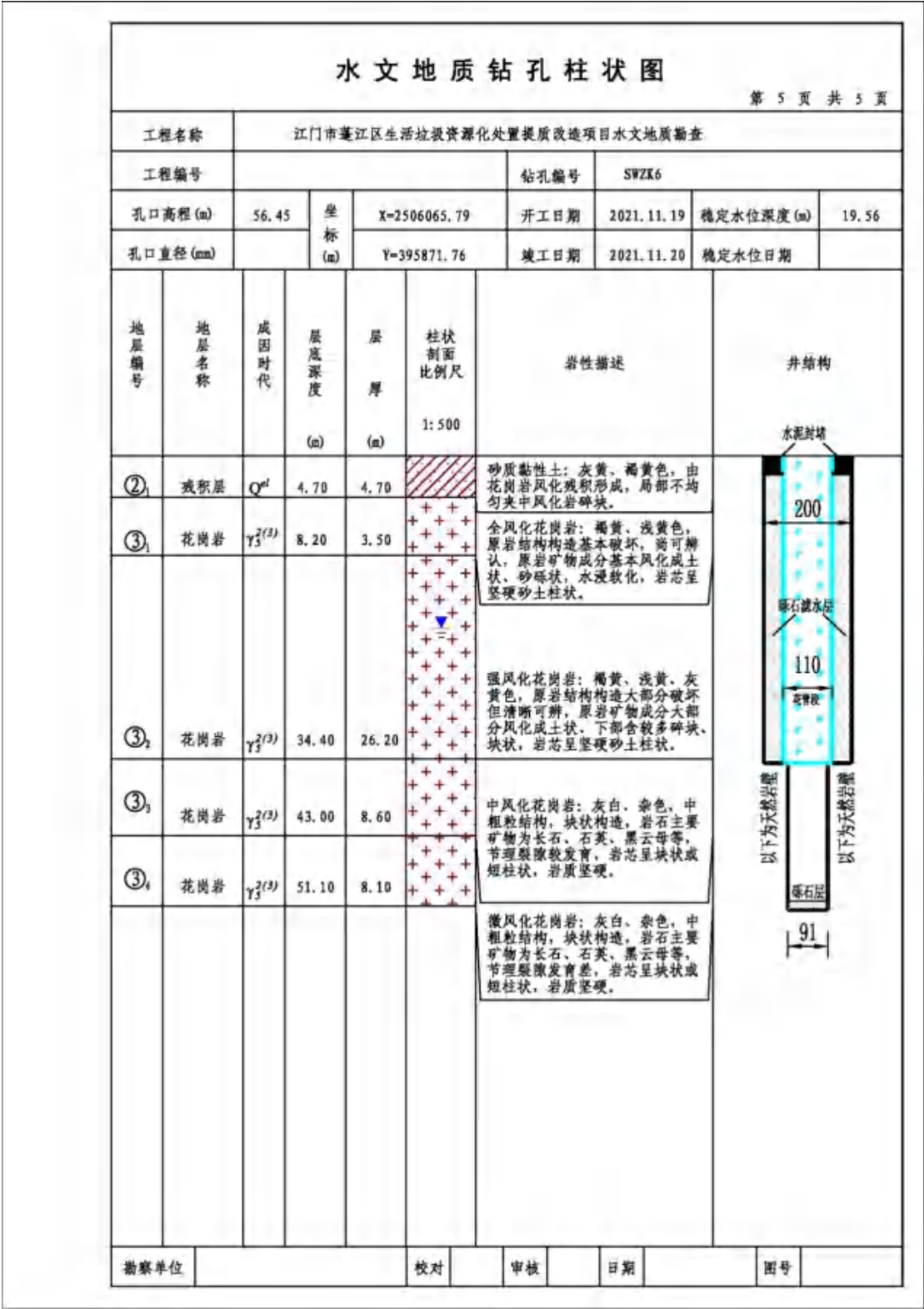
图 5.4-11 SWZK6 水文地质钻孔柱状图
