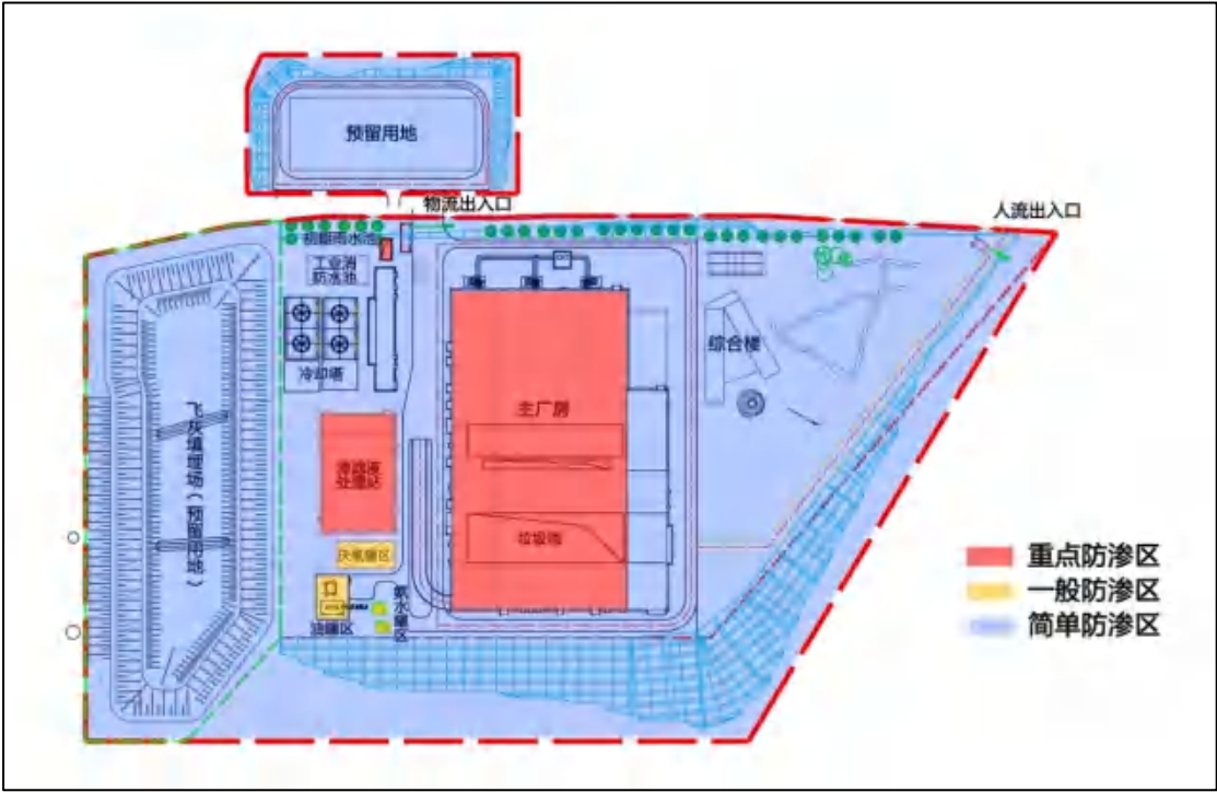
图 7.5-1 现有项目污染防治分区图
