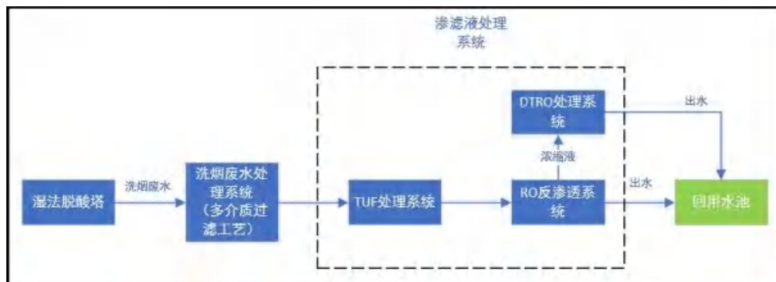
图 3.6-3 洗烟废水处理工艺流程图
