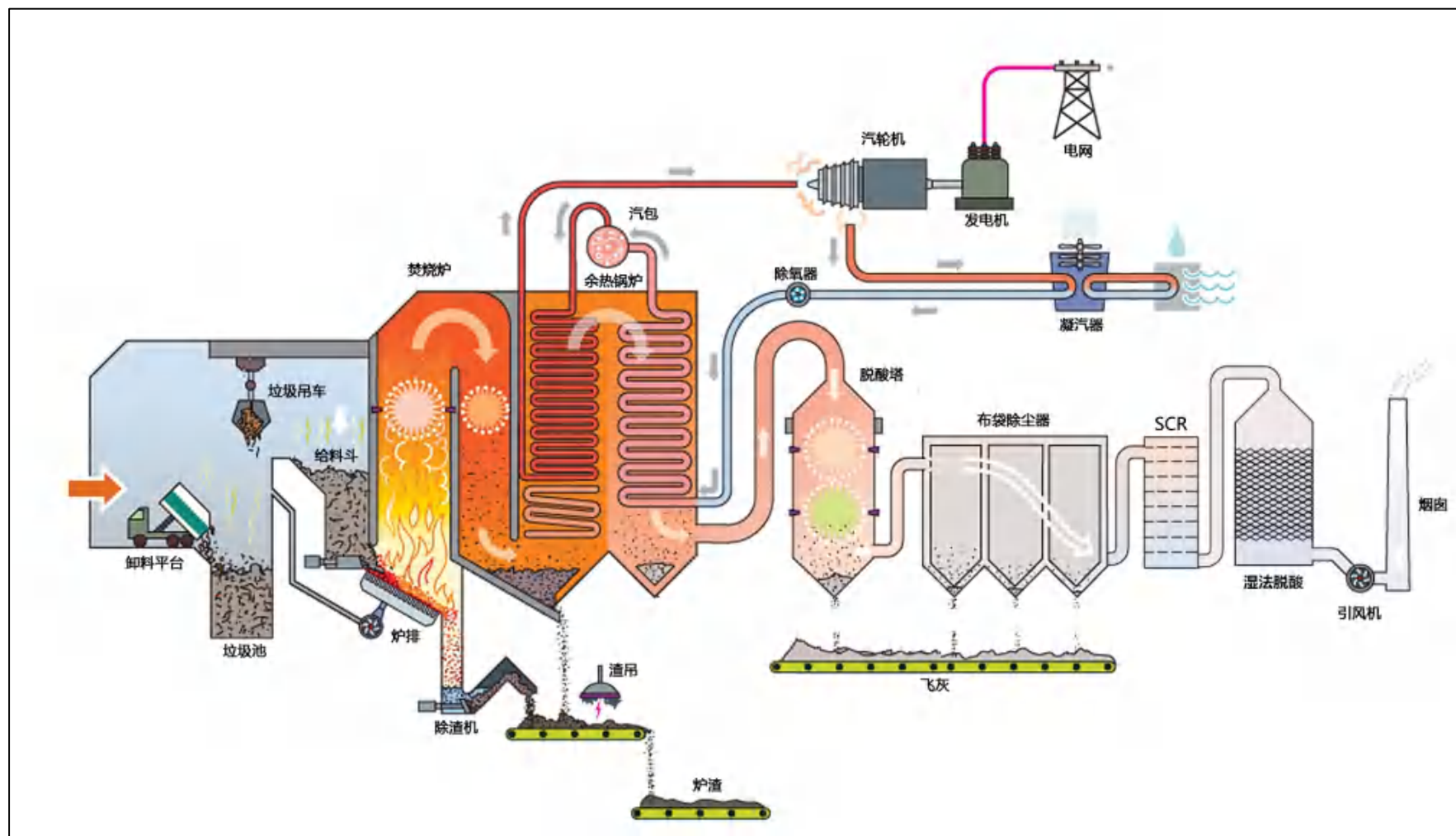
图 3.4-1 生活垃圾焚烧发电工艺流程图
