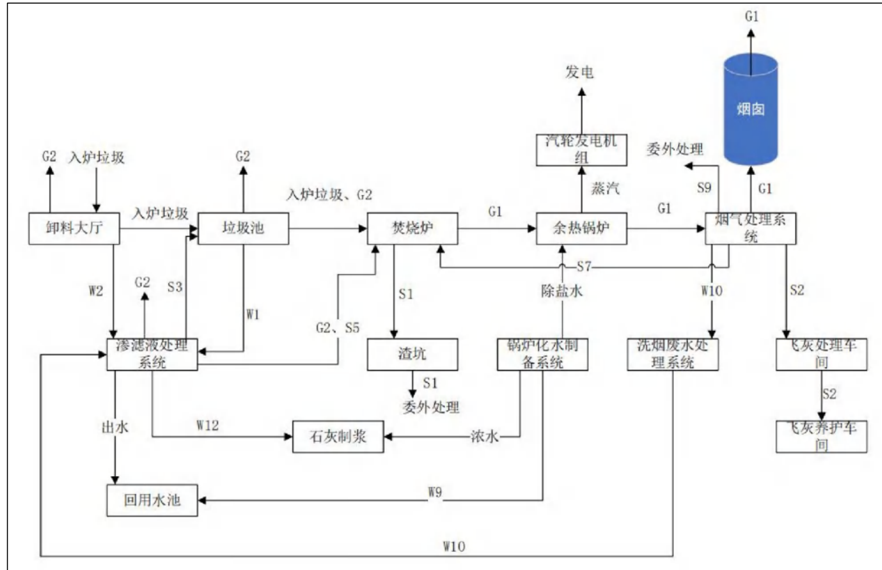
图 4.2-4 生产工艺流程及产污环节示意图
