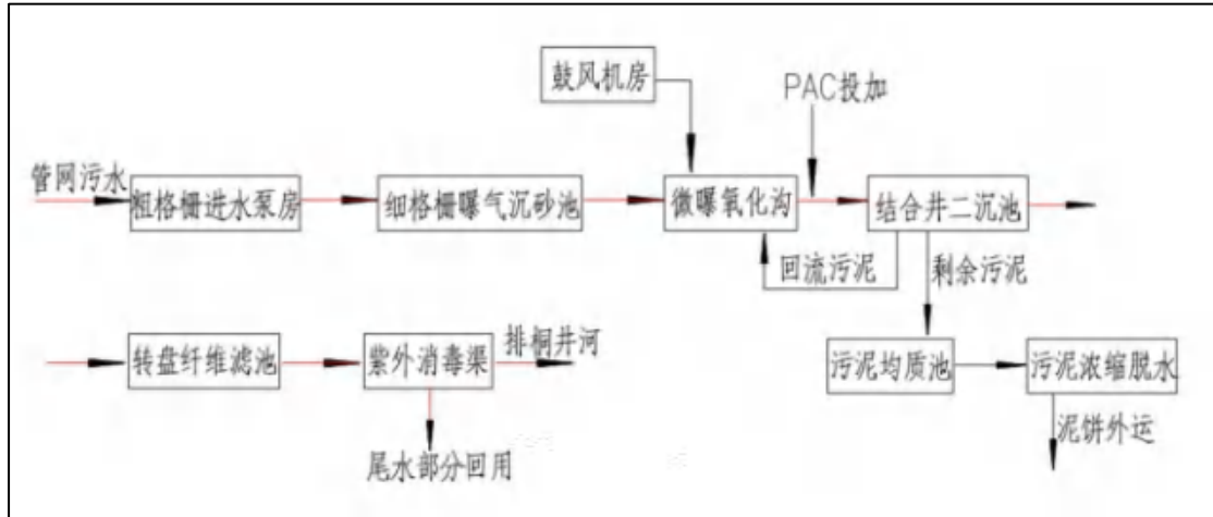
图 7.2-3 江门市棠下污水处理厂一期工程污水处理工艺流程图
