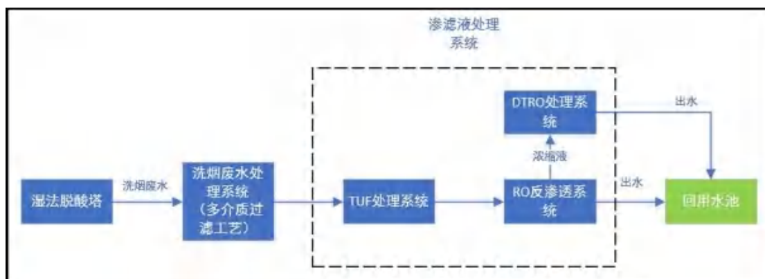
图 7.2-2 洗烟废水处理系统工艺流程图
