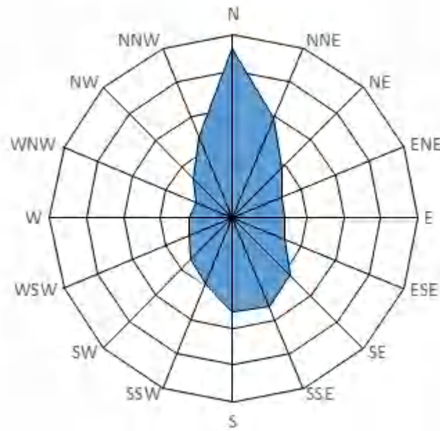
图 6.1-1 鹤山近 20 年风向玫瑰图（静风频率 7.33%）
