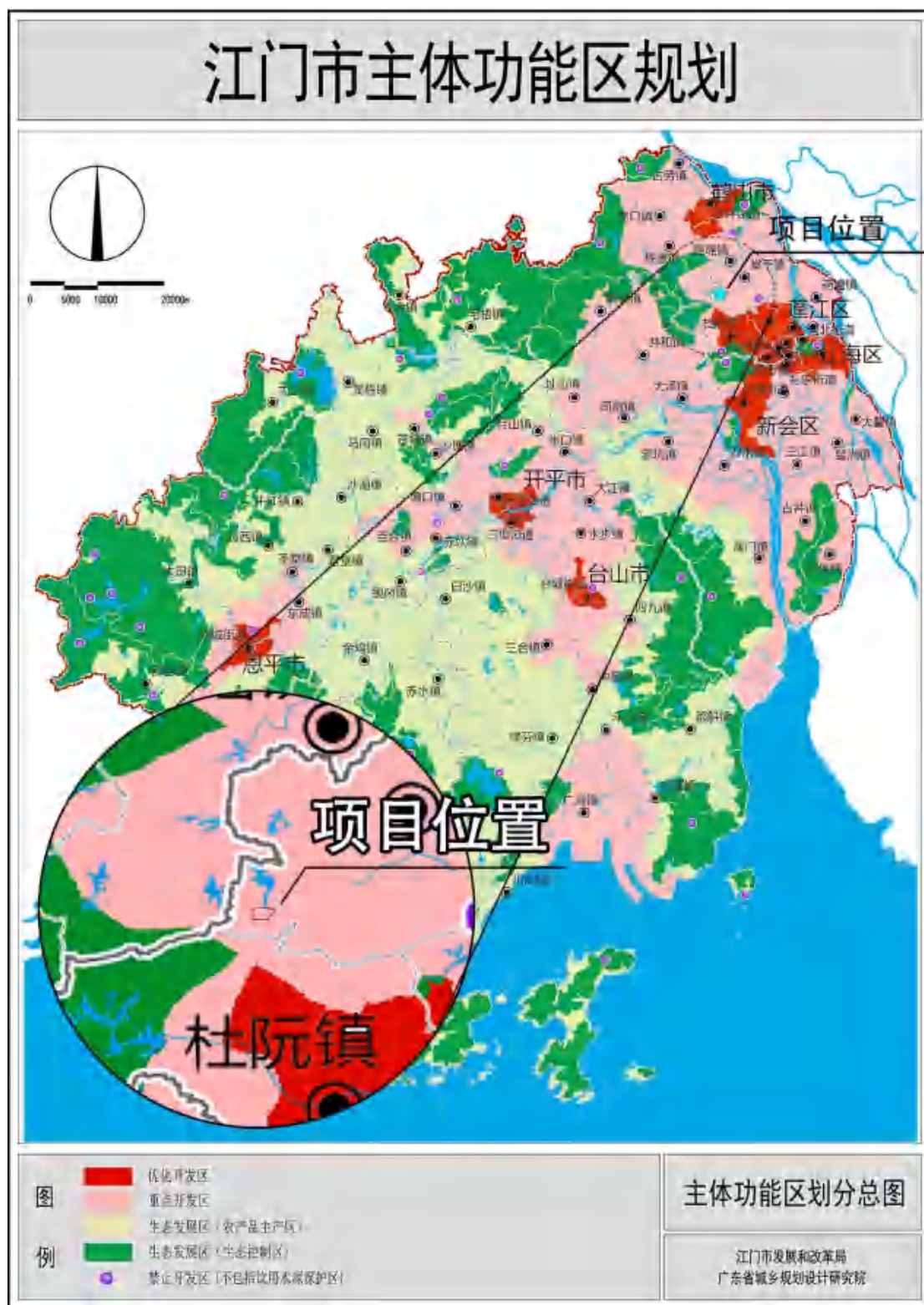
图 2.4-10 江门市主体功能区划图
