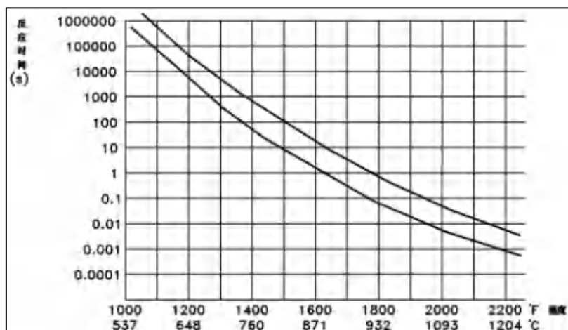
图 7.1-2 二噁英 (TCDD) 分解 99.99%所需时间
