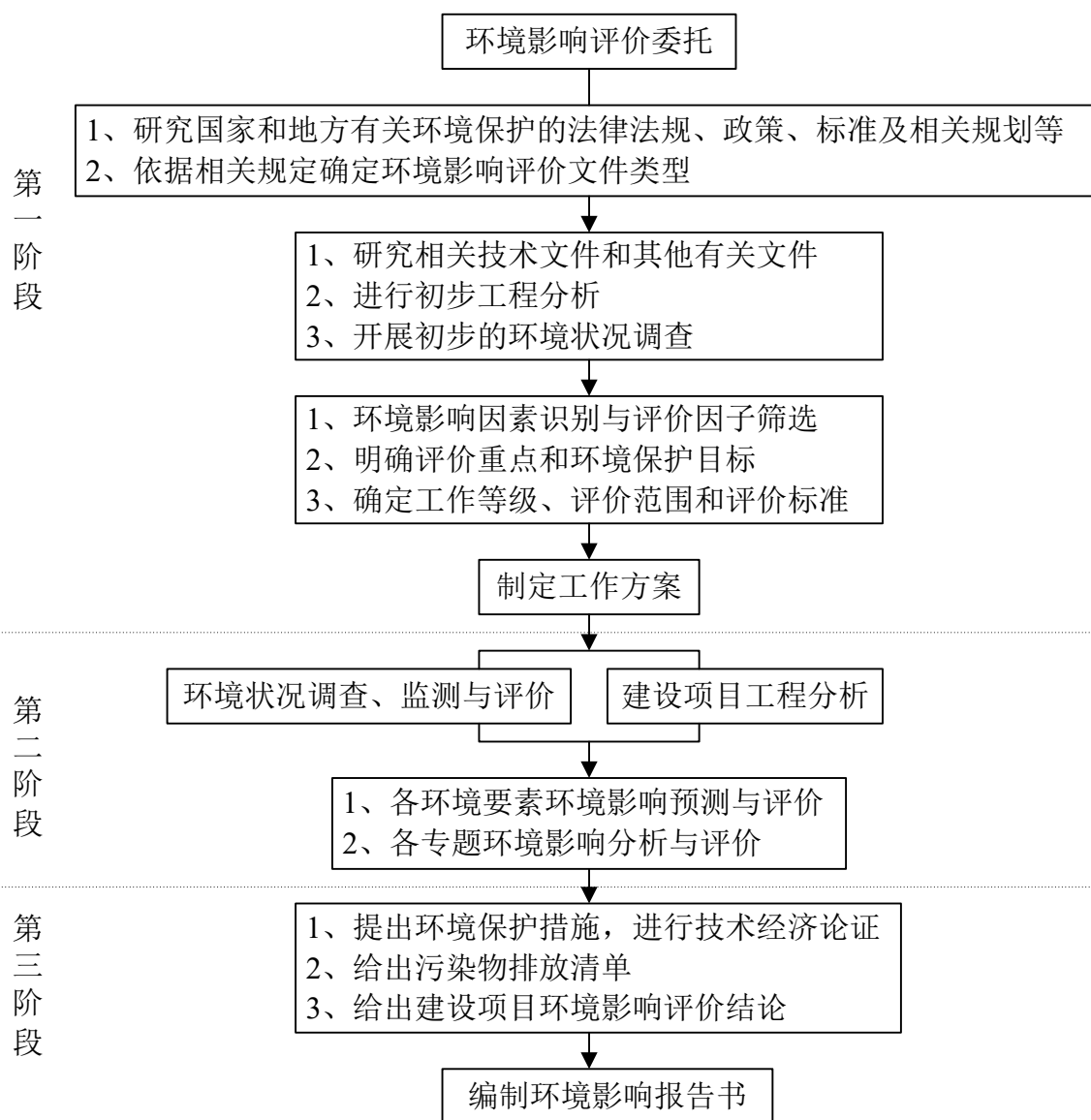
图 1.2-1 环境影响评价工作过程
