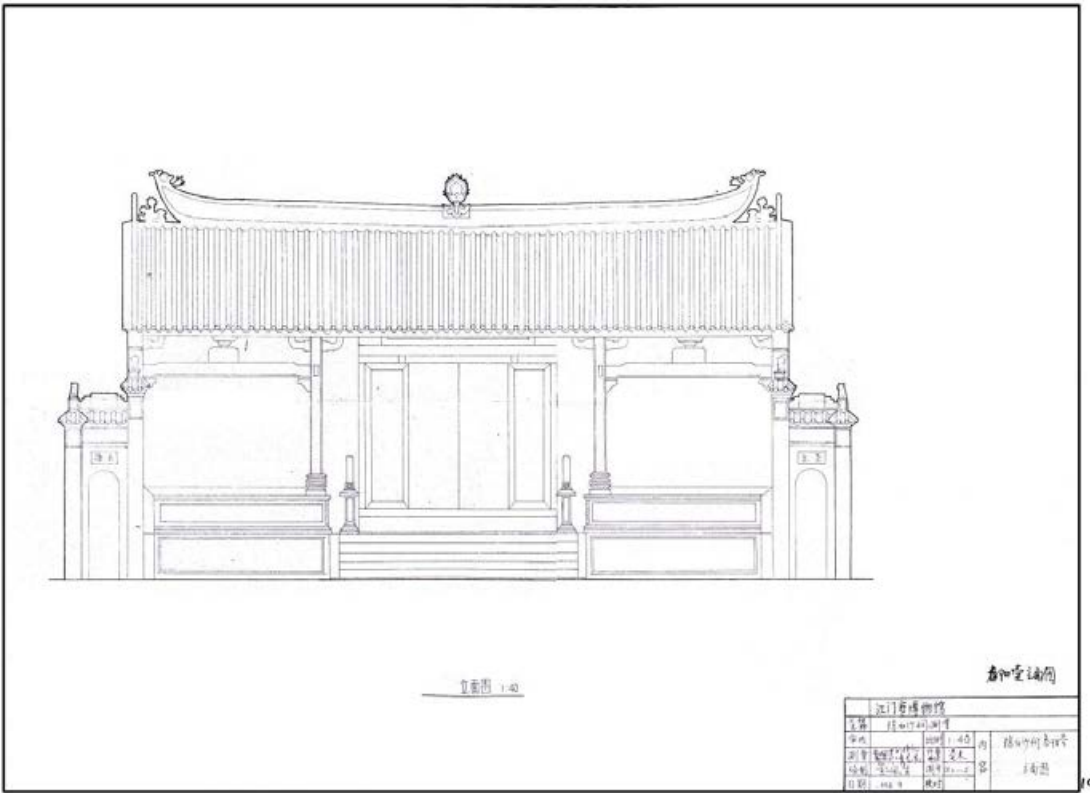
附件五：1、陈白沙祠测绘图纸 1994 年 9 月—春阳堂正立面
