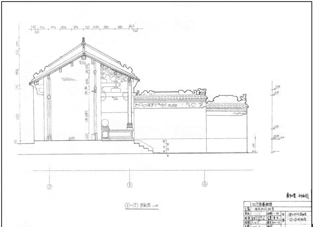
附件五：1、陈白沙祠测绘图纸 1994 年 9 月-春阳堂剖面
