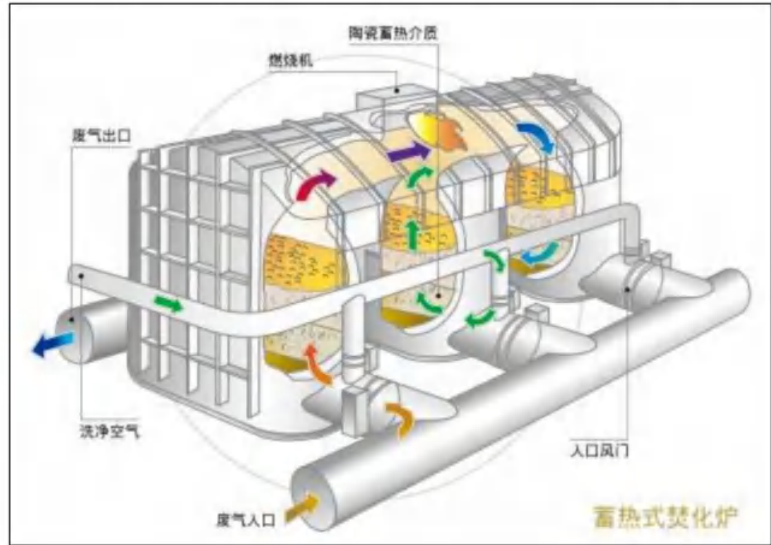
图 9.1-2 RTO 系统示意图
