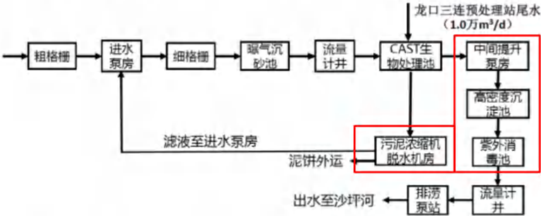
图 7.1-2 鹤山市第二污水处理厂废水处理工艺流程图（红框内为提标改造工程）
