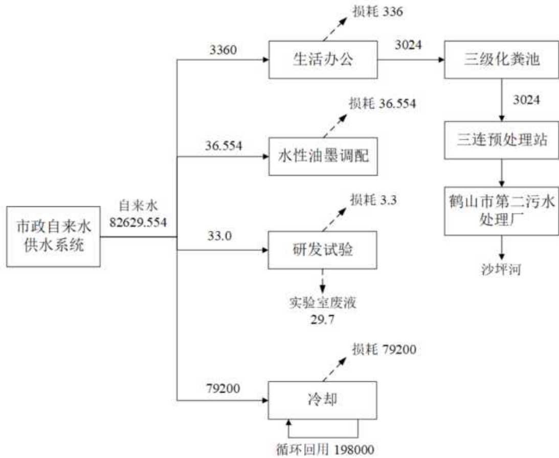
图 4.2-1 项目水平衡图（单位：m³/a）
