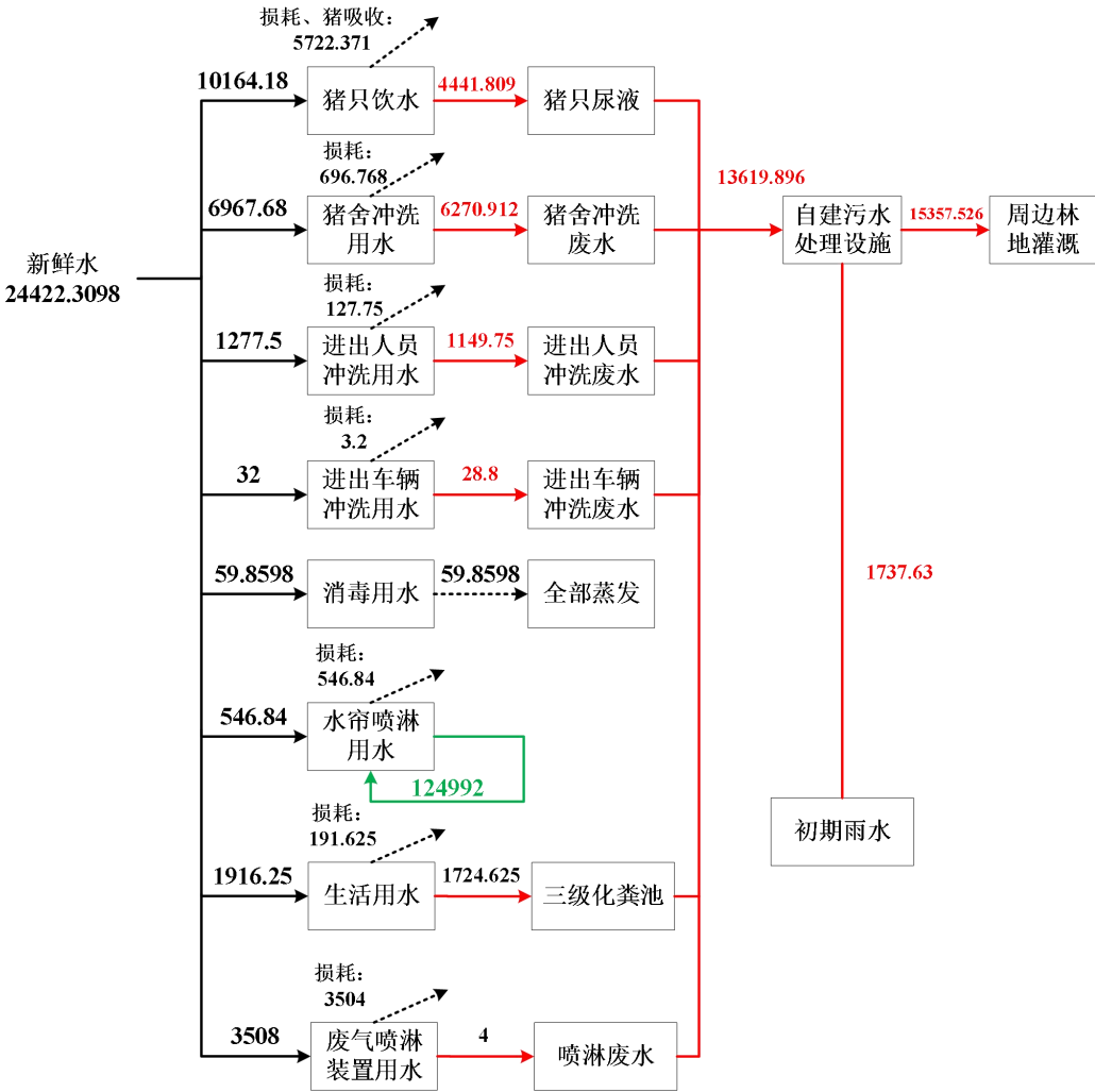
图3.4-1 项目水平衡图 单位： \text{m}^3/\text{a}
