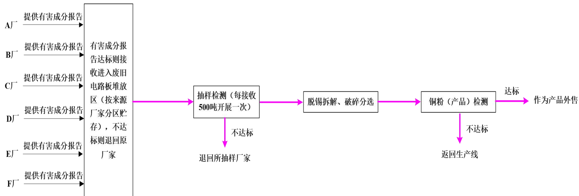
图 3.1-8 含元器件废电路板检验、管理流程示意图
