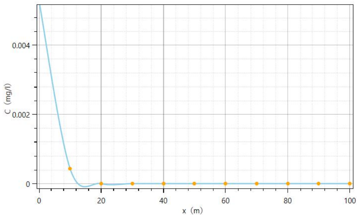
图 5.6-3 污水池渗漏 100d 后，下游不同距离的镍离子浓度分布
