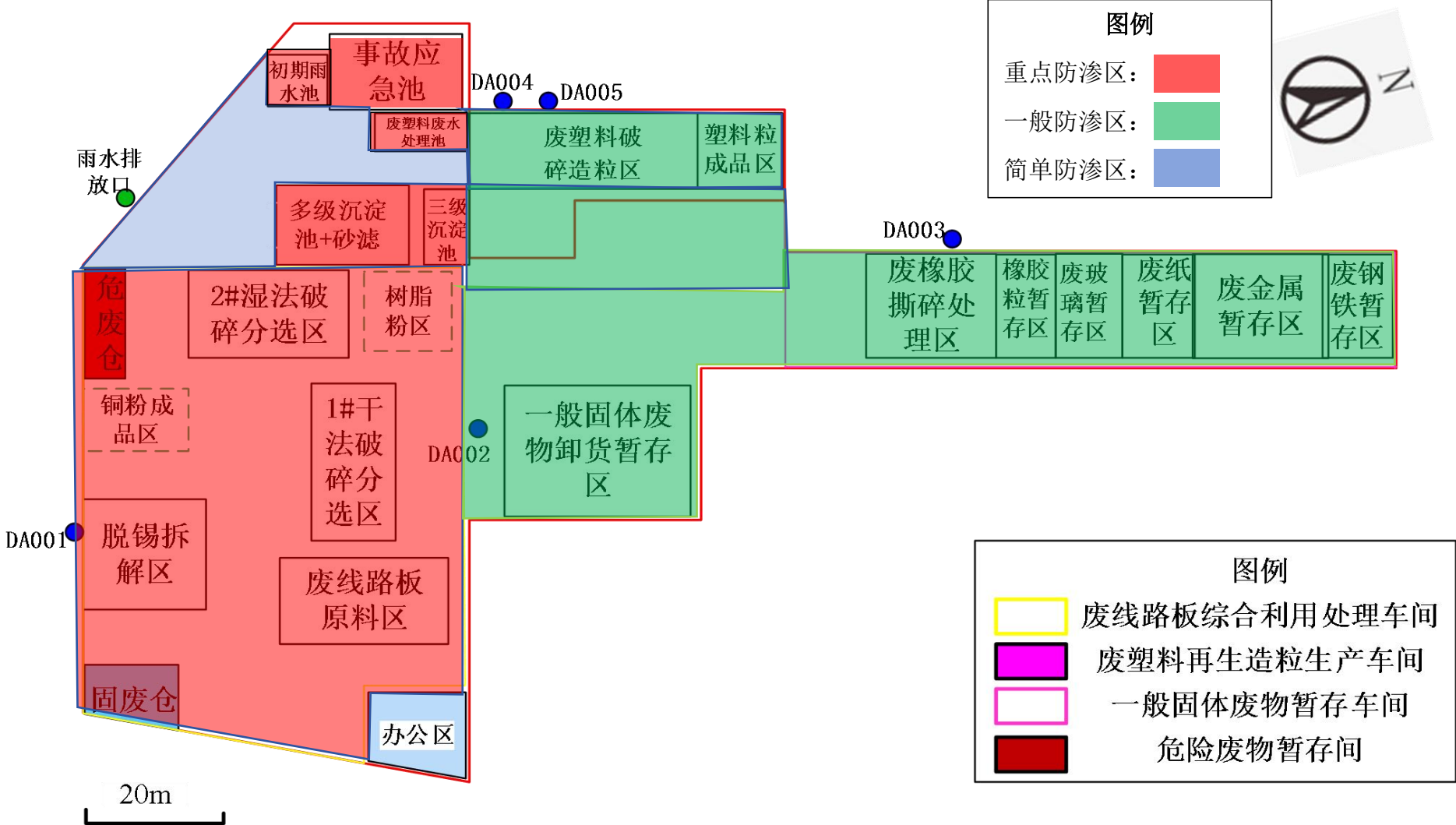
图 7.5-1 项目项目地下水污染防治分区图
