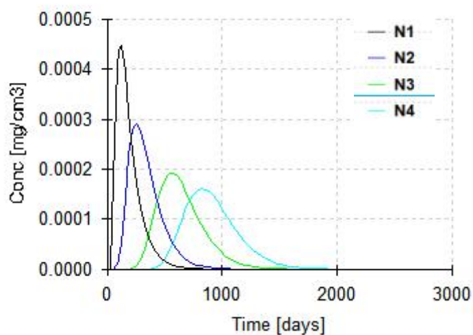
图 5.7-1 观测点镍浓度与时间曲线图（N1 为 0.5m 深度、N2 为 1m 深度，N3 为 2m，N4 为 3m）
