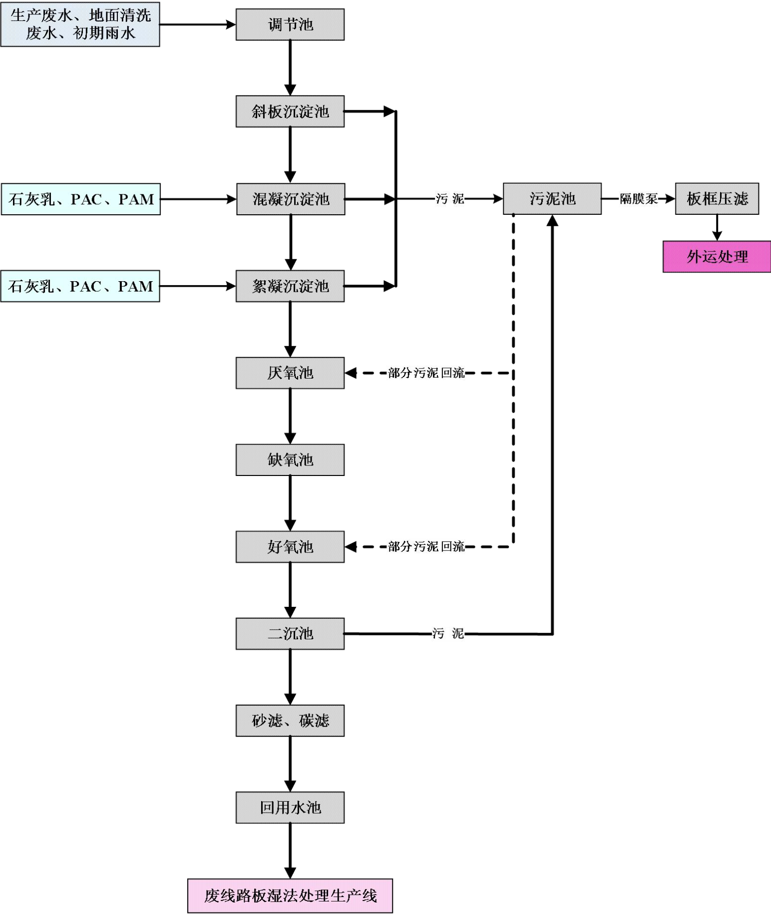
图 7.2-2 自建（废线路板湿法线）废水治理设施工艺流程图
