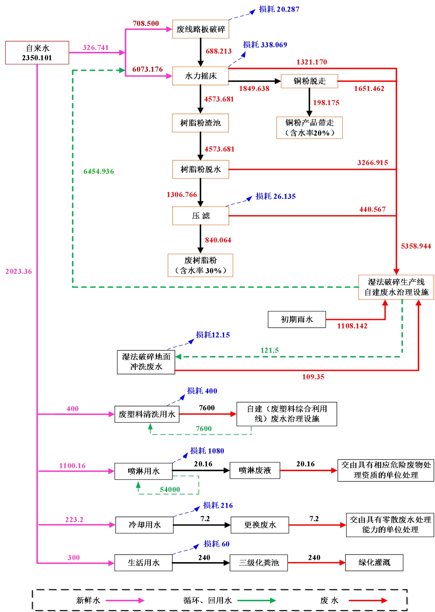
图 3.3-4 全厂水平衡图 (单位: 吨/年)
