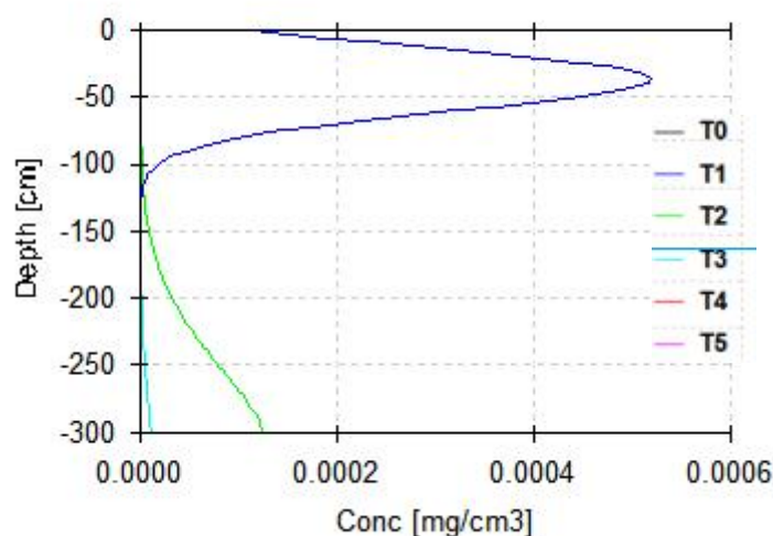
图 5.7-2 观测点镍浓度与深度曲线图（T1 为 100d、T2 为 1000d，T3 为 1500d，T4 为 2000d，T5 为 3000d）
