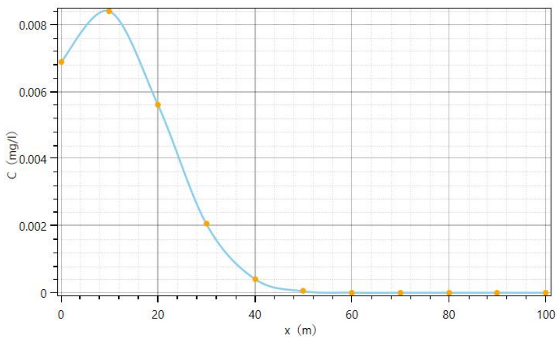
图 5.6-2 污水池渗漏 1000d 后，下游不同距离的铜离子浓度分布
