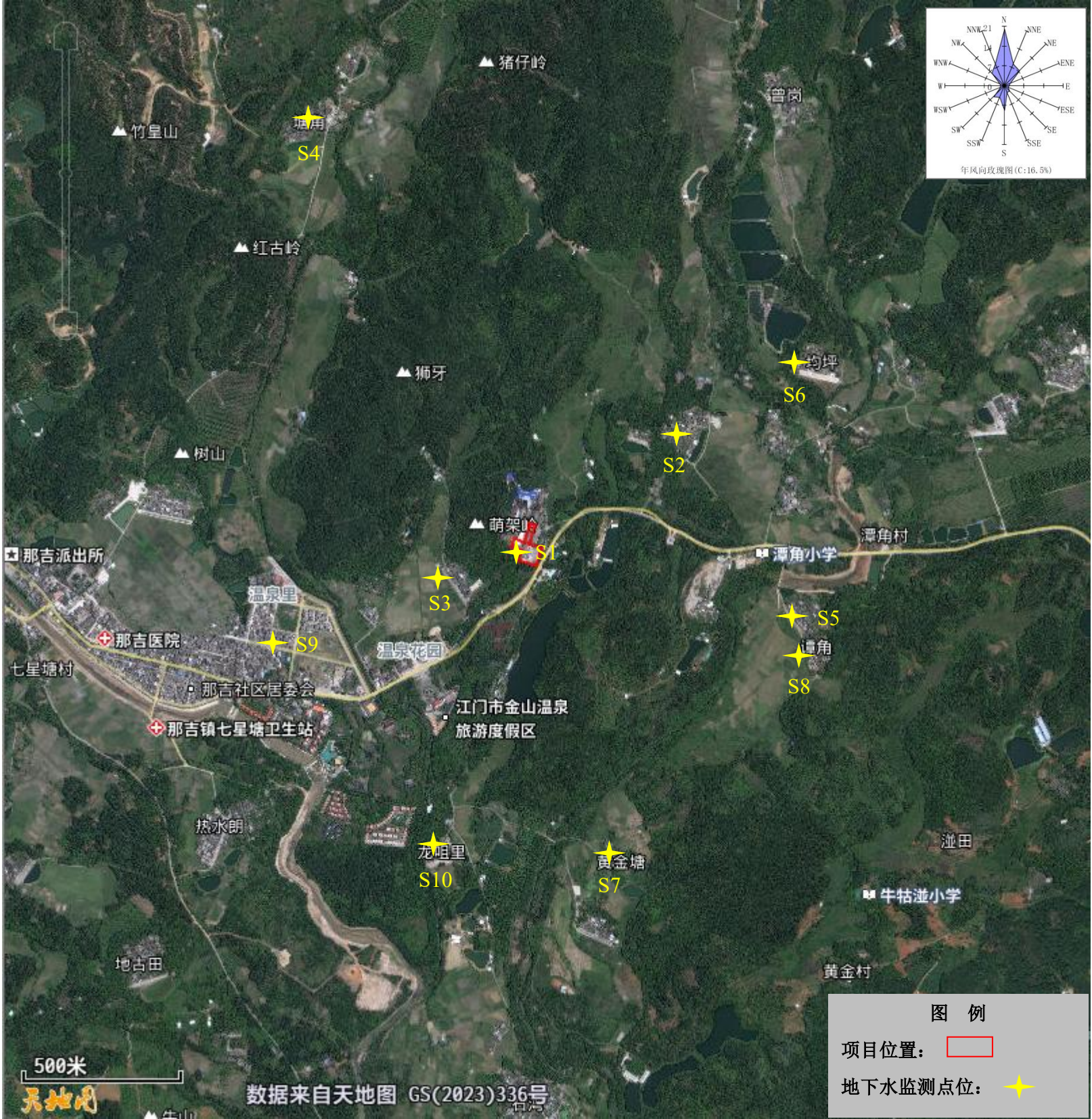
图 4.3-1 项目地下水监测断面分布图
