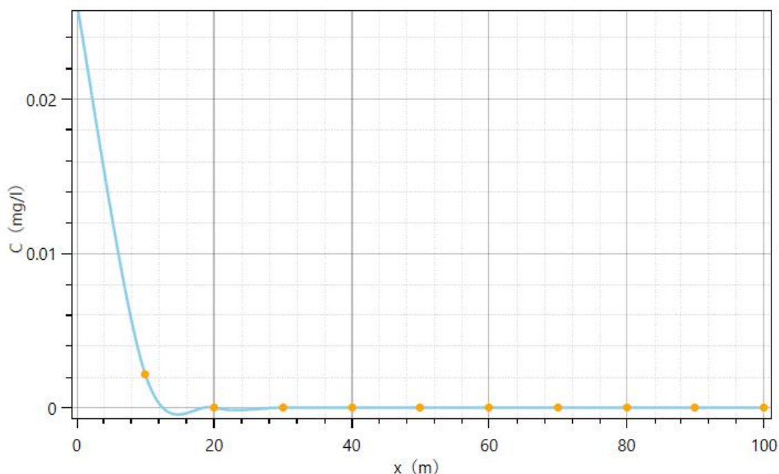
图 5.6-1 污水池渗漏 100d 后, 下游不同距离的铜离子浓度分布
