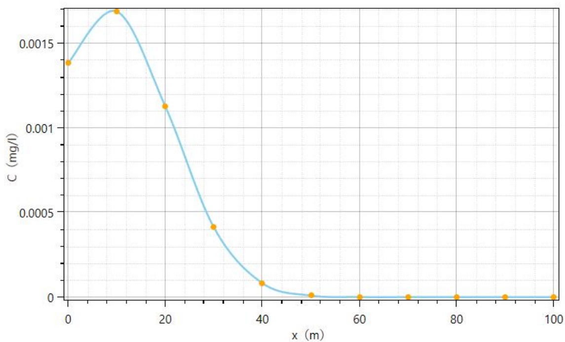
图 5.6-4 污水池渗漏 1000d 后，下游不同距离的镍离子浓度分布
