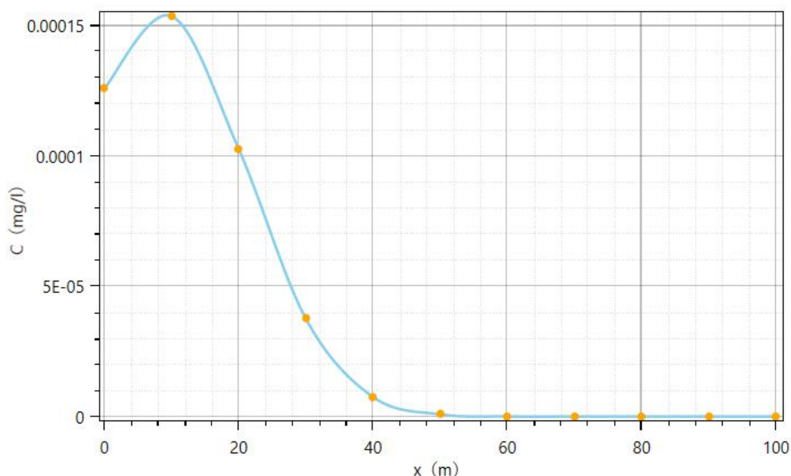
图 5.6-8 污水池渗漏 1000d 后，下游不同距离的铅离子浓度分布
