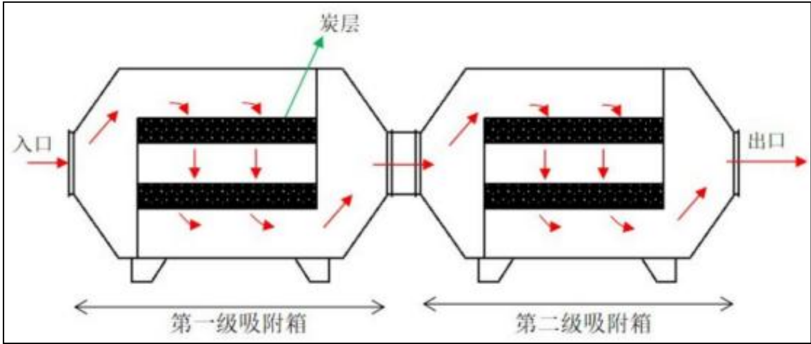
图 7.1-1 活性炭吸附设备原理示意图
