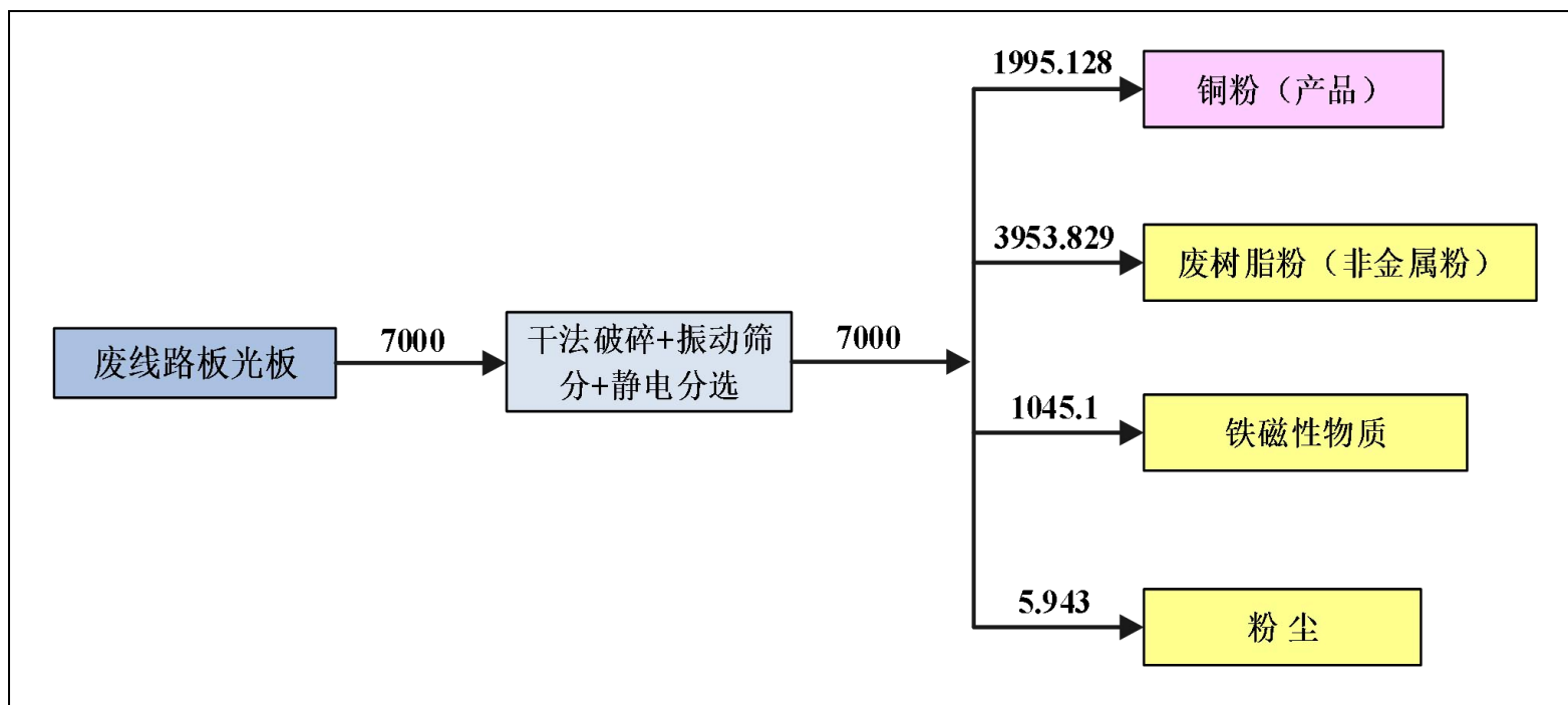
图 3.3-2 干法破碎分选处理生产线物料平衡图 (单位: t/a)
