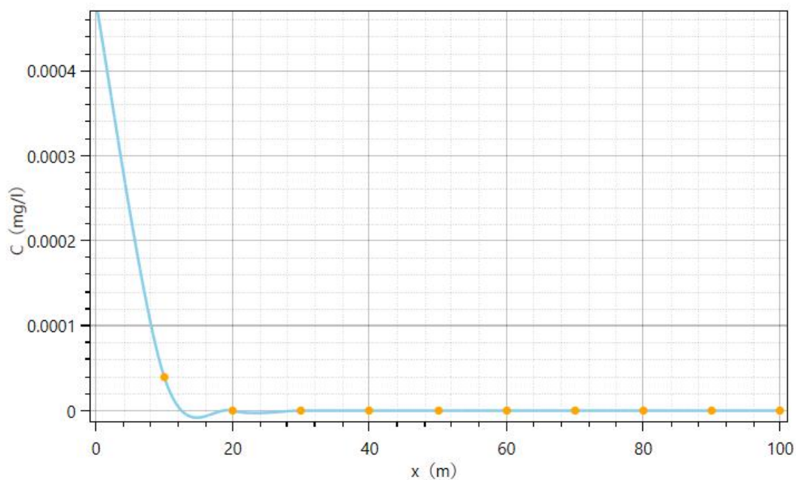
图 5.6-6 污水池渗漏 1000d 后，下游不同距离的锰离子浓度分布
