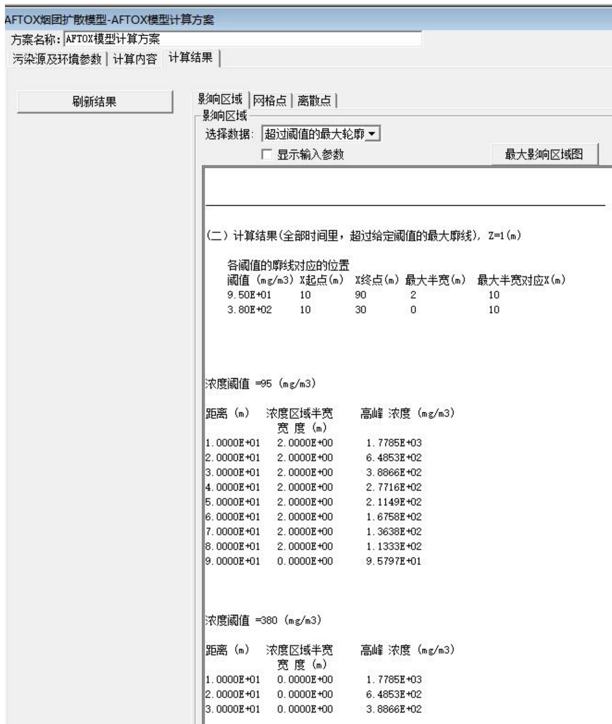
图6.4-1 最不利气象下, 下风向不同距离处CO(泄漏)的最大浓度值
