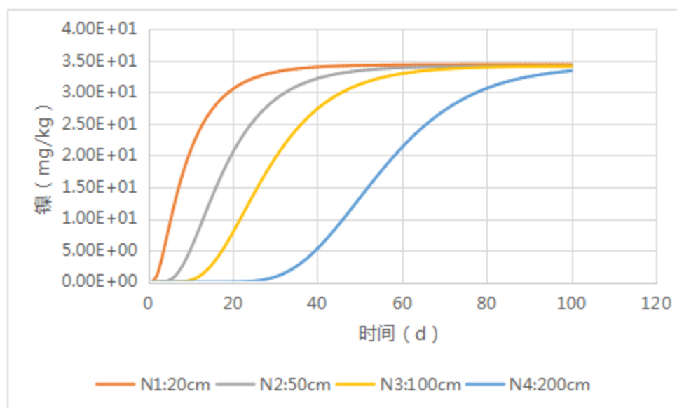
图 7.7-4 总镍浓度不同深度随时间变化曲线图
