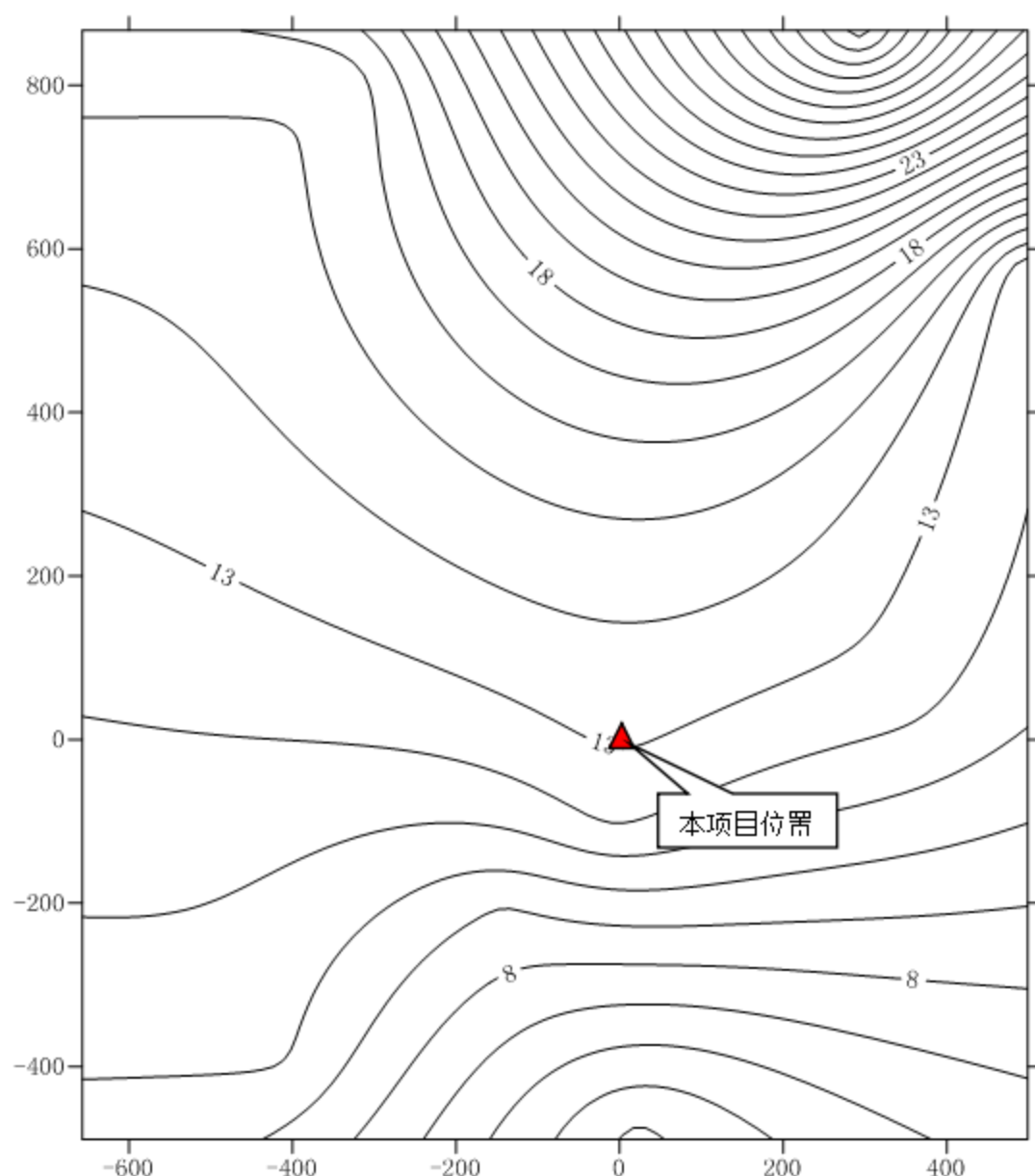
图 7.4-3 项目附近地下水等水位线图 (单位: m)
