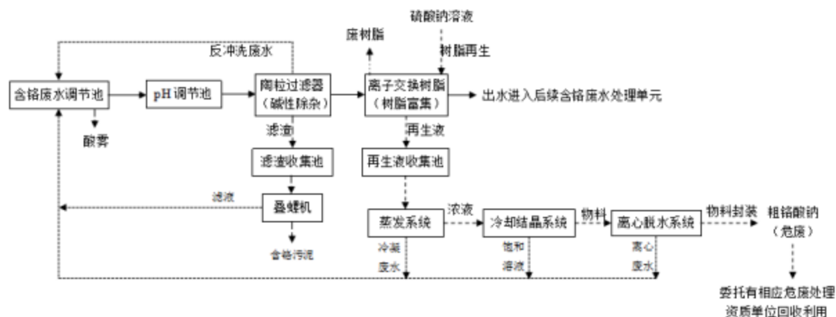
图 7.3-5 含铬废水预处理工艺流程图
