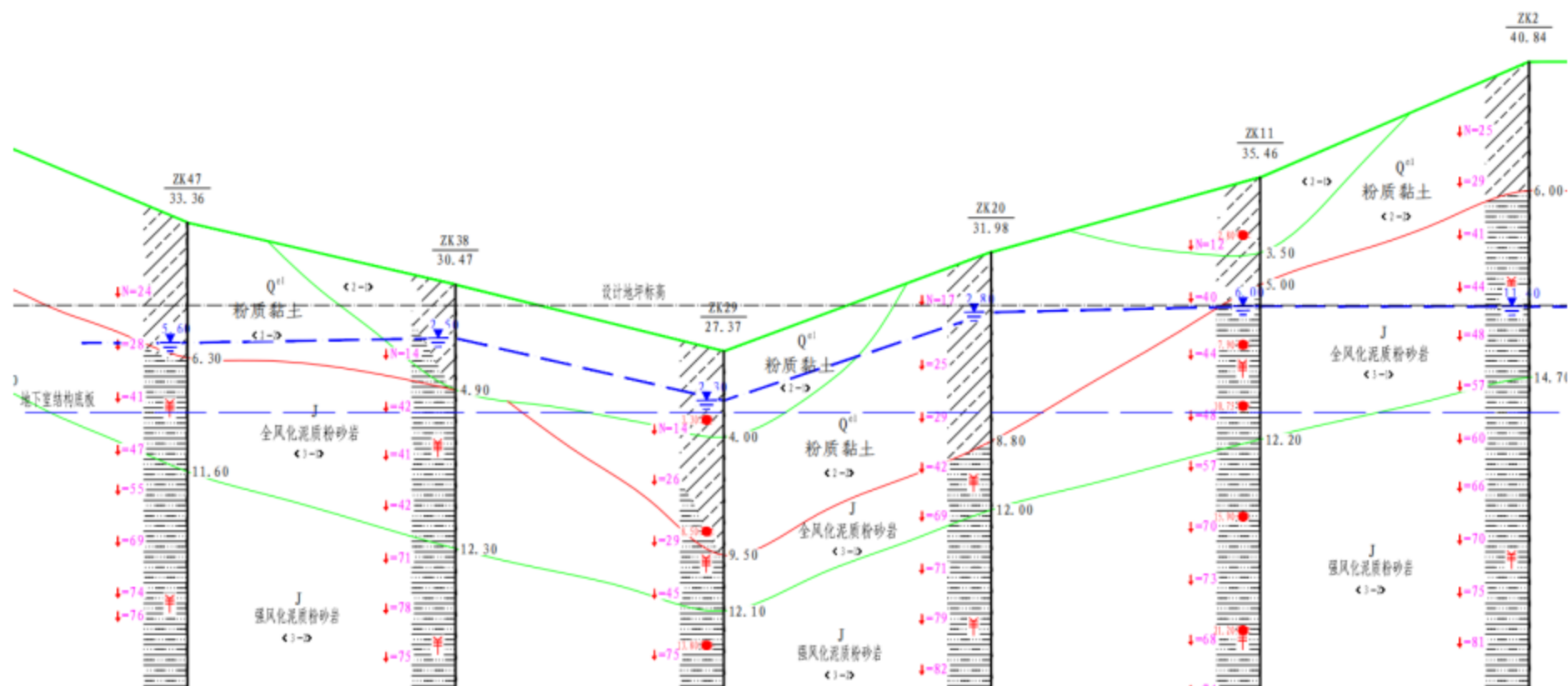
图 7.4.2 场地典型断面工程地质剖面
