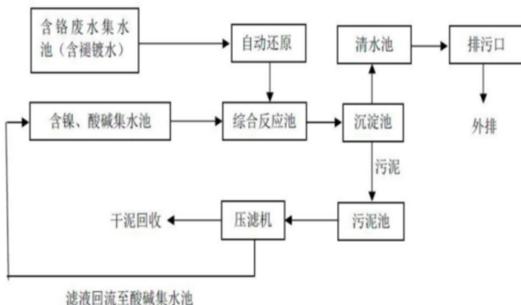
图 4.2-3 污水处理工艺流程图
