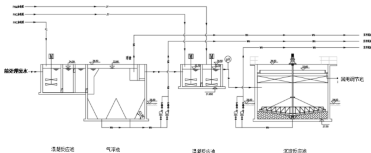
图 7.3-3 前处理废水预处理工艺流程图
