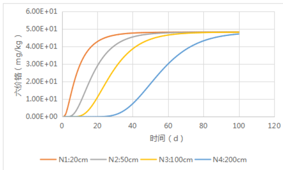
图 7.7-3 六价铬浓度不同深度随时间变化曲线图
