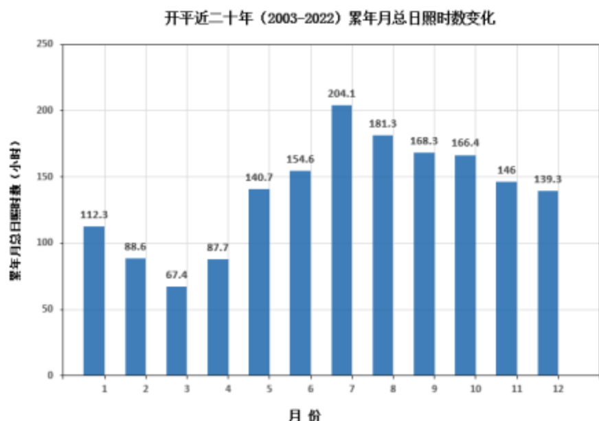
图 7.2-8 开平 (2003-2022) 月日照时数统计图 (单位: 小时)
