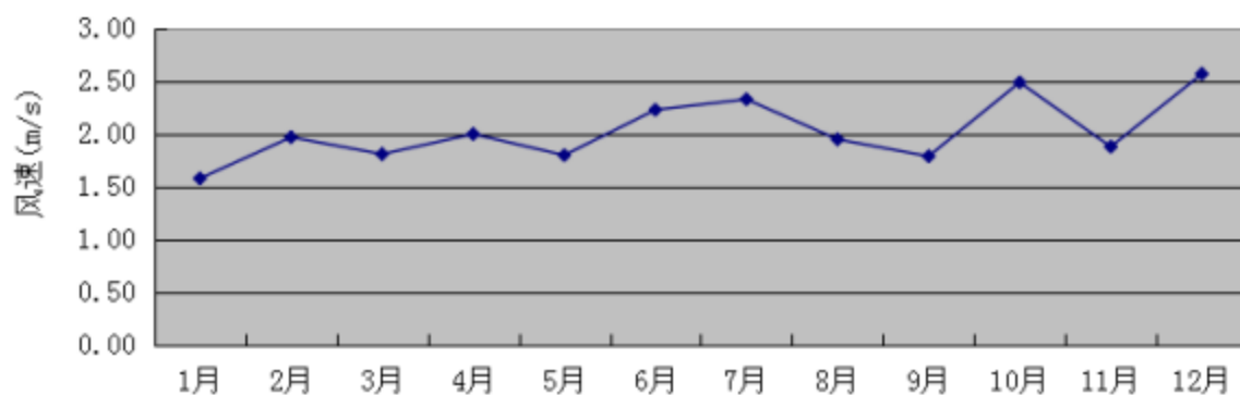
图 7.2-13 项目所在区域 2022 年平均风速月变化图
