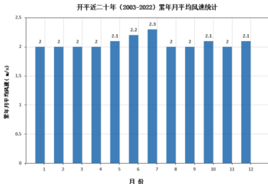
图 7.2-2 开平 (2003-2022) 月平均风速 (单位: m/s)
