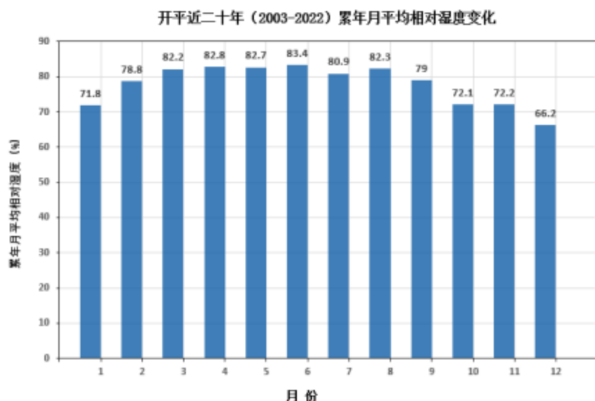
图 7.2-10 开平 (2003-2022) 月平均相对湿度统计结果 (纵轴为百分比)
