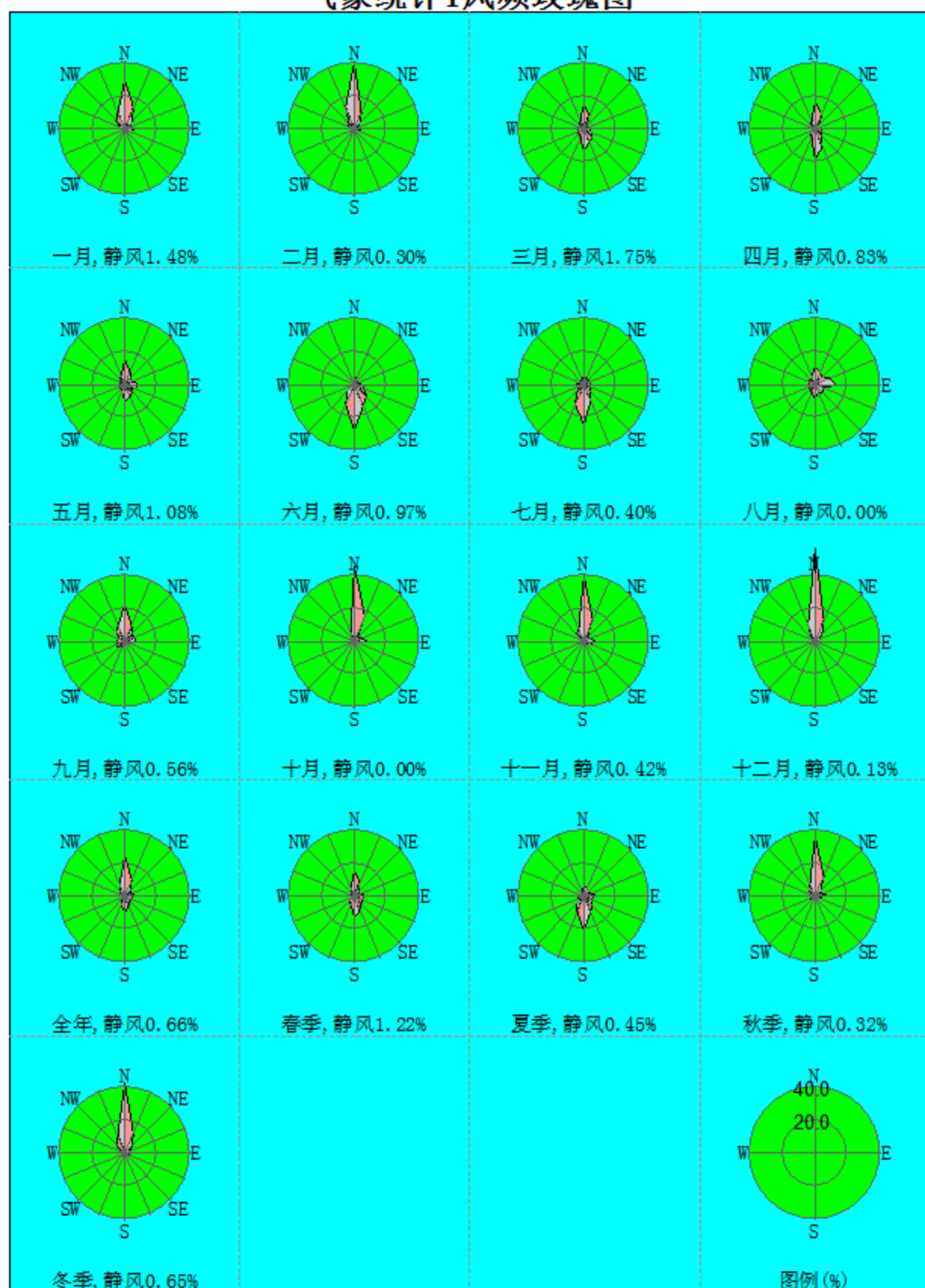
图 7.2-15 项目所在区域 2022 年各季及年平均风频图
