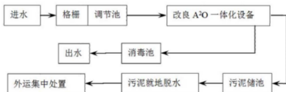
图 7.3-1 开平市月山镇污水处理厂污水处理工艺流程图
