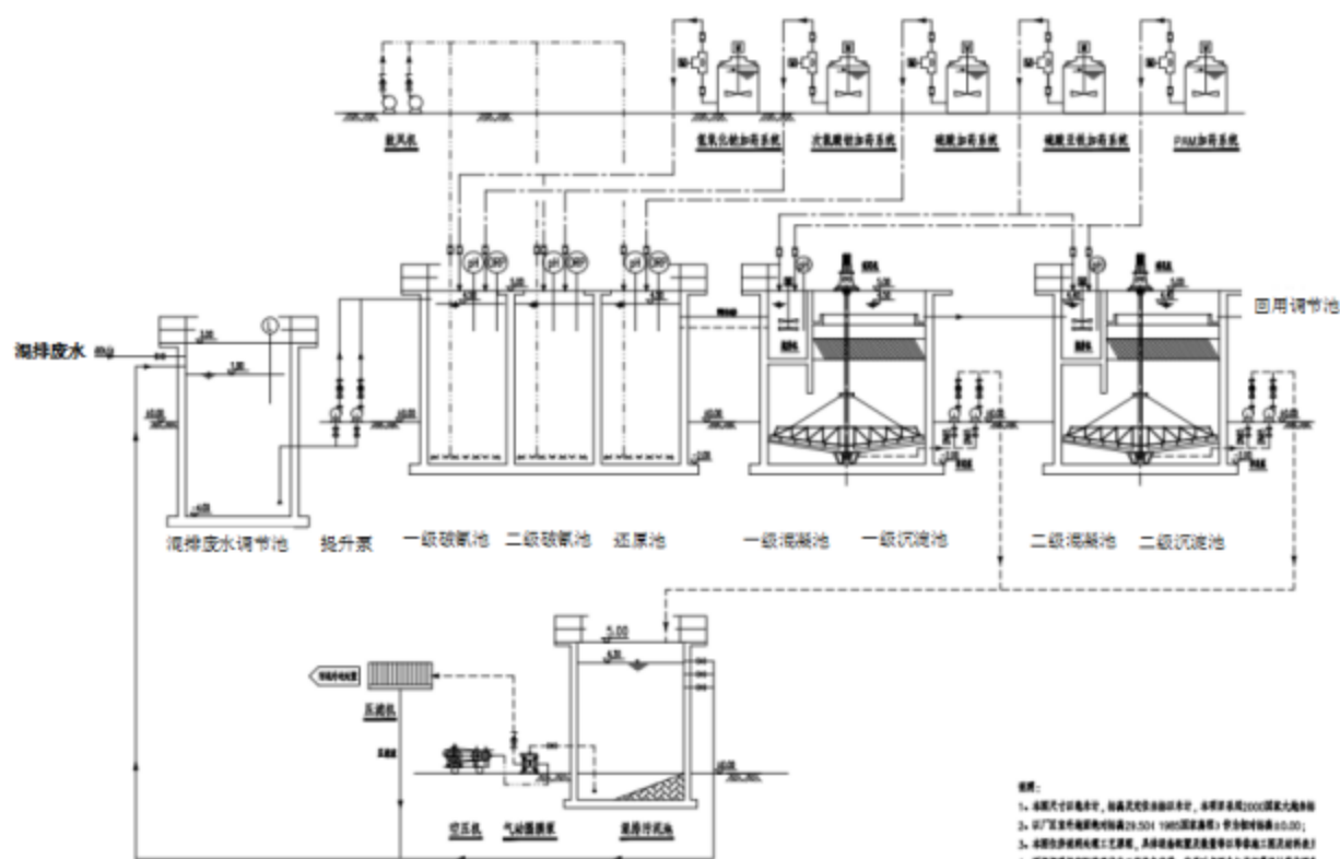
图 7.3-7 混排废水预处理工艺流程图
