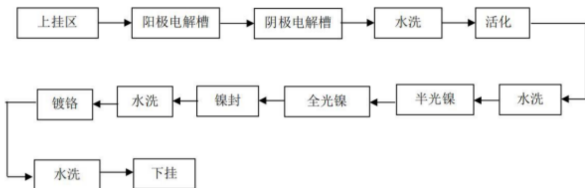
图 4.2-2 电镀生产线工艺流程图
