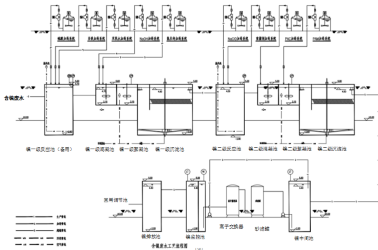
图 7.3-4 含镍废水预处理工艺流程图
