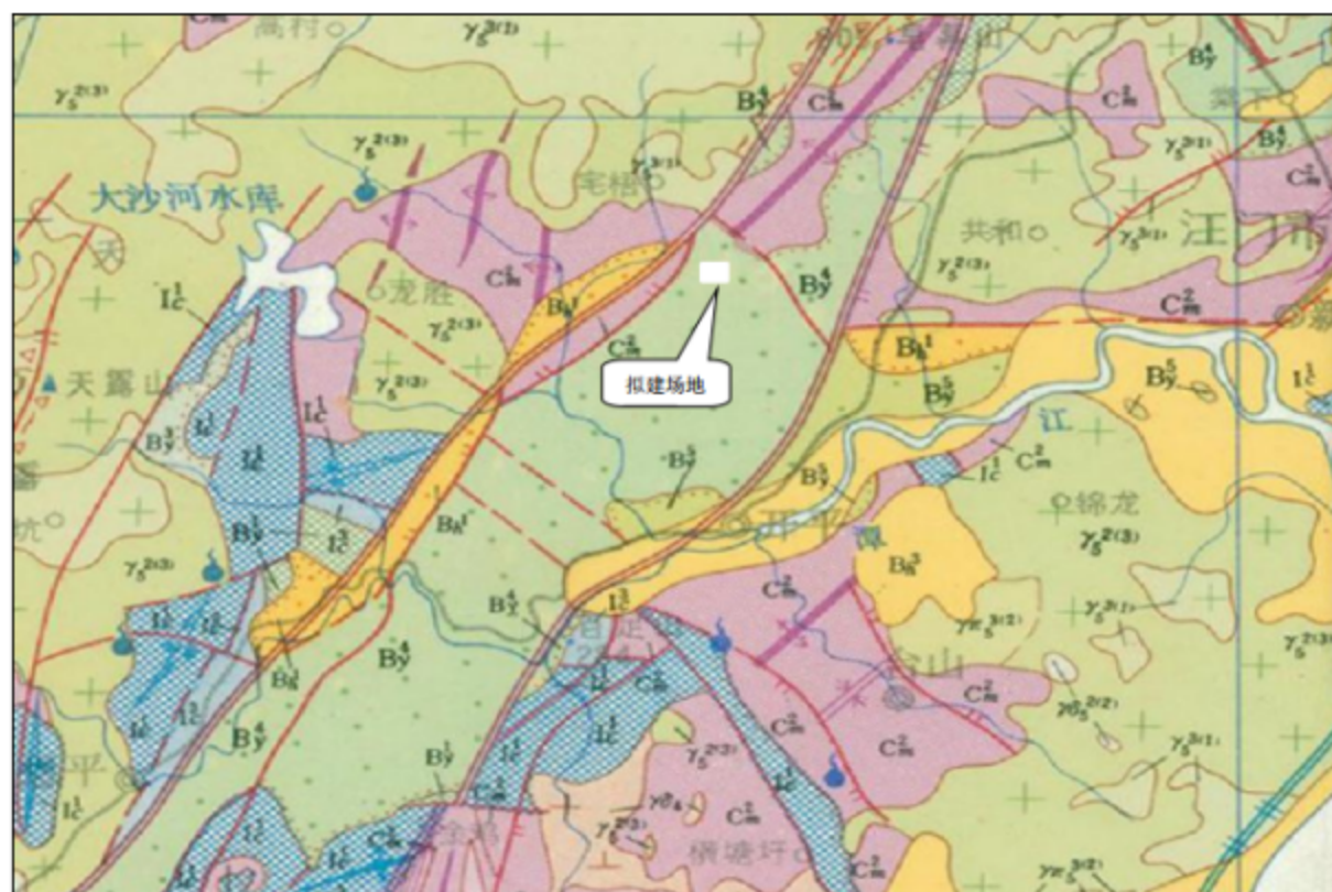
图 7.4-1 地质构造纲要图
