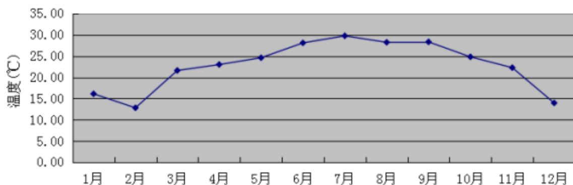
图 7.2-12 项目所在区域 2022 年平均温度月变化图
