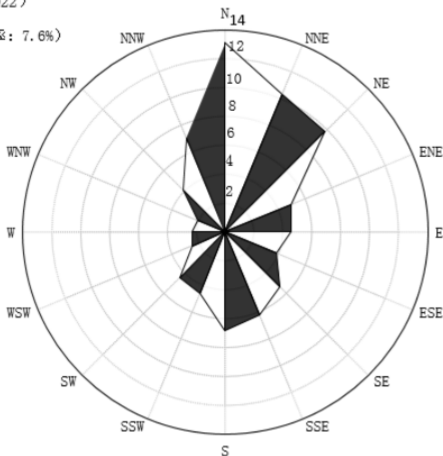
图 7.2-1 开平近 20 年风向玫瑰图 (统计年限: 2003-2022 年)
