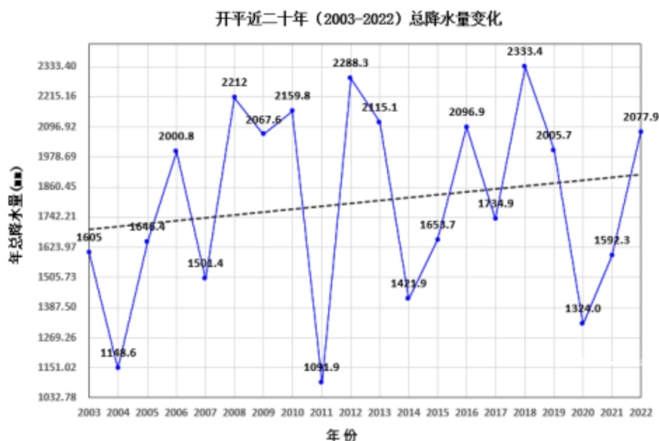
图 7.2-7 开平 (2003-2022) 年总降水量 (单位: 毫米)
