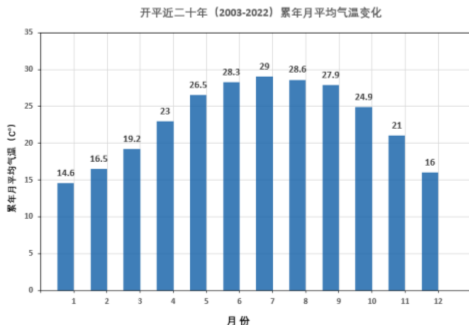
图 7.2-4 开平 (2003-2022) 月平均气温统计情况
