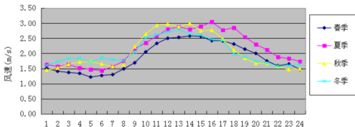
图 7.2-14 项目所在地 2022 年季小时平均风速的日变化图
