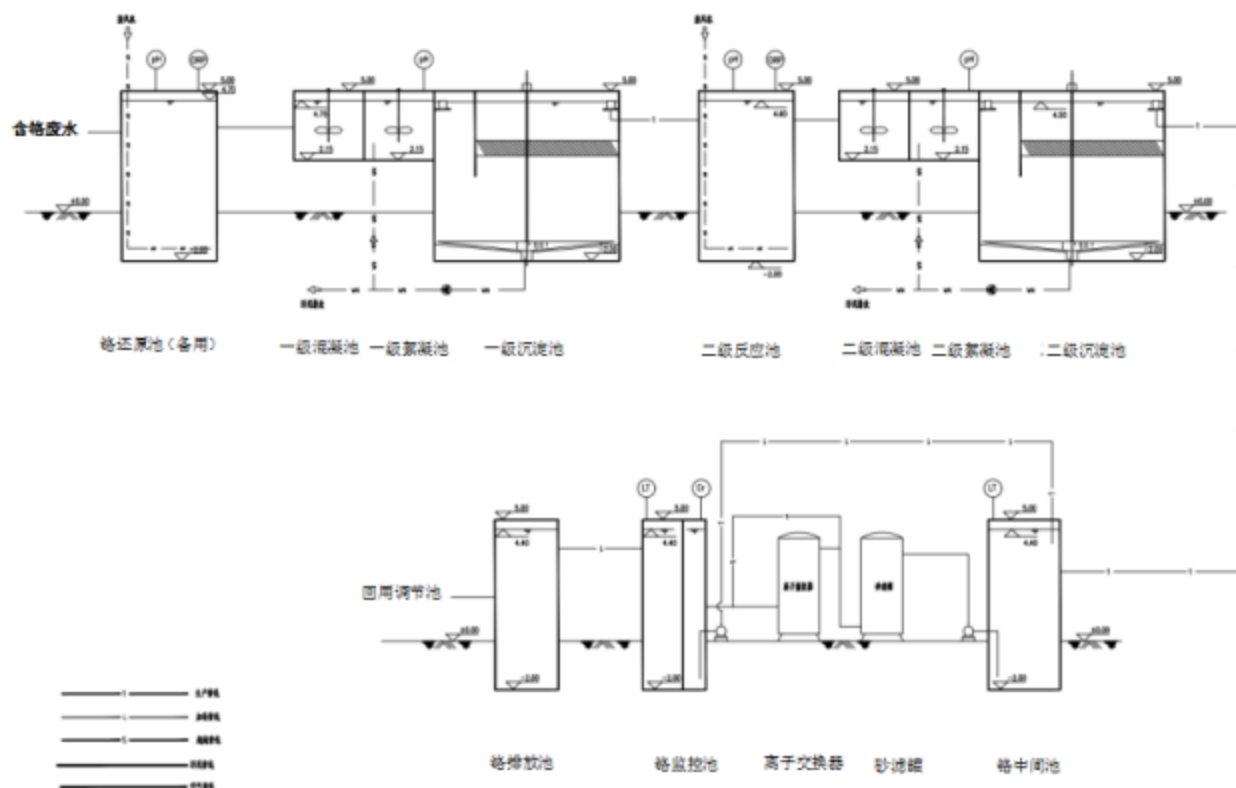
图 7.3-5 含铬废水预处理工艺流程图
