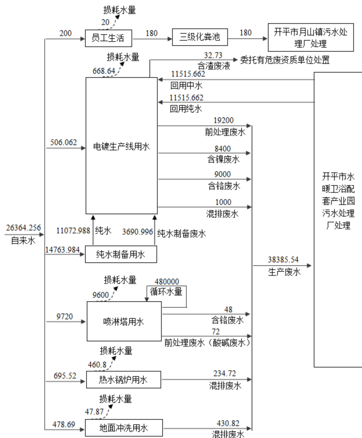
图 5.1-5 项目水平衡图 (单位: \text{m}^3/\text{a} )
