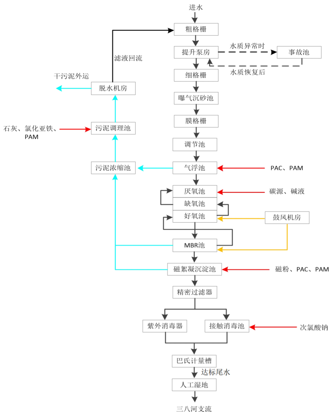
图 3.3-1 污水处理工程工艺流程图
