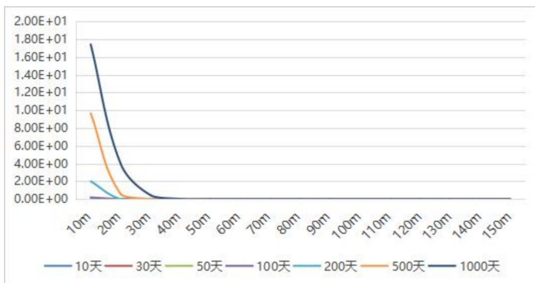
图 5.4-2 NH 3 -N 污染物连续渗漏预测统计图
