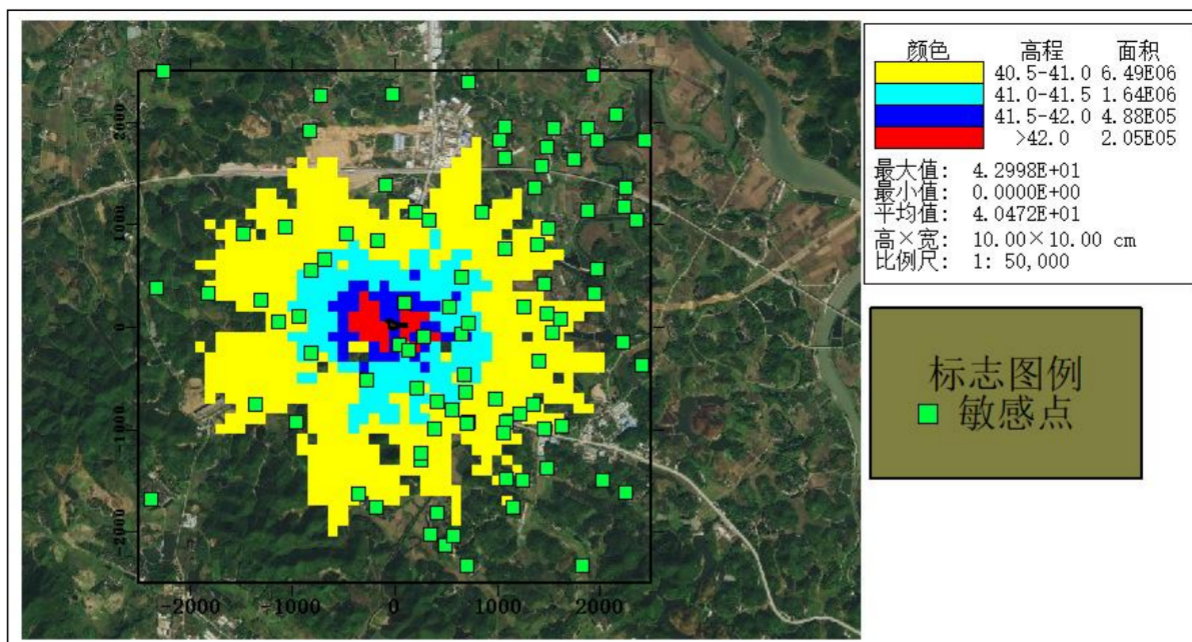
图 5.3-19 本项目 \text{NH}_3 叠加浓度预测结果图
