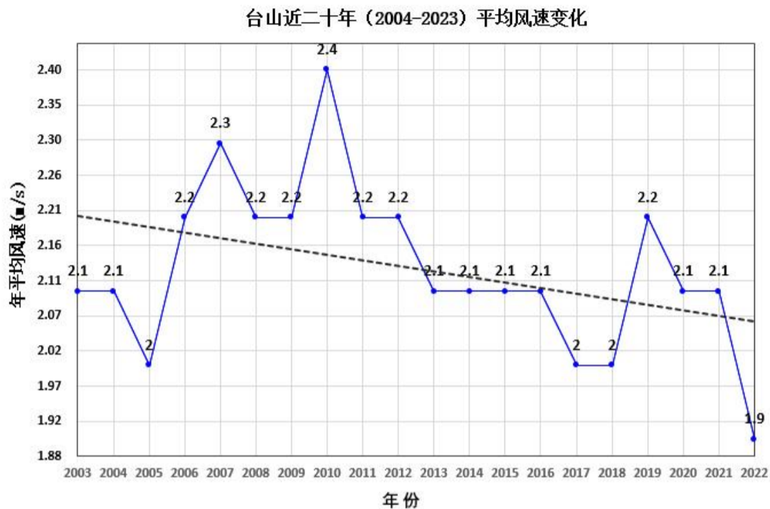
图 5.3-3 台山近二十年（2004-2023）平均风速变化（单位：m/s，虚线为趋势线）
