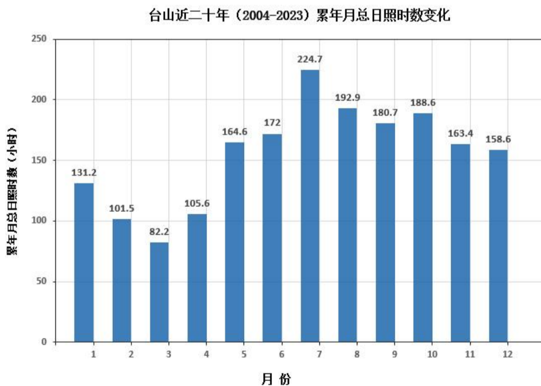
图 5.3-8 台山近二十年（2004-2023）累年月总日照时数变化（单位：小时）
