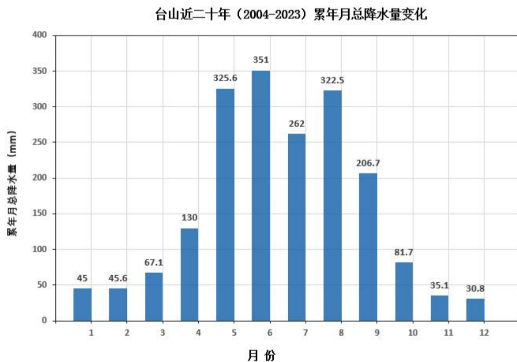
图 5.3-6 台山近二十年（2004-2023）累年月总降水量变化（单位：mm）
