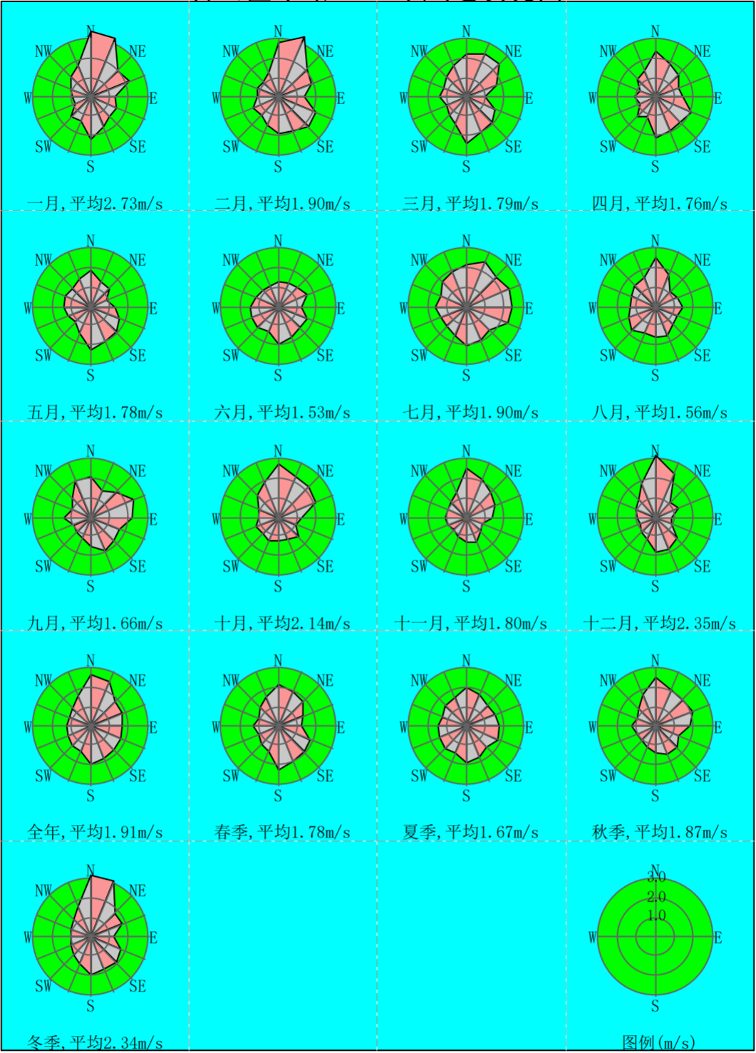
台山基本站2023年风速玫瑰图
