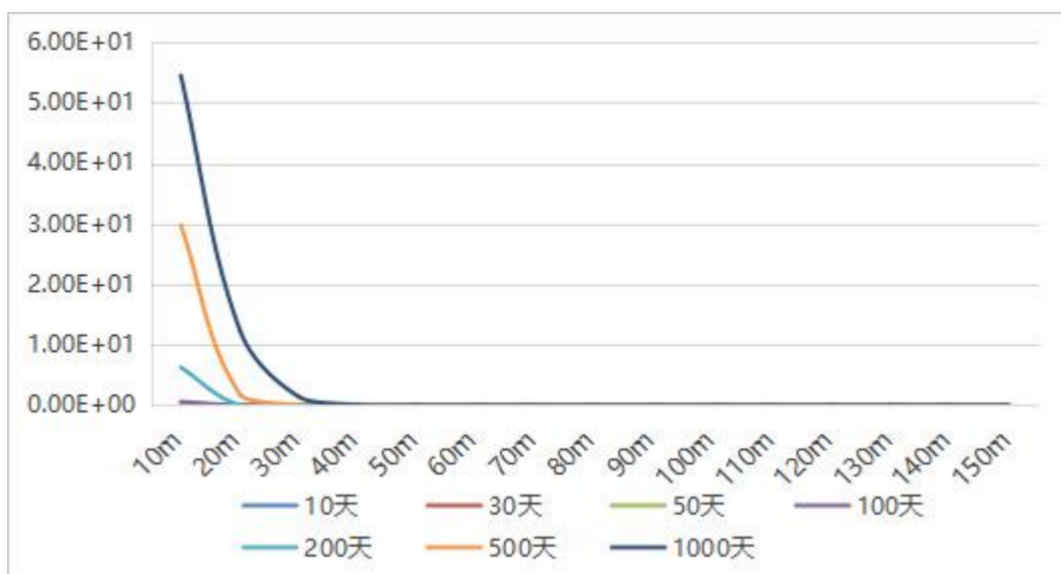
图5.4-1 COD Mn 污染物连续渗漏预测统计图
