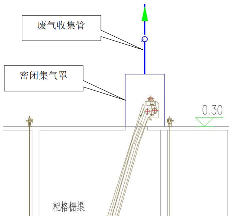
图 3.4-3 粗格栅、细格栅和提升泵房废气收集示意图
