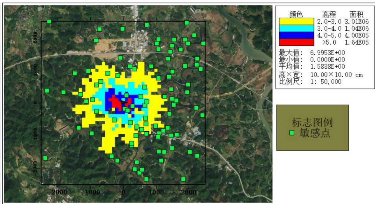
图 5.3-20 本项目 H 2 S 叠加浓度预测结果图
