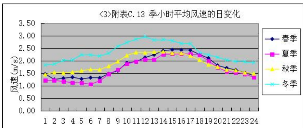
图 5.3-14 2023 年台山季小时平均风速日变化
