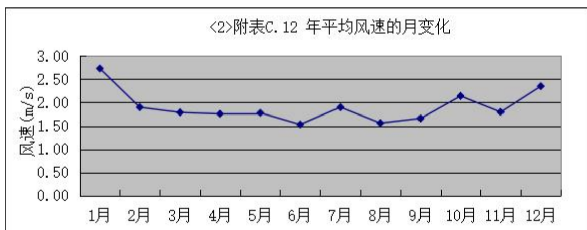
图 5.3-13 2023 年台山平均风速月变化曲线
