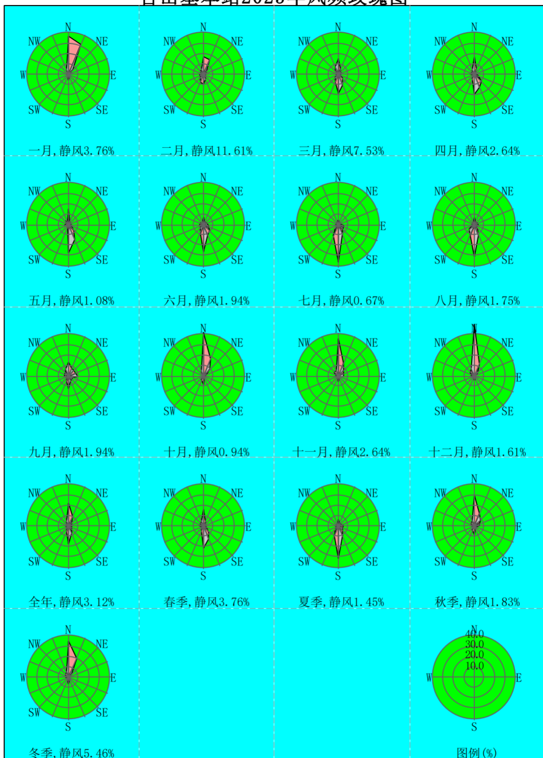
台山基本站2023年风频玫瑰图
