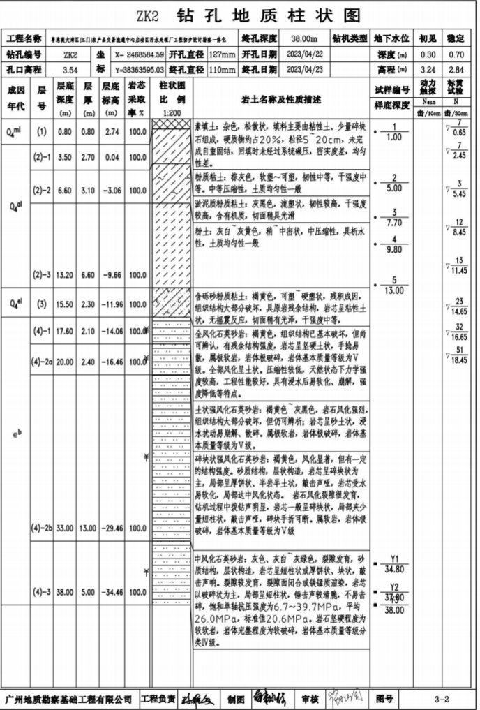
图 4.6-1 项目典型钻孔地质柱状图
