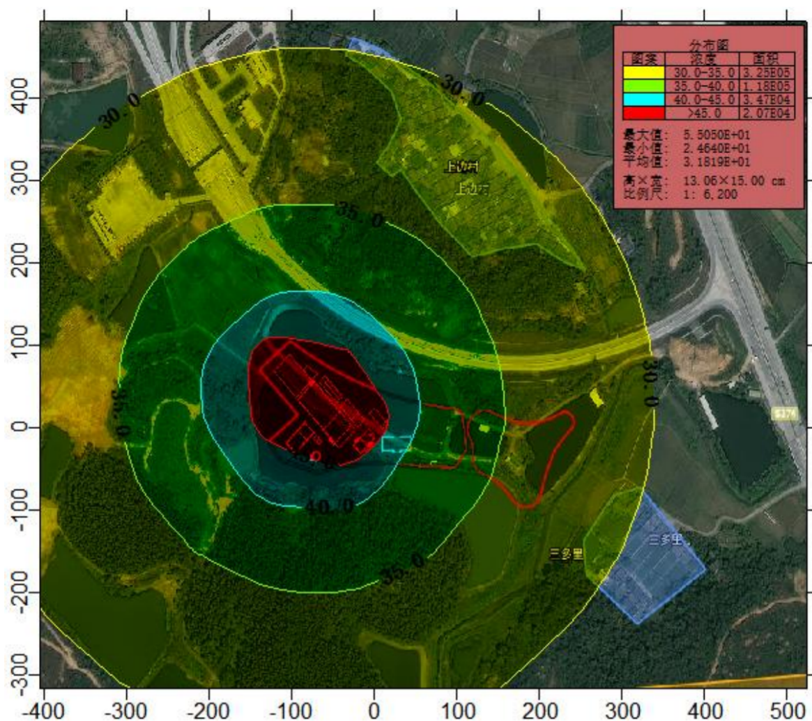
图 5.5-1 项目等声级线图
