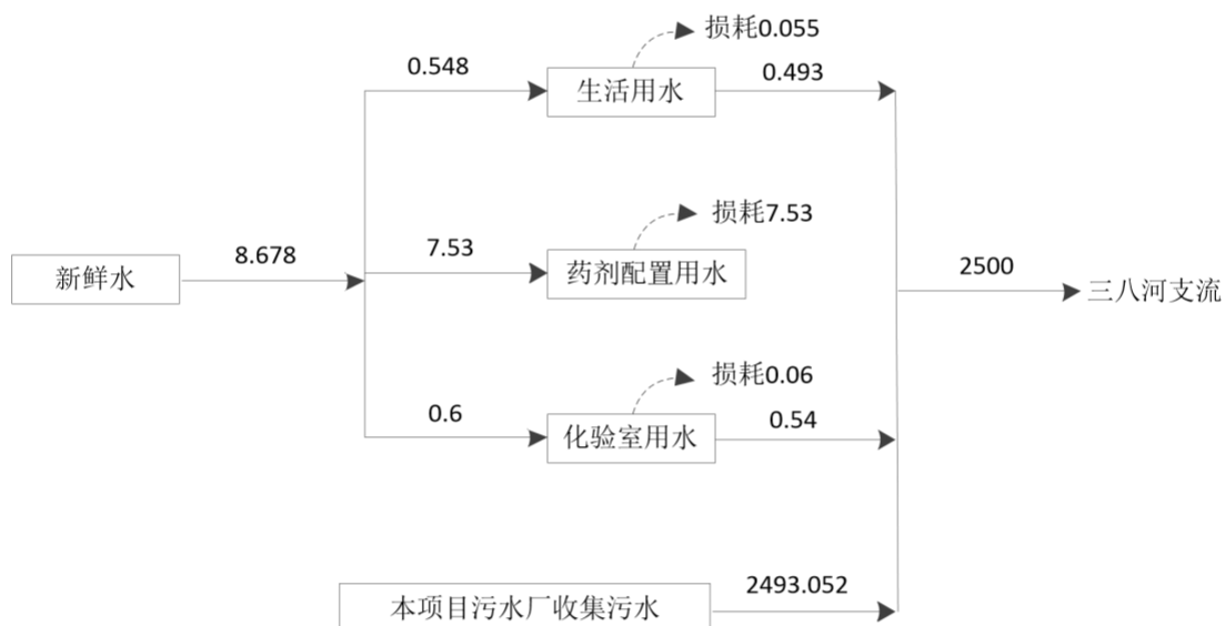
图 3.1-7 项目雨天水平衡一览表 单位: \text{m}^3/\text{d}
