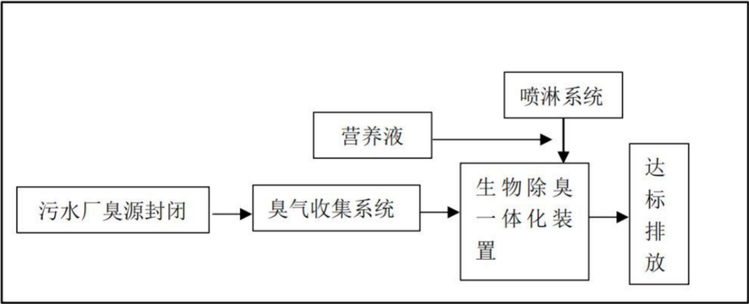
图 6.3-1 项目废气治理工艺流程图
