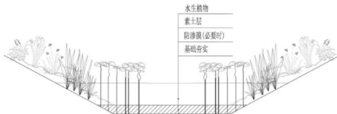
图 3.3-1 表面流人工湿地剖面示意图
