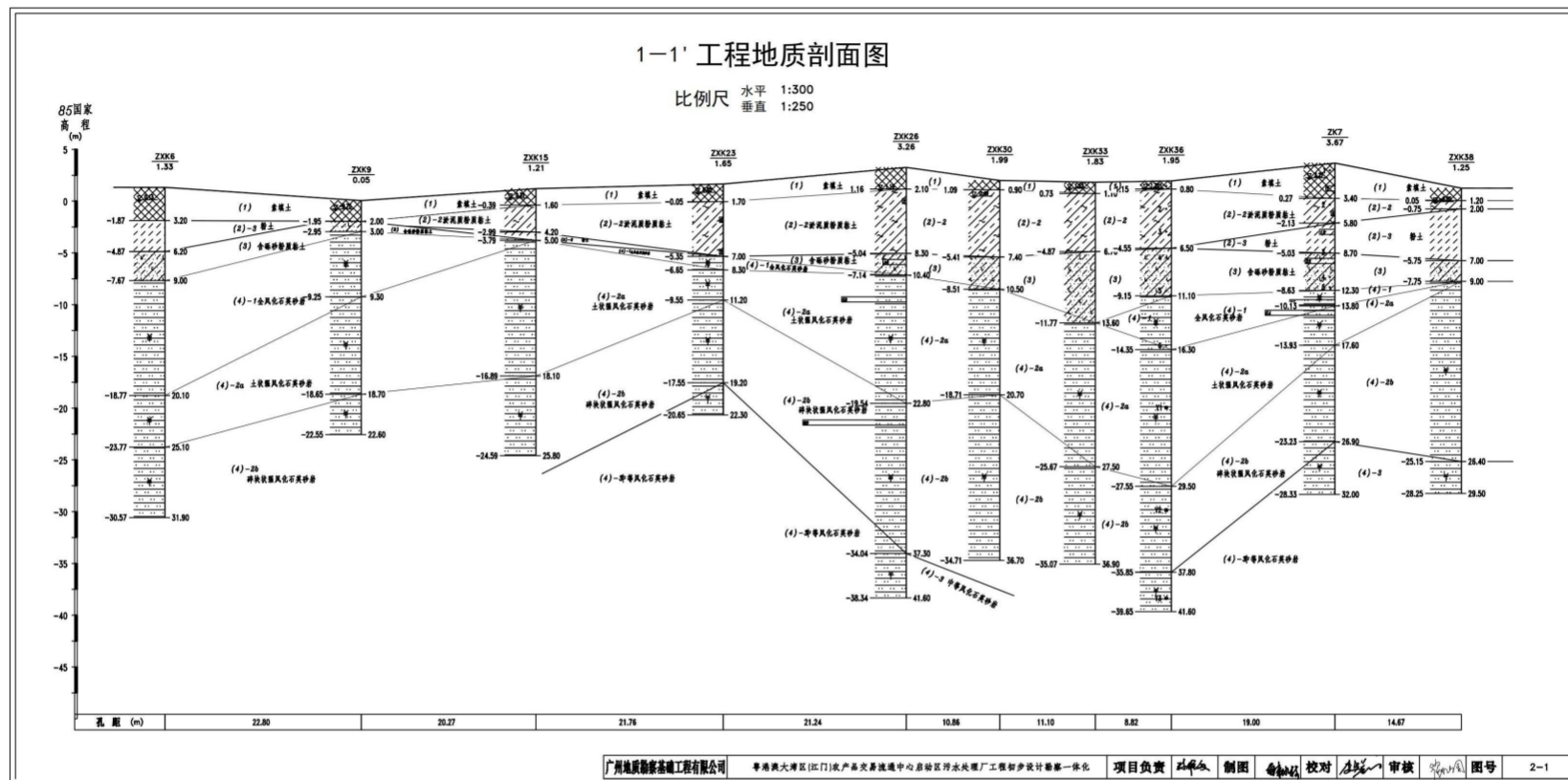
图 4.6-2 项目典型工程地质剖面图
