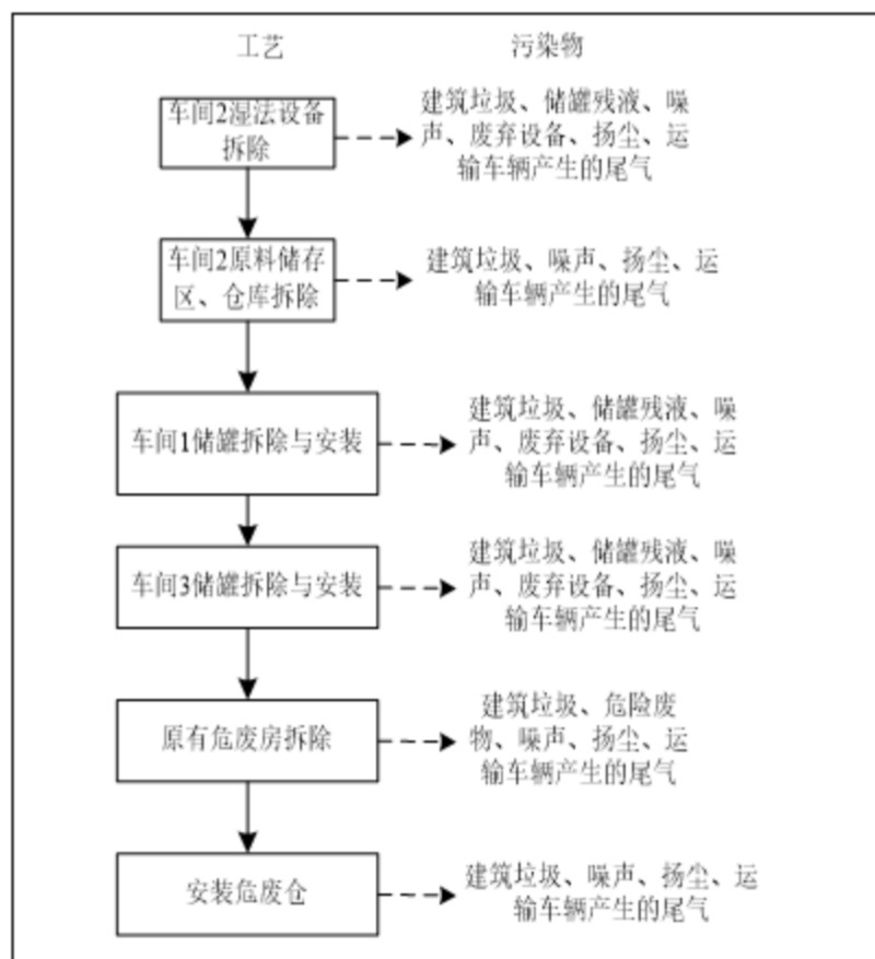
图 7.1-1 拆除以及新建施工工艺图
