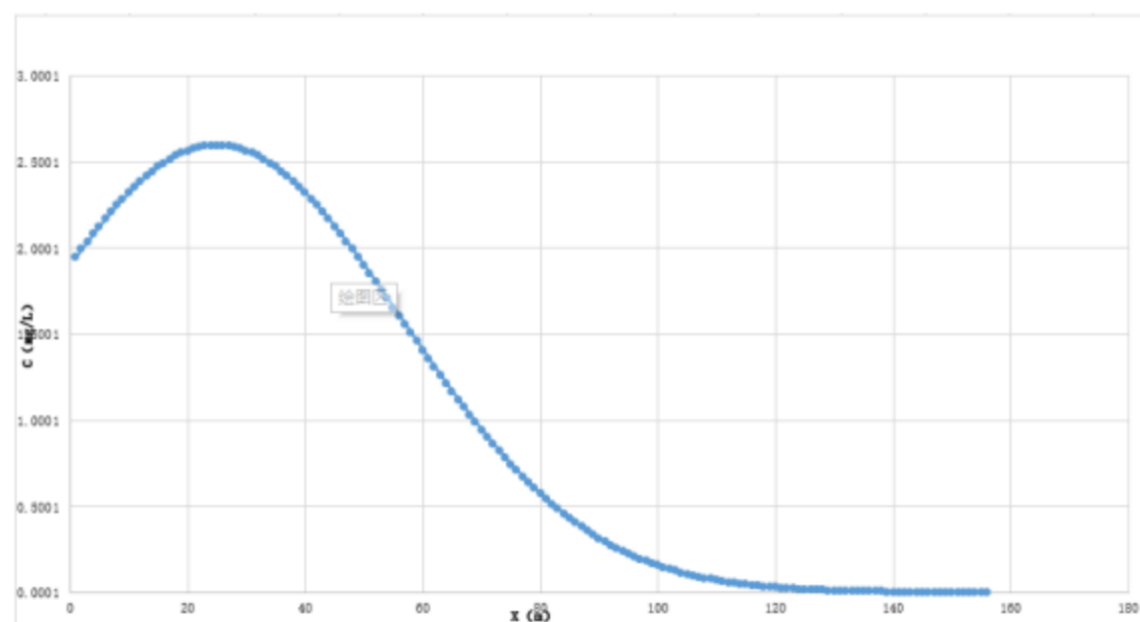
图 7.2-28 污水池渗漏100d后, 下游不同距离的 \text{COD}_{\text{Mn}} 浓度分布
