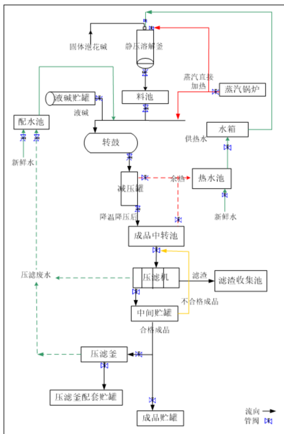
图 4.3-2 改扩建项目硅酸钠生产设备连接图
