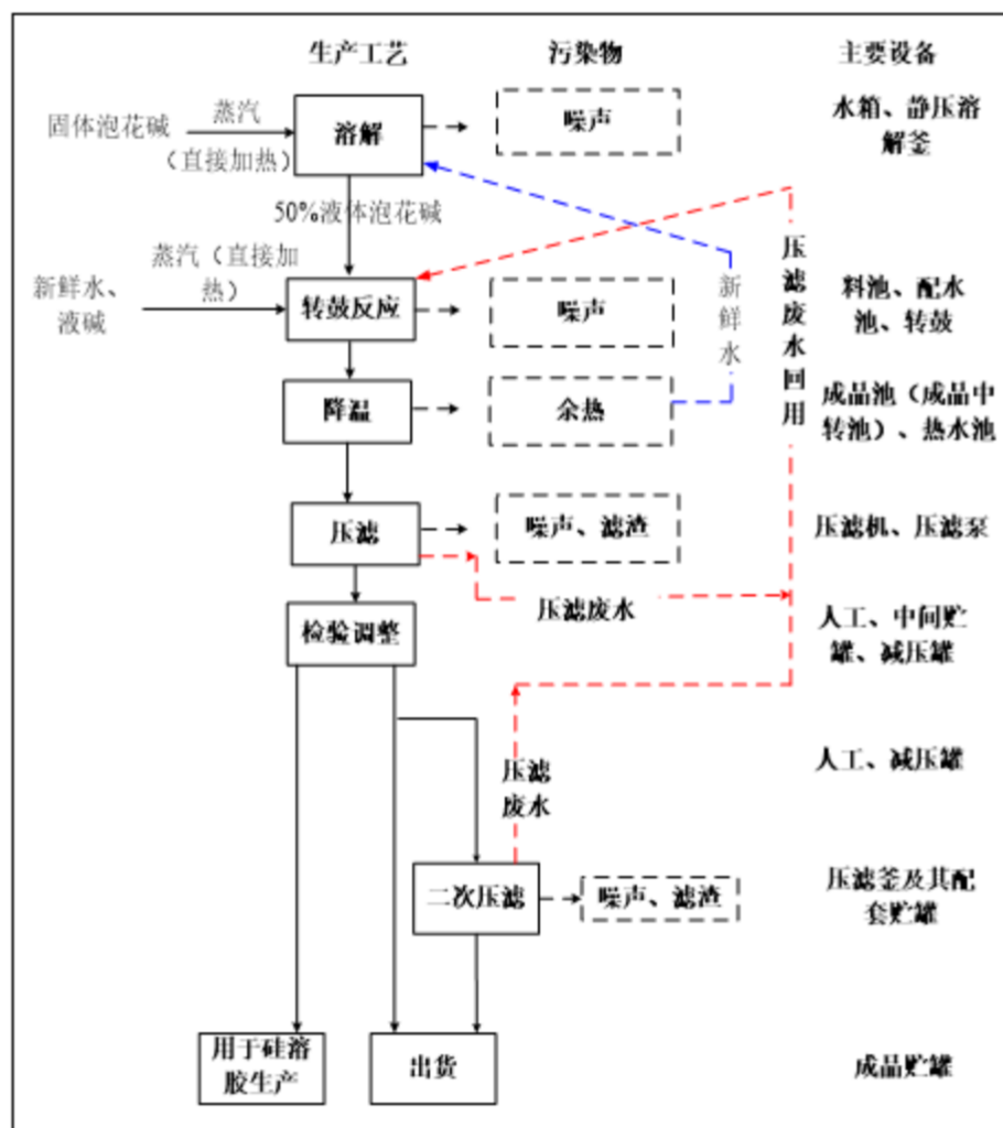
图 4.3-1 改扩建项目硅酸钠生产工艺流程及产污环节
