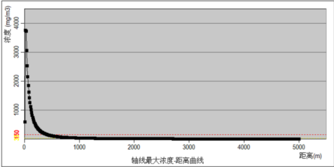
图 7.2-36 下风向不同距离处氯化氢的最大浓度（最不利气象条件）
