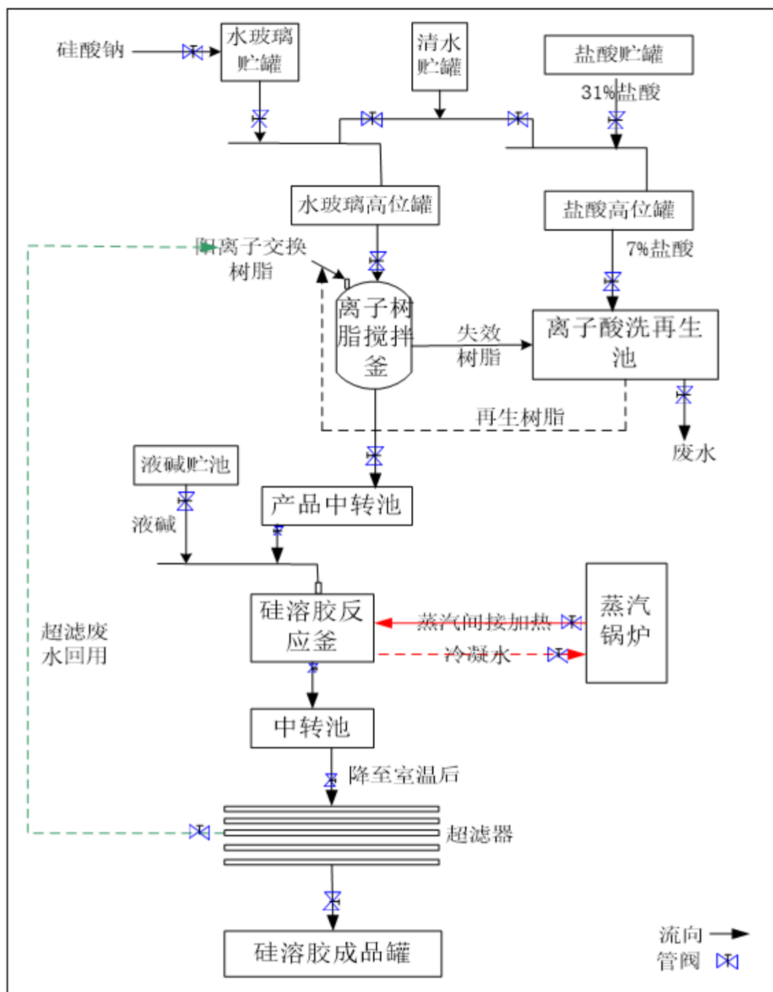
图 4.3-4 改扩建项目硅溶胶生产设备连接图
