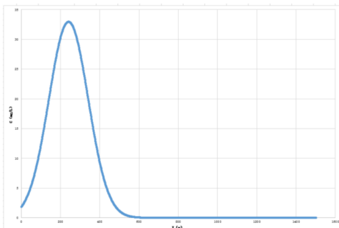
图 7.2-33 储罐渗漏10000d后，下游不同距离的氯化物浓度分布
