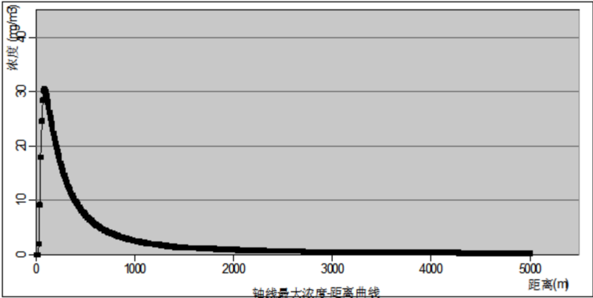
图 7.2-38 下风向不同距离处一氧化碳的最大浓度（最不利气象条件）
