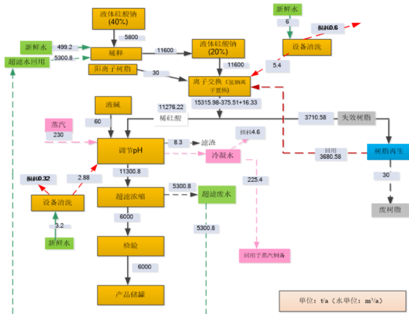
图 4.4-3 改扩建后项目全厂硅溶胶生产物料平衡
