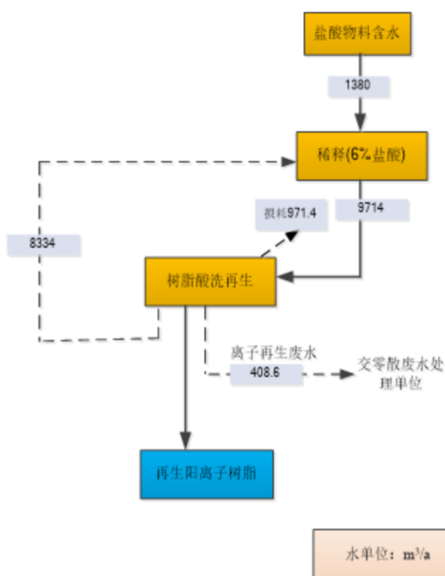
图 4.4-5 改扩建后项目全厂树脂再生盐酸平衡图
