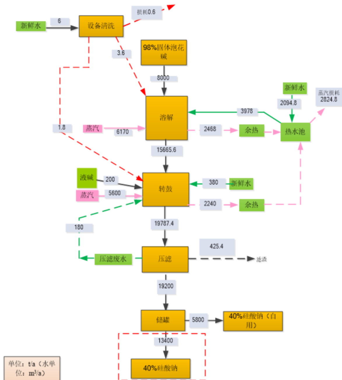
图 4.4-1 改扩建后项目全厂硅酸钠生产物料平衡
