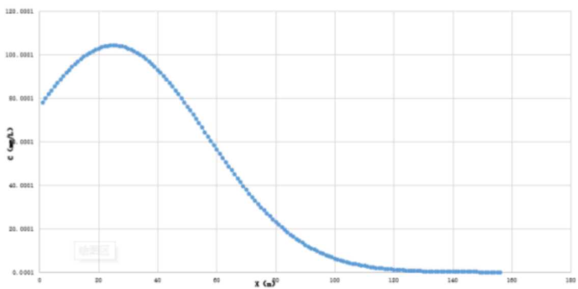
图 7.2-32 储罐渗漏1000d后，下游不同距离的氯化物浓度分布
