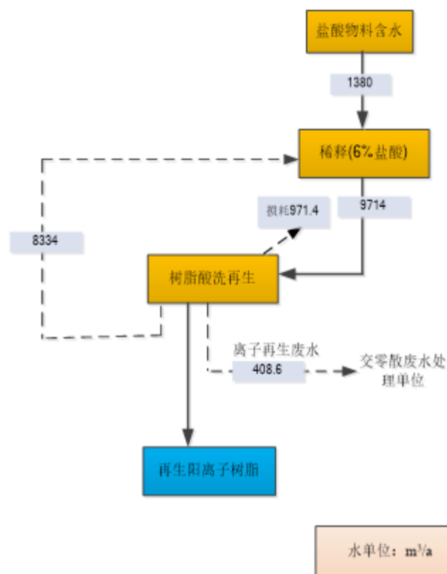
图 4.4-4 改扩建后项目全厂树脂再生水平衡图
