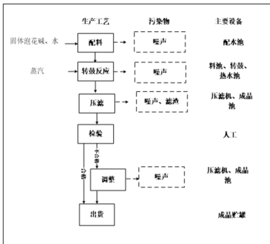
图 3.2-2 现有项目干法硅酸钠生产工艺流程及产污环节
