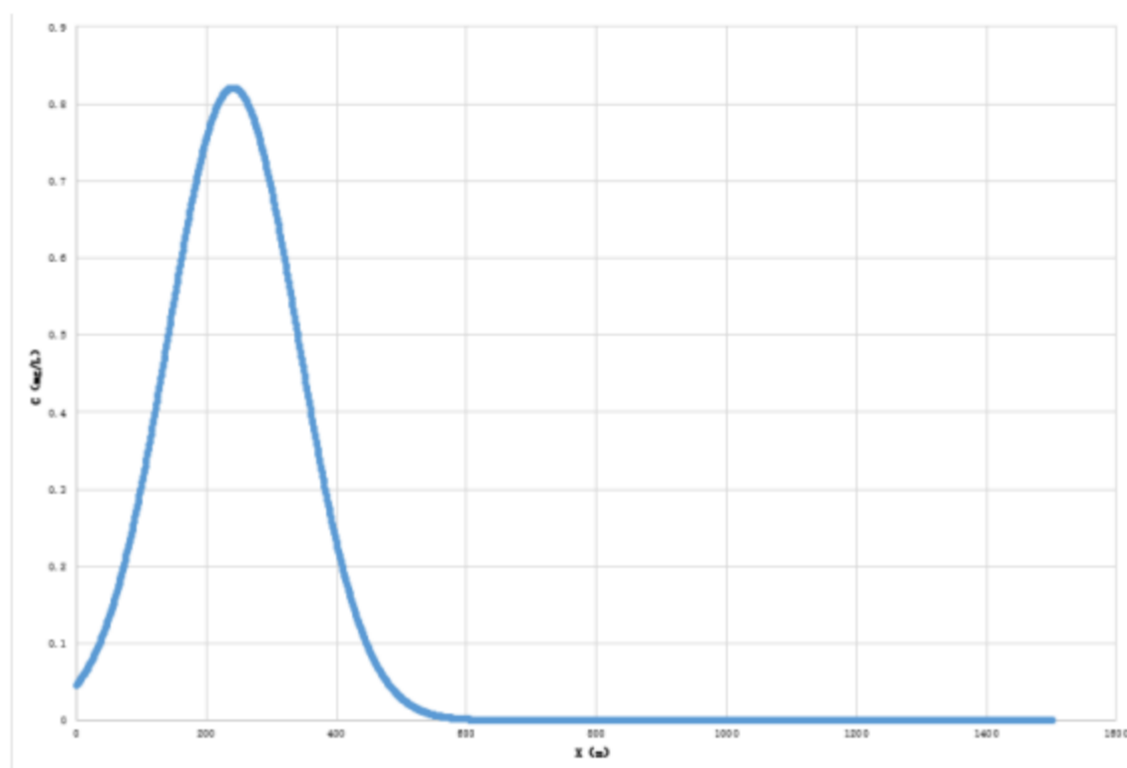
图 7.2-30 污水池渗漏10000d后，下游不同距离的COD Mn 浓度分布
