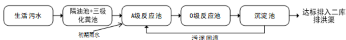
图 8.2-1 项目废水处理工艺流程图
