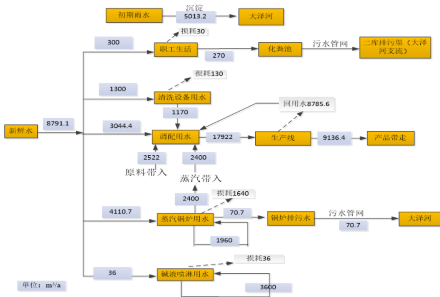
图 3.1-8 现有项目水平衡图
