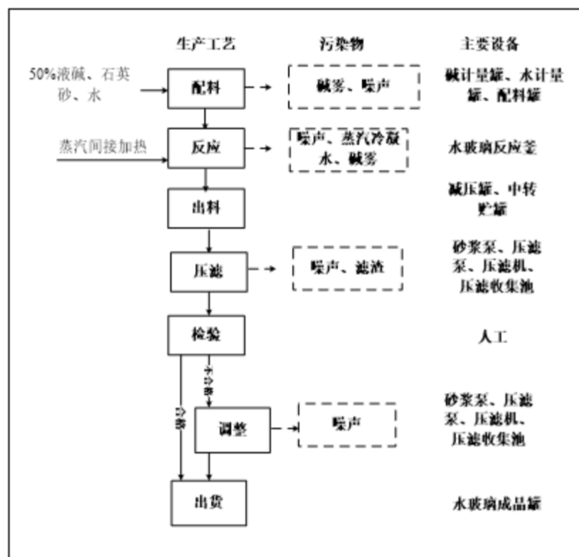
图 3.2-1 现有项目湿法硅酸钠生产工艺及产污环节图
