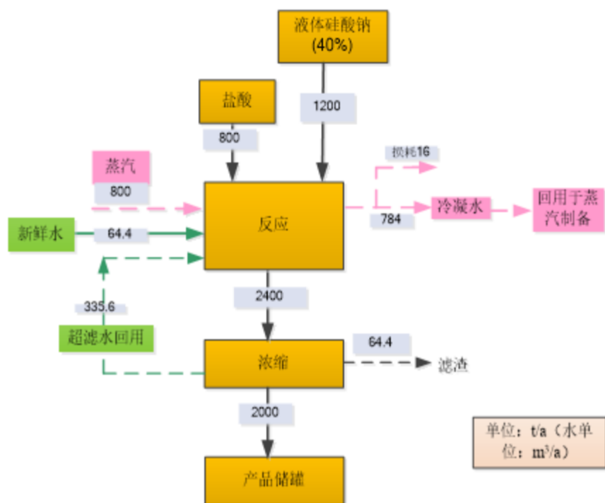
图 3.3-3 现有项目硅溶胶生产物料平衡
