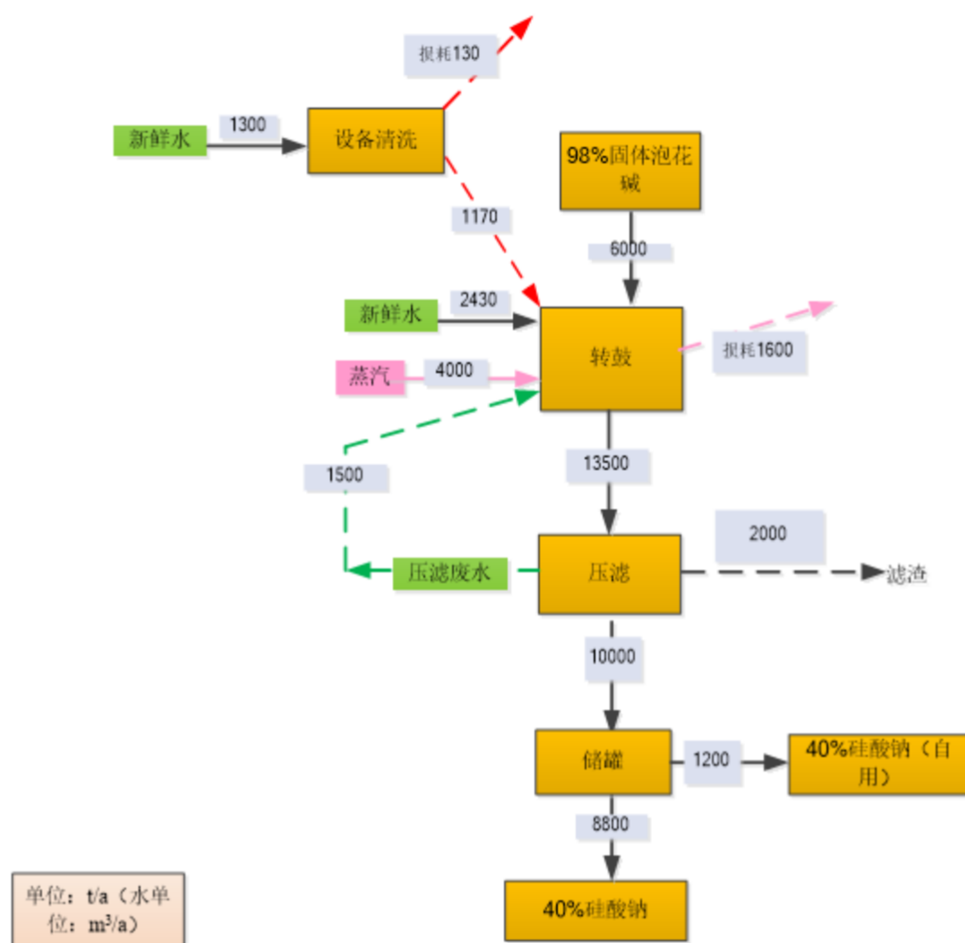
图 3.3-2 现有项目干法硅酸钠生产物料平衡
