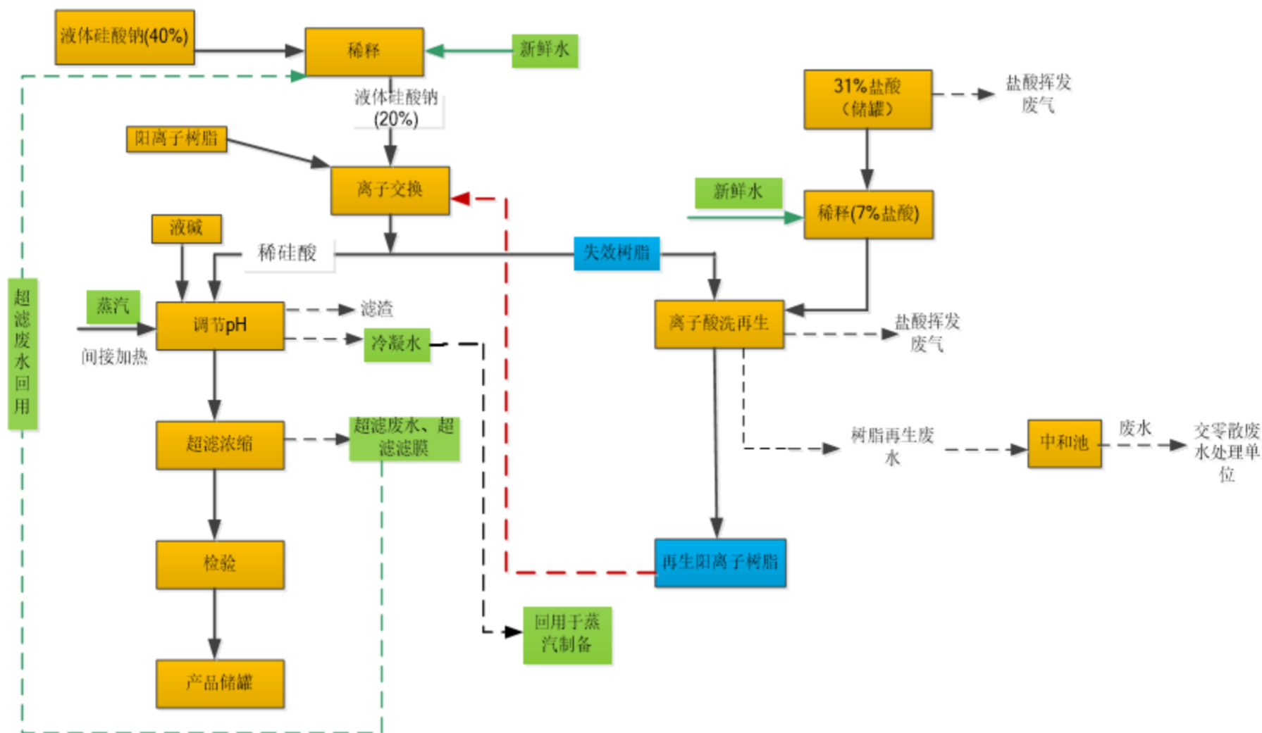
图 4.3-3 改扩建项目硅溶胶工艺流程及产污环节图
