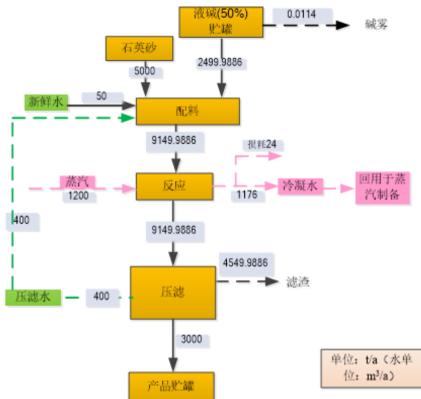
图 3.3-1 现有项目湿法硅酸钠生产物料平衡
