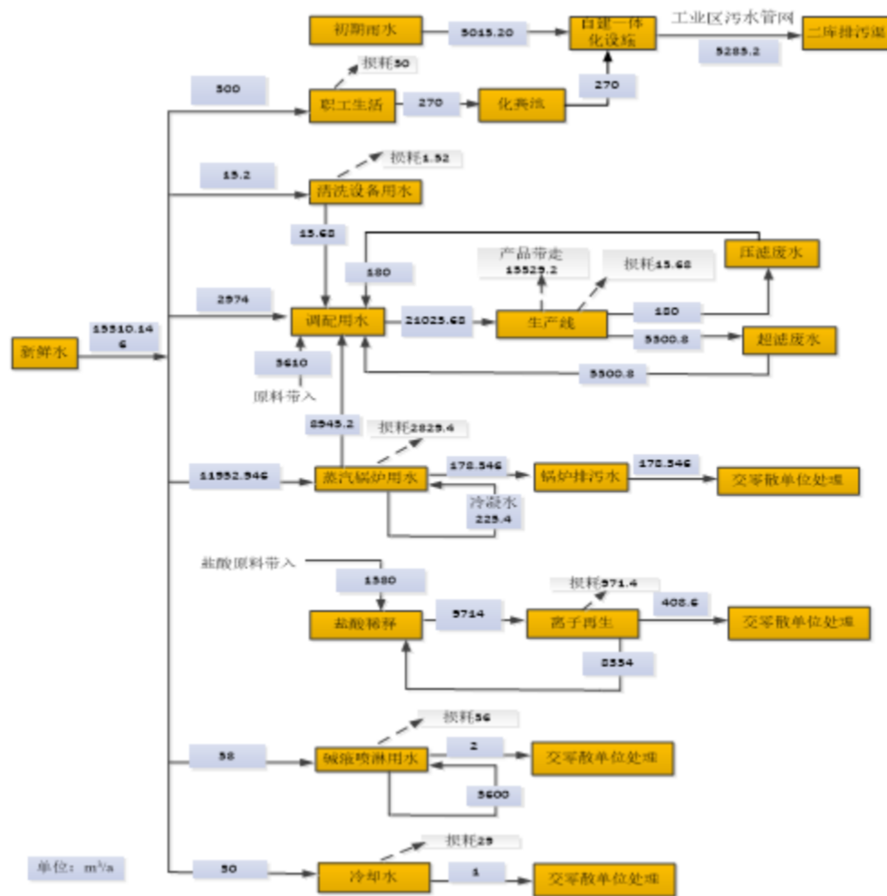
图 4.2-2 改扩建后全厂项目水平衡图
