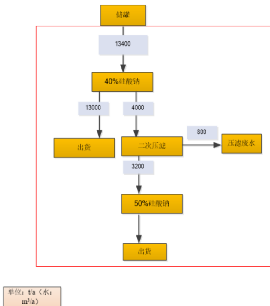
图 4.4-2 为图 4.4-1 红框部分物料细化图
