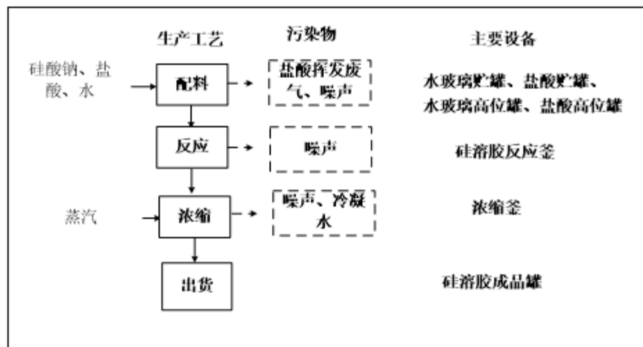
图 3.2-3 现有项目硅溶胶生产工艺流程及产污环节图
