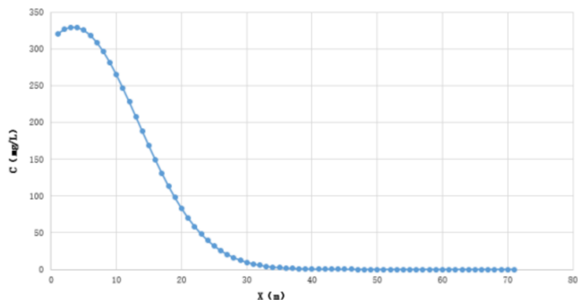
图 7.2-31 储罐渗漏100d后，下游不同距离的氯化物浓度分布
