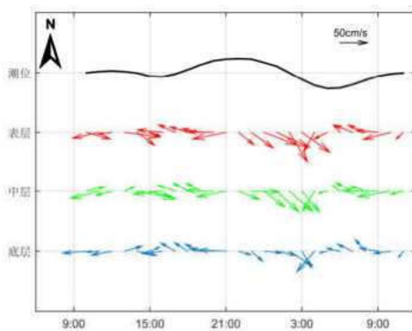
图 6.4-19 调查海域大潮 CL2 站实测海流矢量图
