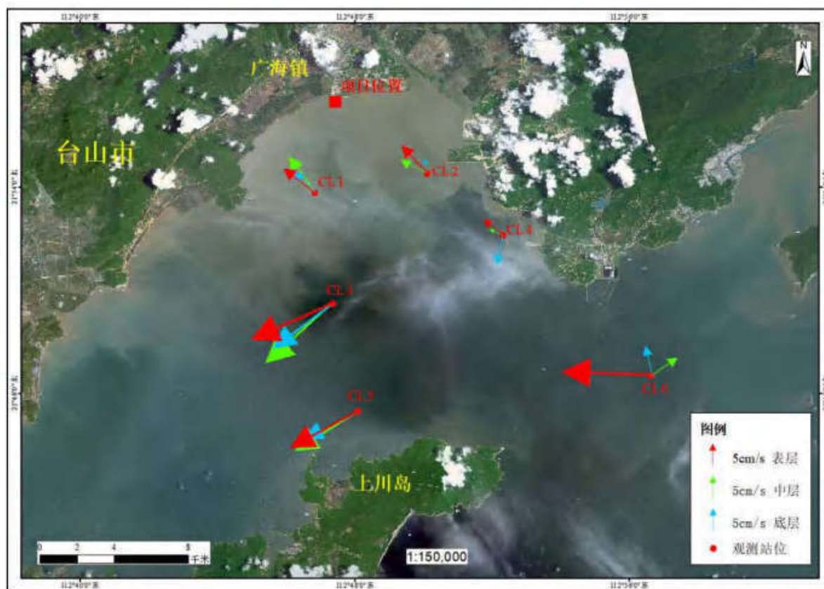
图 6.4-13 观测期间各站各层次余流图
