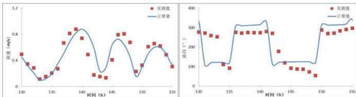
图 7.1-10 CL5 站流速、流向验证
