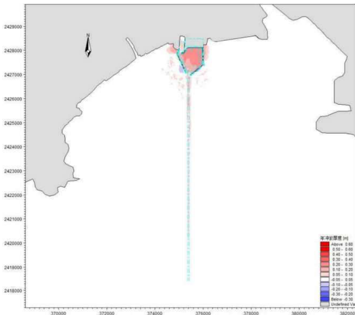
图 7.7-2 48 小时港池及航道骤淤量
