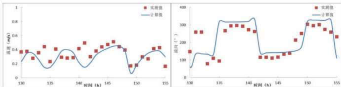
图 7.1-7 CL2 站流速、流向验证
