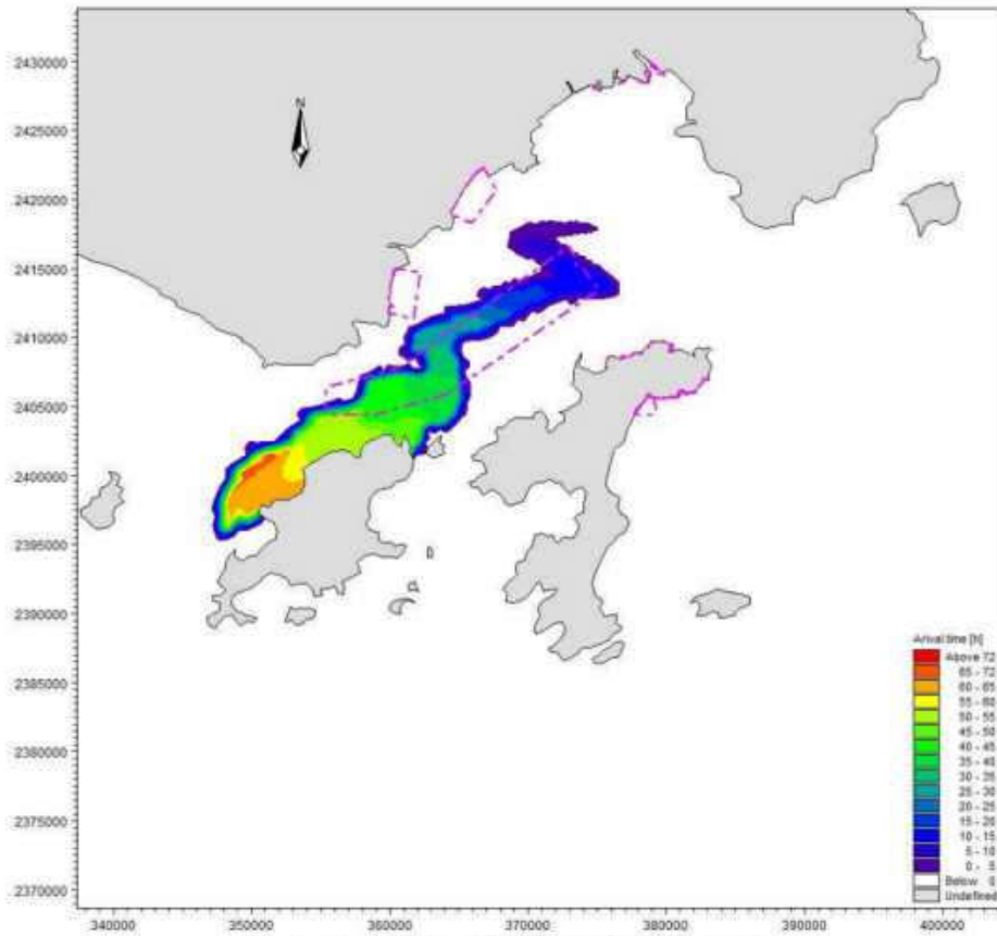
图 8.4-8 工况 7 溢油扫海范围 (72 时)
