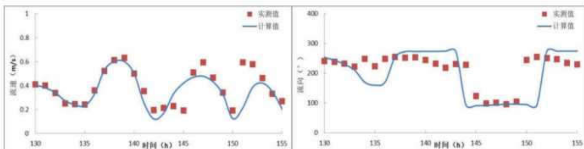
图 7.1-8 CL3 站流速、流向验证
