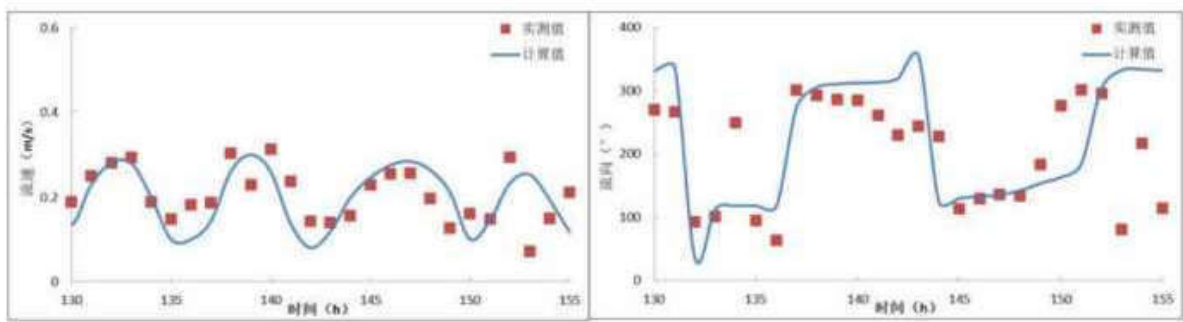
图 7.1-6 CL1 站流速、流向验证
