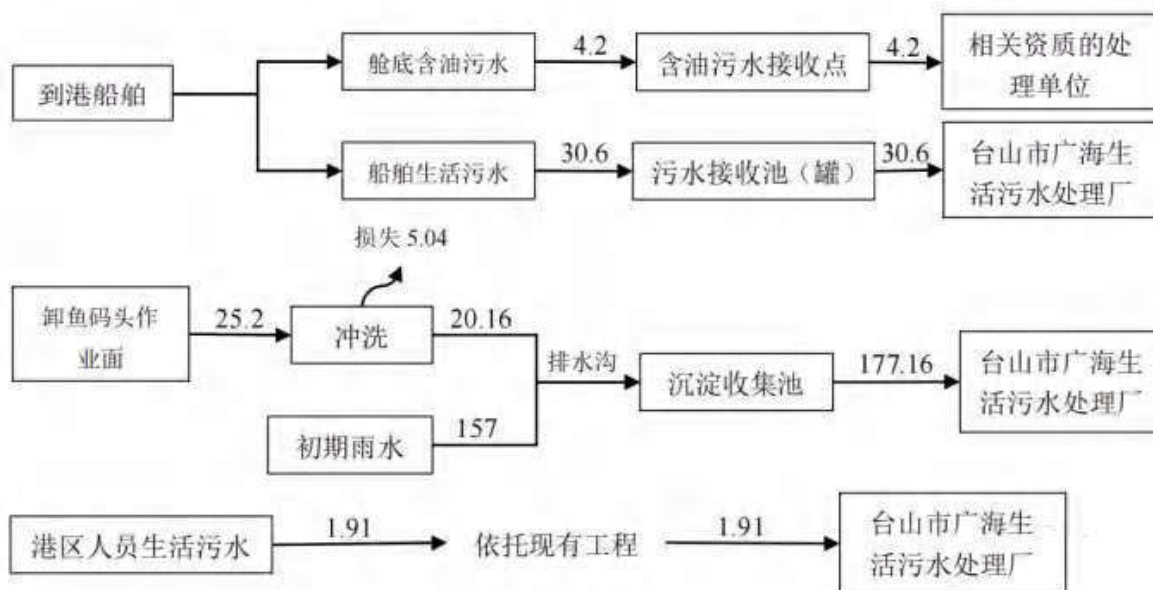
图 5.2-1 项目水平衡图（单位：t/d，初期雨水为 t/次）
