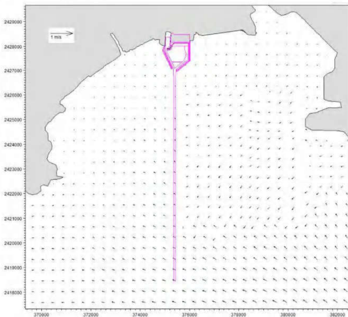
图 7.5-1 项目周边余流图
