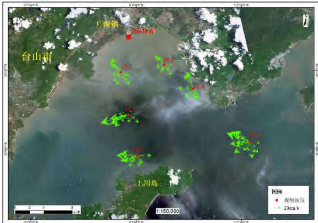
图 6.4-3 观测期间各站表层（0.2h）海流矢量图
