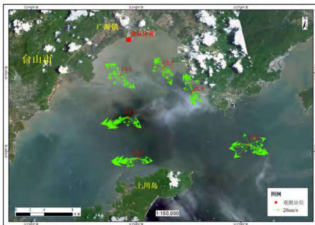
图 6.4-4 观测期间各站中层 (0.6h) 海流矢量图
