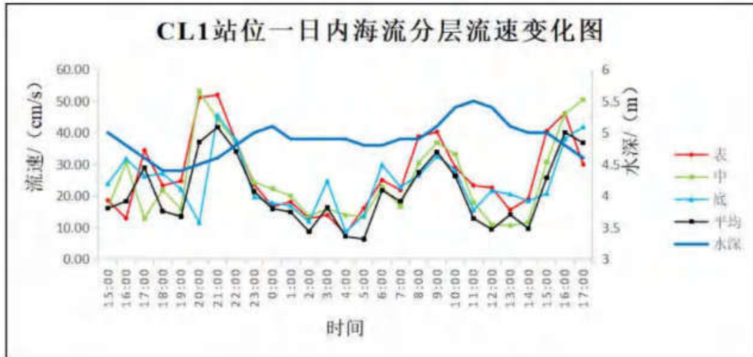
图 6.4-7 CL1 站位海流分层流速变化图
