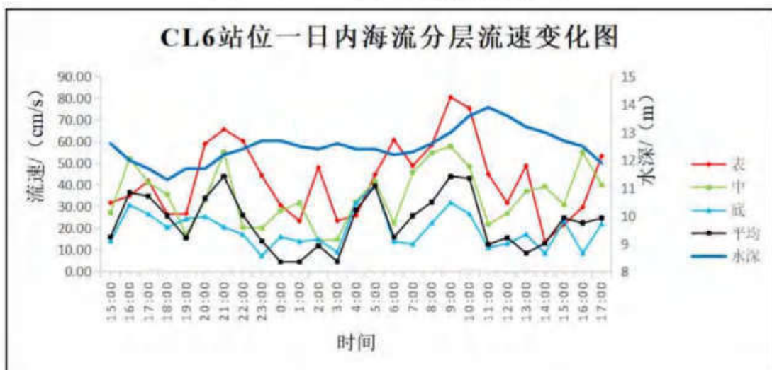
图 6.4-12 CL6 站位海流分层流速变化图
