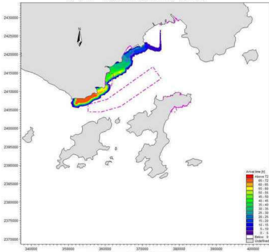
图 8.4-3 工况 2 溢油扫海范围 (72 时)
