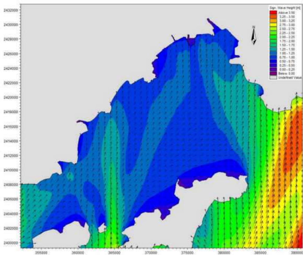
图 7.6-8 工程后 50 年一遇 SW 向波高分布图
