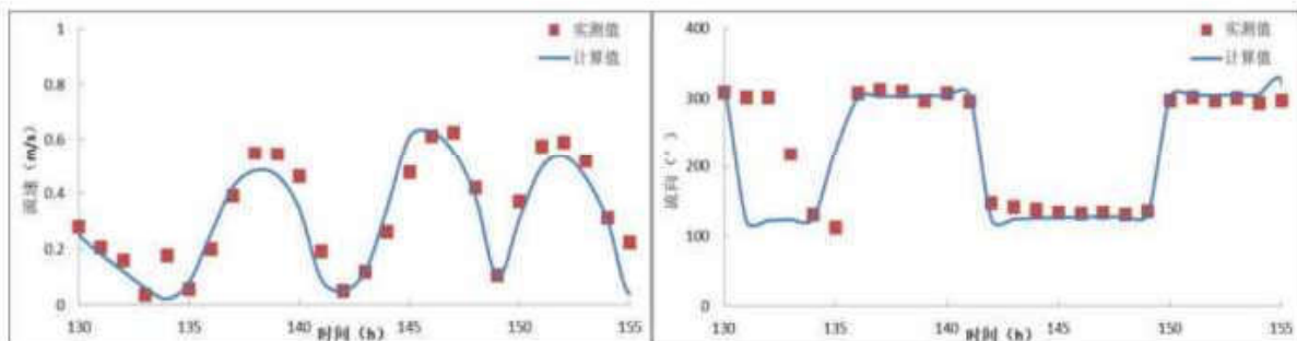
图 7.1-9 CL4 站流速、流向验证
