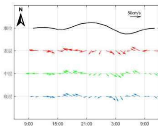
图 6.4-18 调查海域大潮 CL1 站实测海流矢量图
