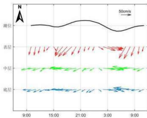
图 6.4-20 调查海域大潮 CL3 站实测海流矢量图
