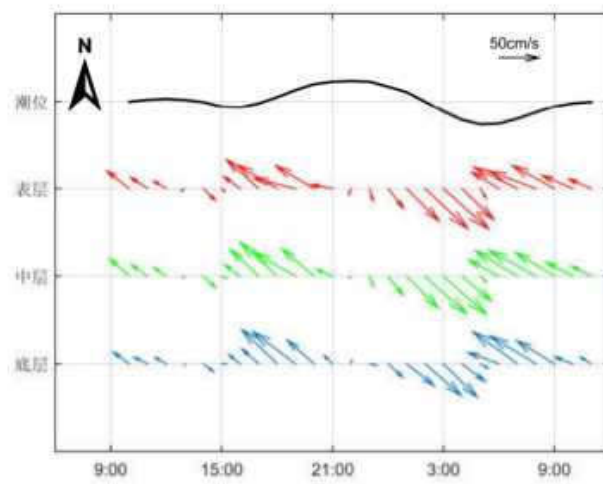
图 6.4-21 调查海域大潮 CL4 站实测海流矢量图
