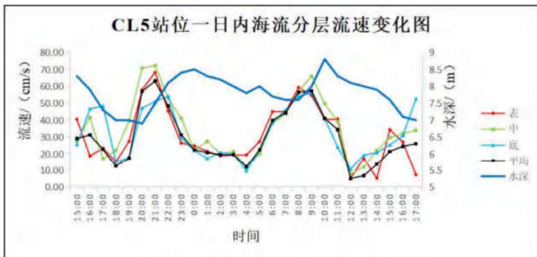
图 6.4-11 CL5 站位海流分层流速变化图
