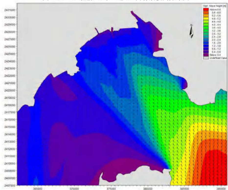
图 7.6-3 工程前 50 年一遇 SSE 向有效波高分布图
