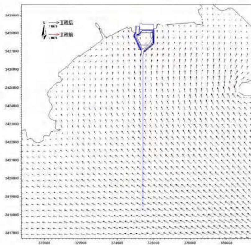
图 7.1-18 工程前后涨急流场叠加图
