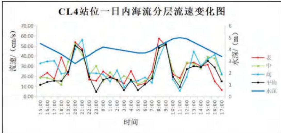
图 6.4-10 CL4 站位海流分层流速变化图
