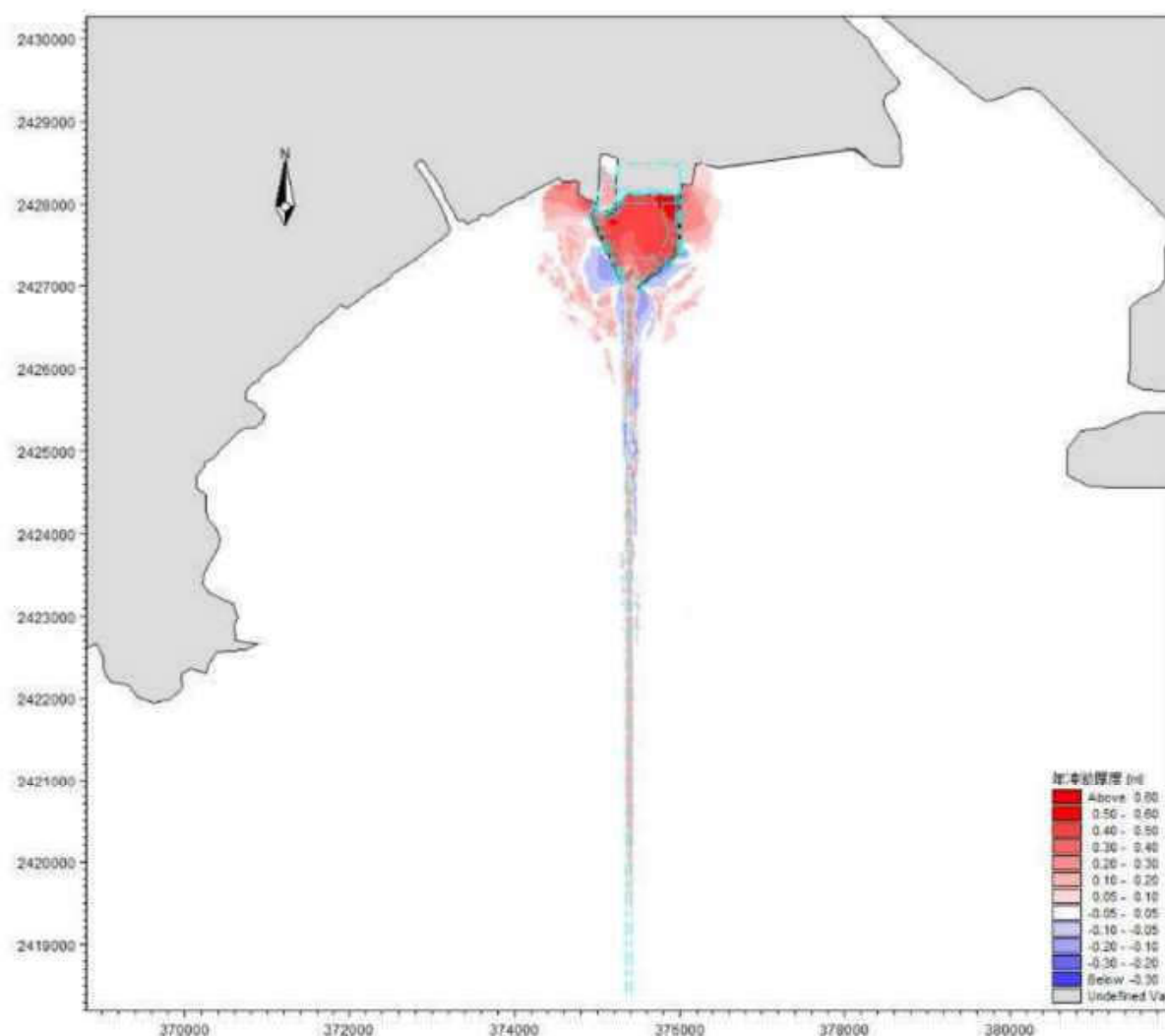
图 7.7-1 工程实施后年冲淤变化图
