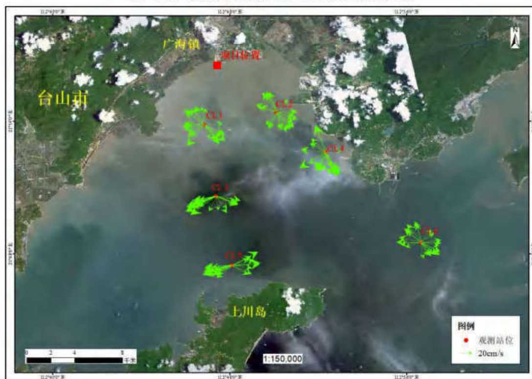
图 6.4-5 观测期间各站底层 (0.8h) 海流矢量图
