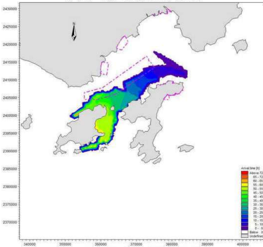
图 8.4-9 工况 8 溢油扫海范围 (72 时)
