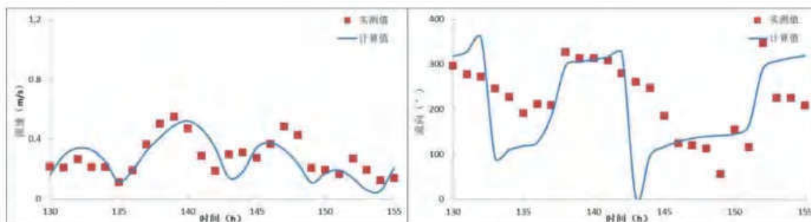
图 7.1-11 CL6 站流速、流向验证
