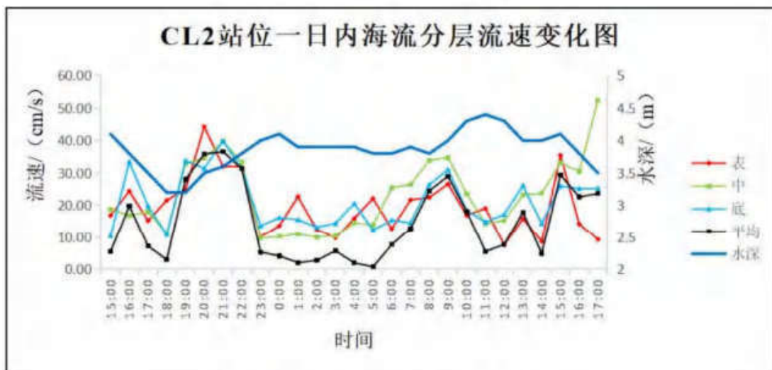
图 6.4-8 CL2 站位海流分层流速变化图
