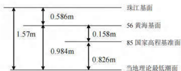
图 6.1-5 工程各基面换算关系示意图
